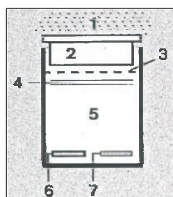
Abbildung 3: Prinzipskizze des elektrochemischen CO-Sensors – Schematic diagram of the electrochemical sensor.
