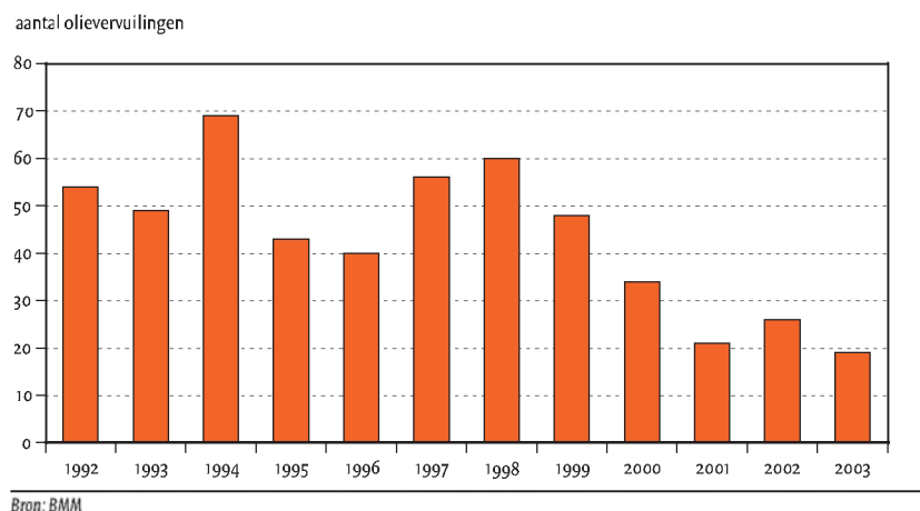
Figuur 8.4: Aantal operationele olieverontreinigingen geobserveerd door het toezichtvliegtuig (Belgisch gedeelte van de Noordzee en aangrenzende zone, 1992-2003)
