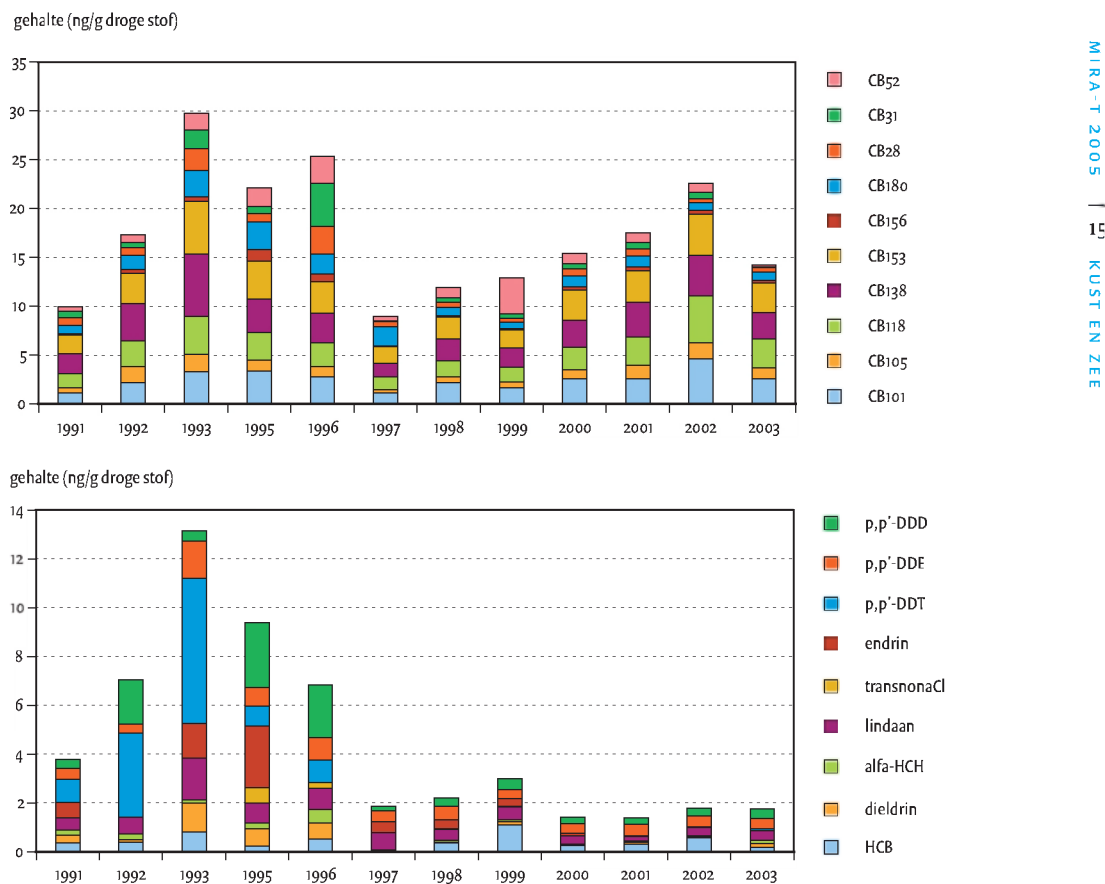
Figuur 8.2: Gehaltes aan PCB's* (boven) en OCP's (onder) in de fijne fractie (< 63 µm) van het sediment (Belgisch gedeelte van de Noordzee, 1991-2003)
