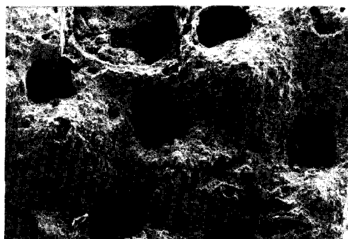
FIG. 16. — Umbonula megastoma (Busk, 1859). Saint-Sauveur-le-Vicomte, la Gathe (Manche), niveau 48-49,5 m. Pliocène inférieur. (R 62718 ; LP, MNHN). x 66.
