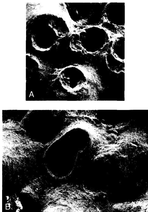
FIG. 31. — Turbicellepora coronopus (Wood, 1844). Saint-Sauveur-le-Vicomte, la Gathe (Manche), niveau 49,5-52 m. Pliocène inférieur. (R 62733 ; LP, MNHN). A, x 80. B, aviculaire interzoécial, x 100.
