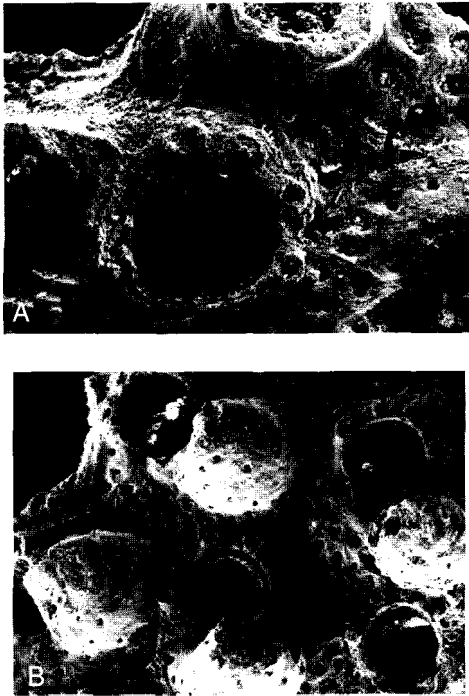
FIG. 35. — Ascophora incertae sedis. Remilly-sur-Lozon, l'Angle (Manche), niveau 19-20 m. Pliocène supérieur. (R 62725 ; LP, MNHN). A , ouverture avec bord inférieur concave. Trace de quatre épines, x 80. B , umbo frontal très développé, x 48.
