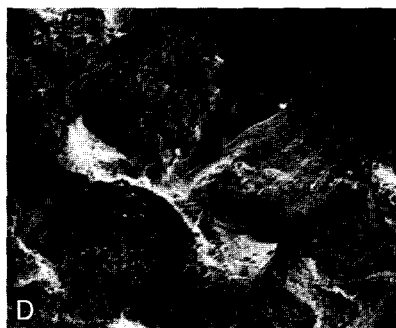
FIG. 14. — Cribrilina gathensis n.sp. Saint-Sauveur-le-Vicomte, la Gathe (Manche), niveau 49,5-52 m. Pliocène inférieur. (R 62715 ; LP, MNHN). A, x 100. B, x 120. C, les trois épines orales sont nettement visibles. Noter la présence des aviculaires latéraux entre la première et la deuxième paire de costules, x 160. D, ovicele avec protubérance médiane, longitudinale et les deux épines orales, x 146.
