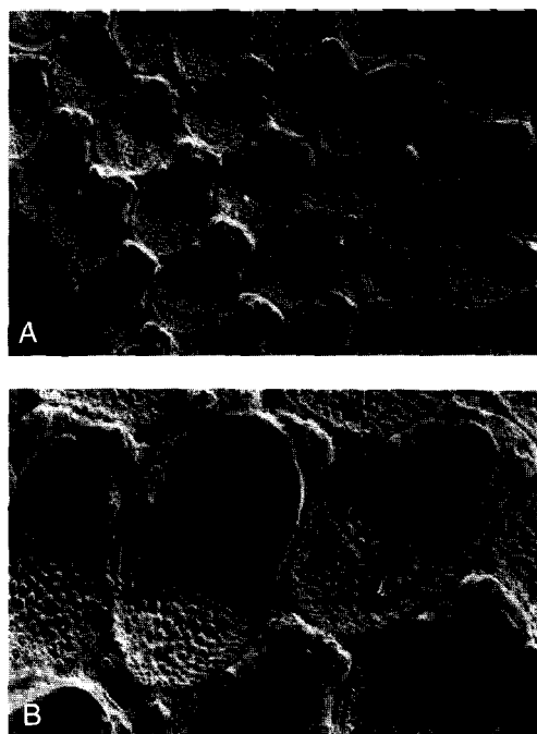
FIG. 10. — Steginoporella brevis punctata Canu et Lecoindre, 1927. Saint-Sauveur-le-Vicomte, la Gathe (Manche), niveau 52-54,5 m. Pliocène inférieur. (R 62714 ; LP, MNHN). A, x 26. B, une zoécie B avec son auvent arrondi. Tubercules visibles. x 62.
