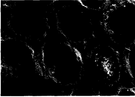
FIG. 5. — Callopora lineata (Linné, 1767). Saint-Sauveur-le-Vicomte, la Gathe (Manche), niveau 49,5-52 m. Pliocène inférieur. (R 62706 ; LP, MNHN). x 80.
