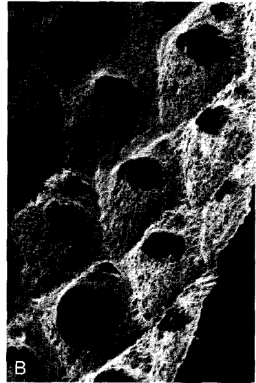
FIG. 11. — Cellaria crassa Wood, 1844. A , Saint-Georges-de-Bohon, réserve de chasse de l'Ermitage 2 (Manche), niveau 38 m. Pliocène inférieur. (R 62710 ; LP, MNHN). x 62. B , Remilly-sur-Lozon, l'Angle (Manche), niveau 12-13 m. Pliocène supérieur. (R 62711 ; LP, MNHN). Aviculaire interzoécial, x 80.
