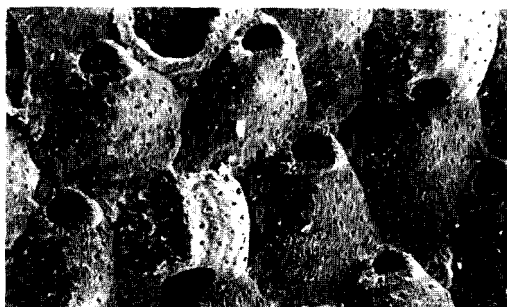
FIG. 15. — Haplopoma graniferum (Johnston, 1847). Saint-Georges-de-Bohon, réserve de chasse de l'Ermitage 2 (Manche), niveau 45 m. Pliocène inférieur. (R 62732 ; LP, MNHN). Portion de zoarium avec zoécies ovicellées. L'ovicelle a une carène médiane. x 52.
