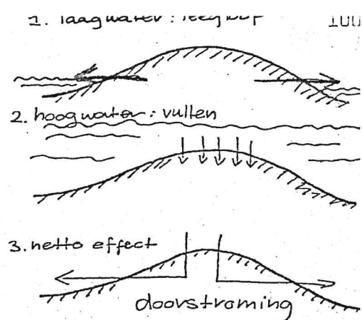
FIGUUR 25 intertidal pump
