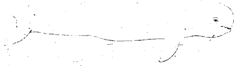
Orcælla bimaculata.
