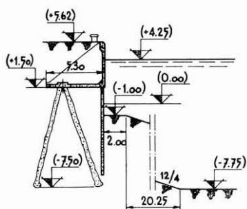
DOORSNEDE E-E
