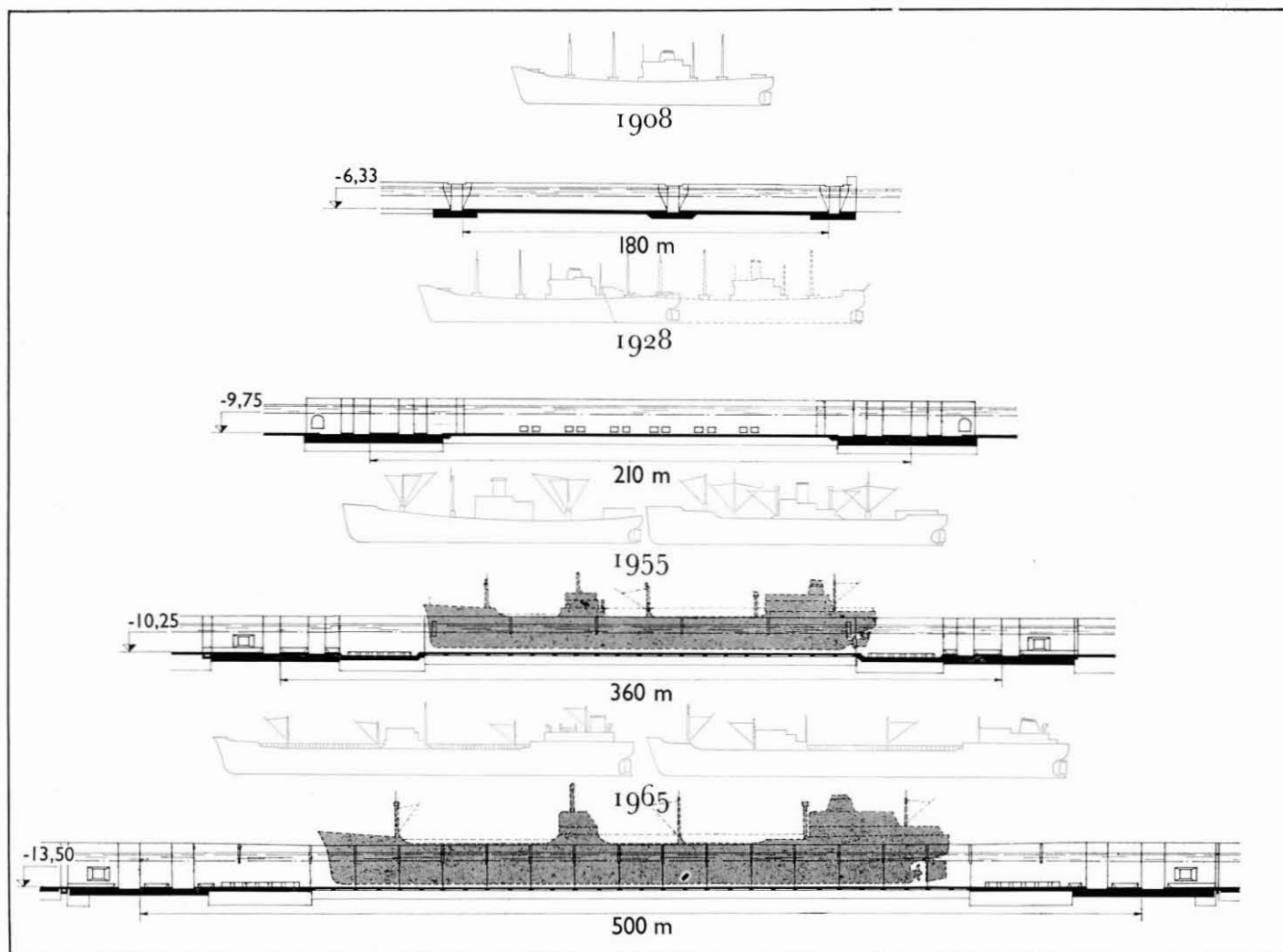
Evolutie van de kolklenge in de schutsluizen te Antwerpen.
