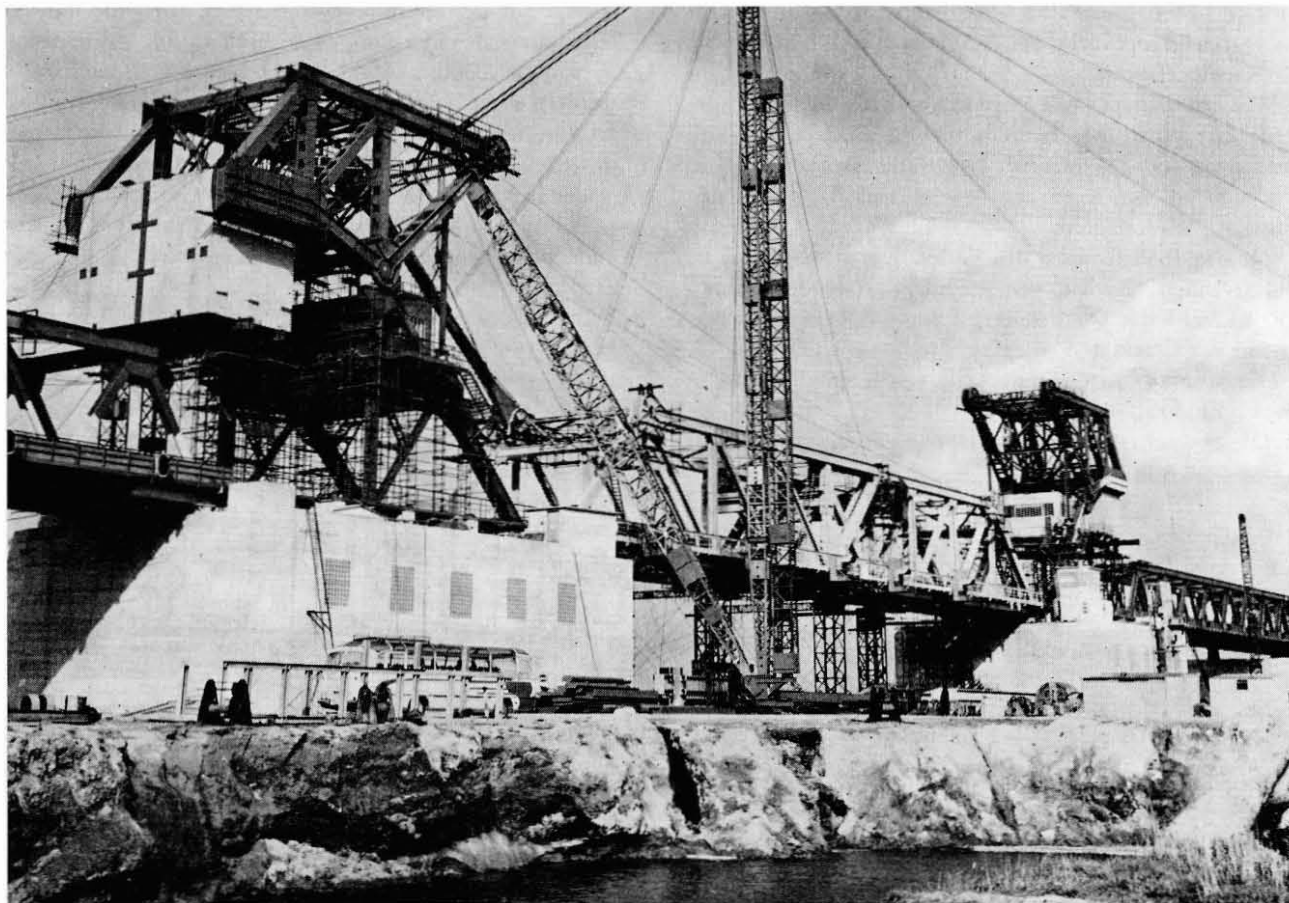
Montagearbeiten (27.2.1967) Montagewerken
