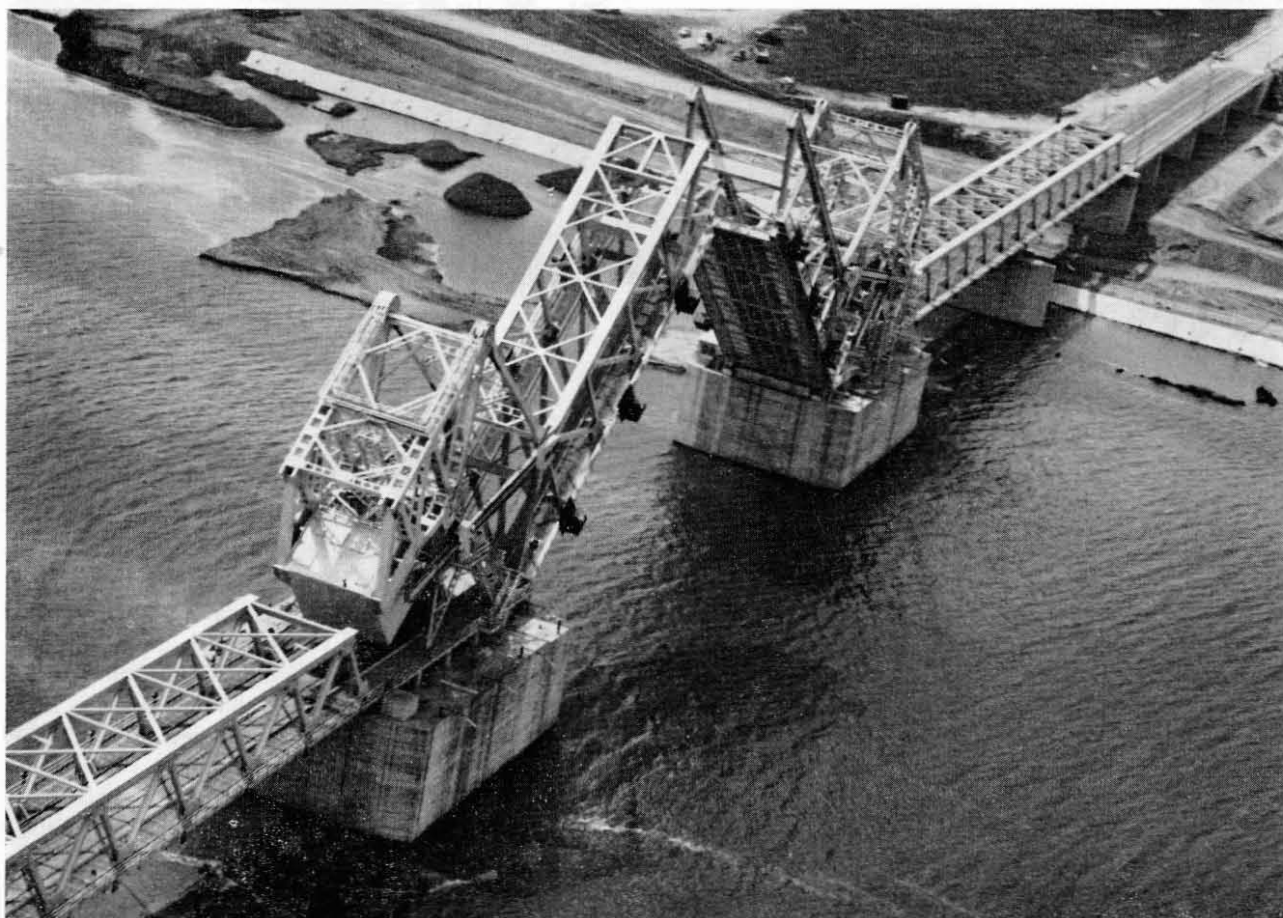
Doppelte Klappbrücke mit festen Warrenbrücken (8.6.1967)
