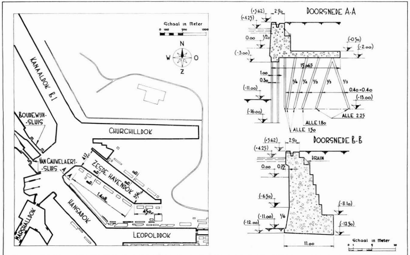
Lageplan und Typen von Kai-mauern Liggingplan en types van kaai-muren Plan de situation et types de murs de quai Situation plan and types of quay-walls
