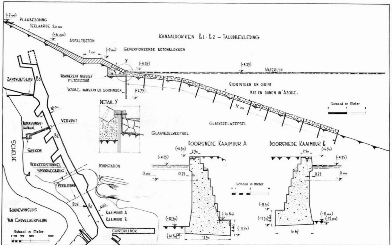
Lageplan und Typen von Kai- mauern und Verkleidung der Böschung
