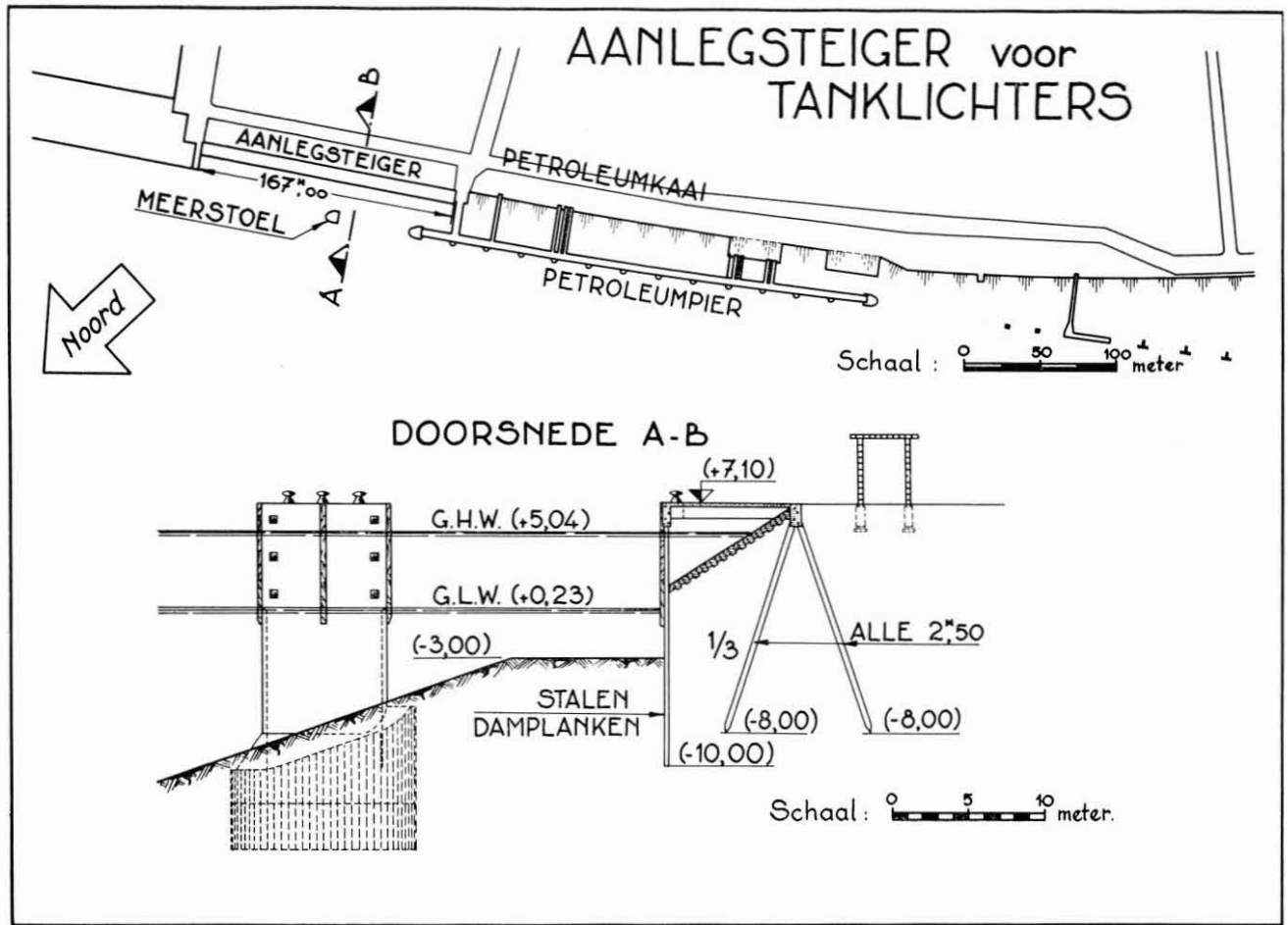
Landungsbrücke für Tanklichter- Aanlegsteiger voor tanklichters Embarcadère pour chalands-ci- Landing-stage for tank-lighters ter ternes
