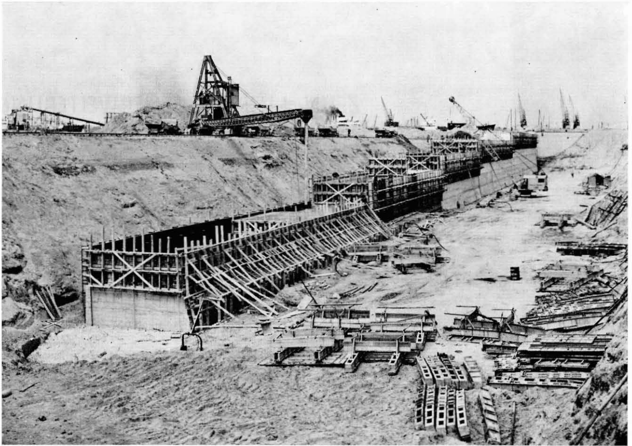
Bau einer Kaimauer (12.6.1958)
