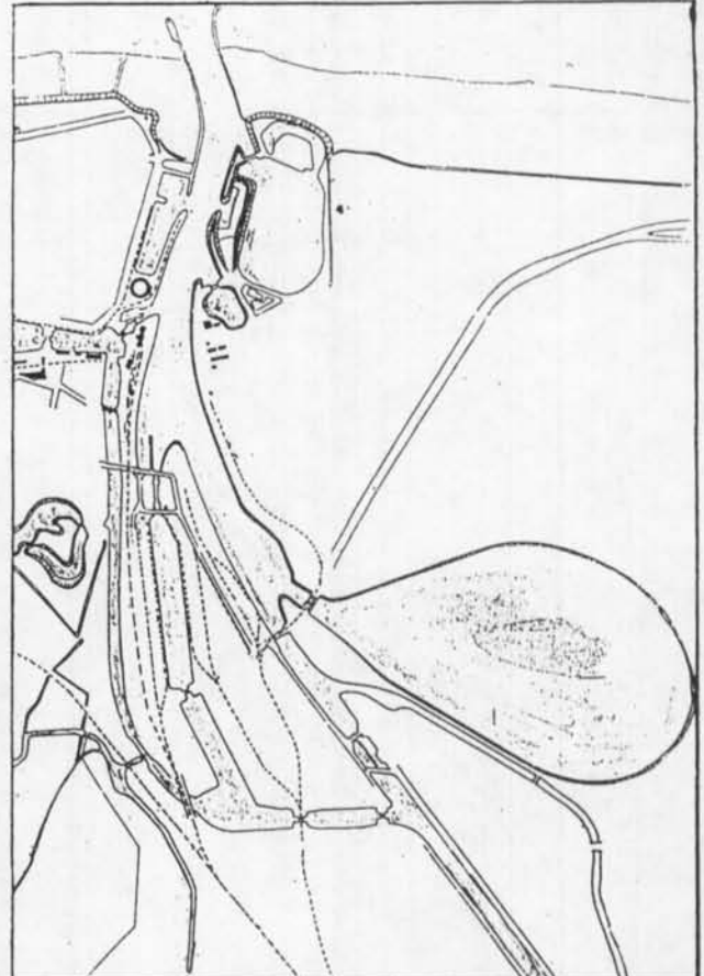
Haven Oostende Situatie 1907
