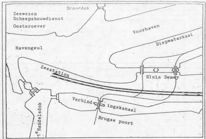
1894 - Origineel ontwerp verbinding Oostende met nieuwe haveninstallaties en Oostkust Fig.20
