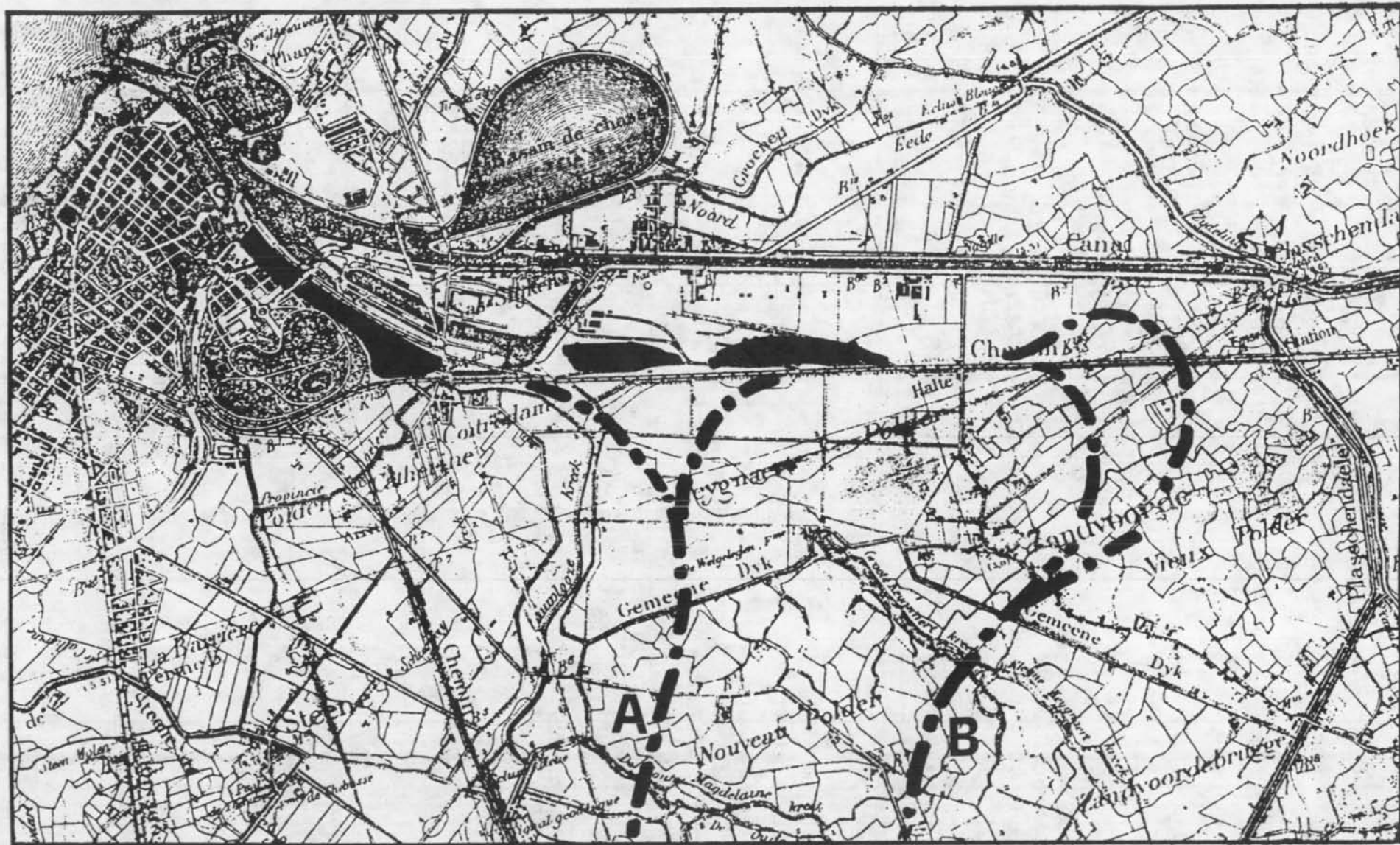
Fig. nr. 10. 1919, ontwerp opgemaakt door de spoorwegen voor de nieuwe spoorinstallaties te Ostende, in functie van de centralisatie van de stations. A: nieuwe lijn, reizigerstreinen, naar Torhout en strategische kustlijn. B: " " , goederentreinen, naar Torhout en strategische kustlijn. ■■■■■ : nieuwe spoorbundels.
