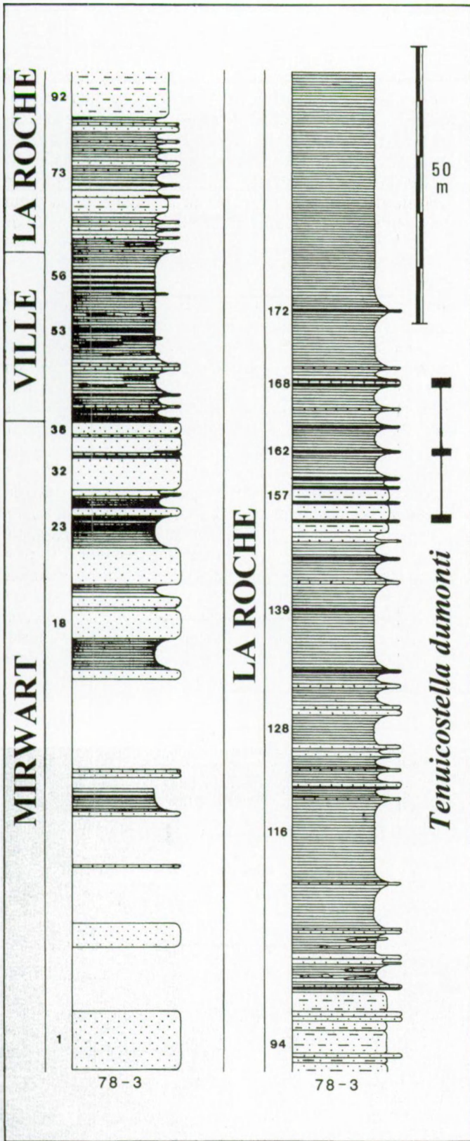
Fig. 8 — Extension verticale de Tenuicostella dumonti dans l'affleurement JG-1978-3. Les noms des formations et les numéros de quelques bancs sont indiqués à gauche de la colonne lithologique.
