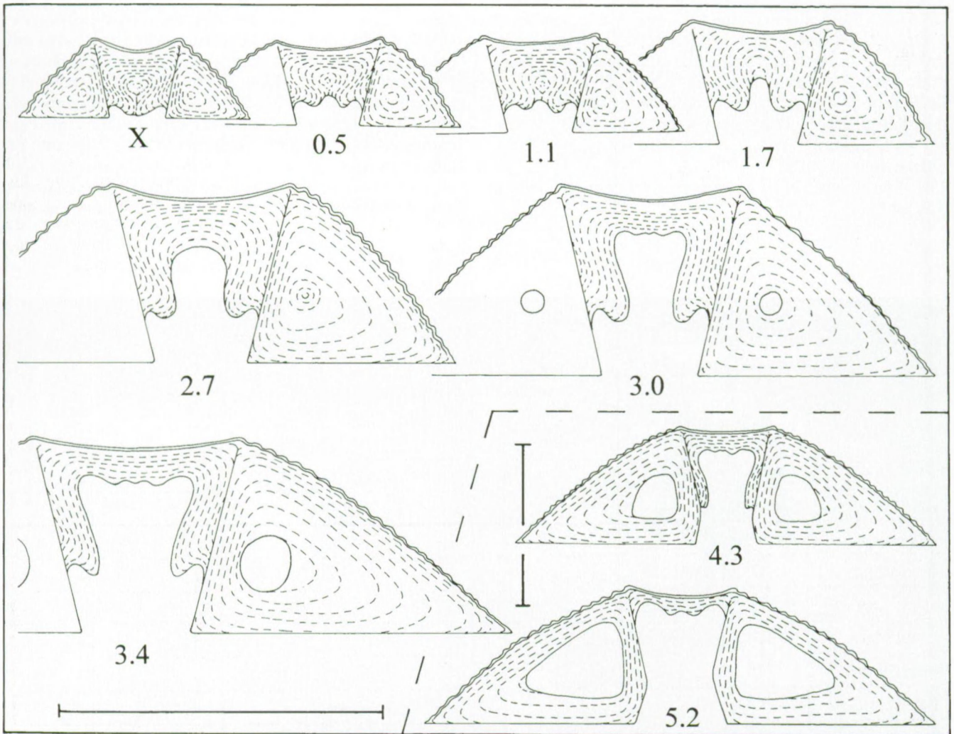
Fig. 6 — Tenuicostella dumonti n. sp. Coupes séries transverses schématiques dans le moulage en plâtre de l'holotype, IRScNB a11287. Les distances en mm sont mesurées à partir de la première section (X). Distance entre la section X et le sommet de l'umbo ventral non mesurée. Les barres correspondent à 1 cm.
