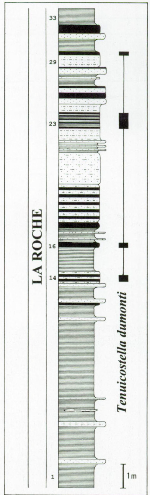
Fig. 9 — Extension verticale de Tenuicostella dumonti dans l'affleurement JG-1973-7. Les noms des formations et les numéros de quelques bancs sont indiqués à gauche de la colonne stratigraphique.
