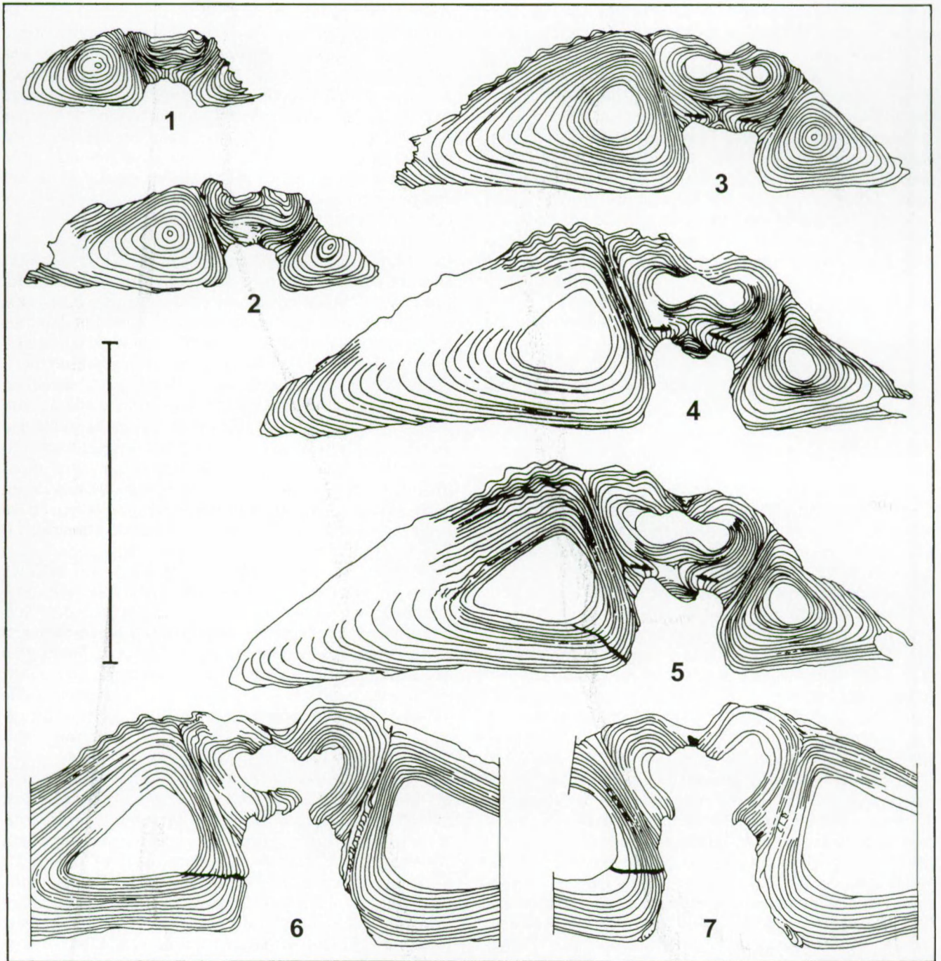
Fig. 2 — Subcuspidella cf. subcuspidata (SCHNUR, 1851). Spécimen IRScNB a11268. Grupont, coupe de la gare, partie sud, banc 1. Coupes sériées transverses dans une valve pédonculaire. Les flèches indiquent la direction de croissance des deux parties de la plaque delthyriale. Distances entre les sections non mesurées. La barre correspond à 1 cm.
