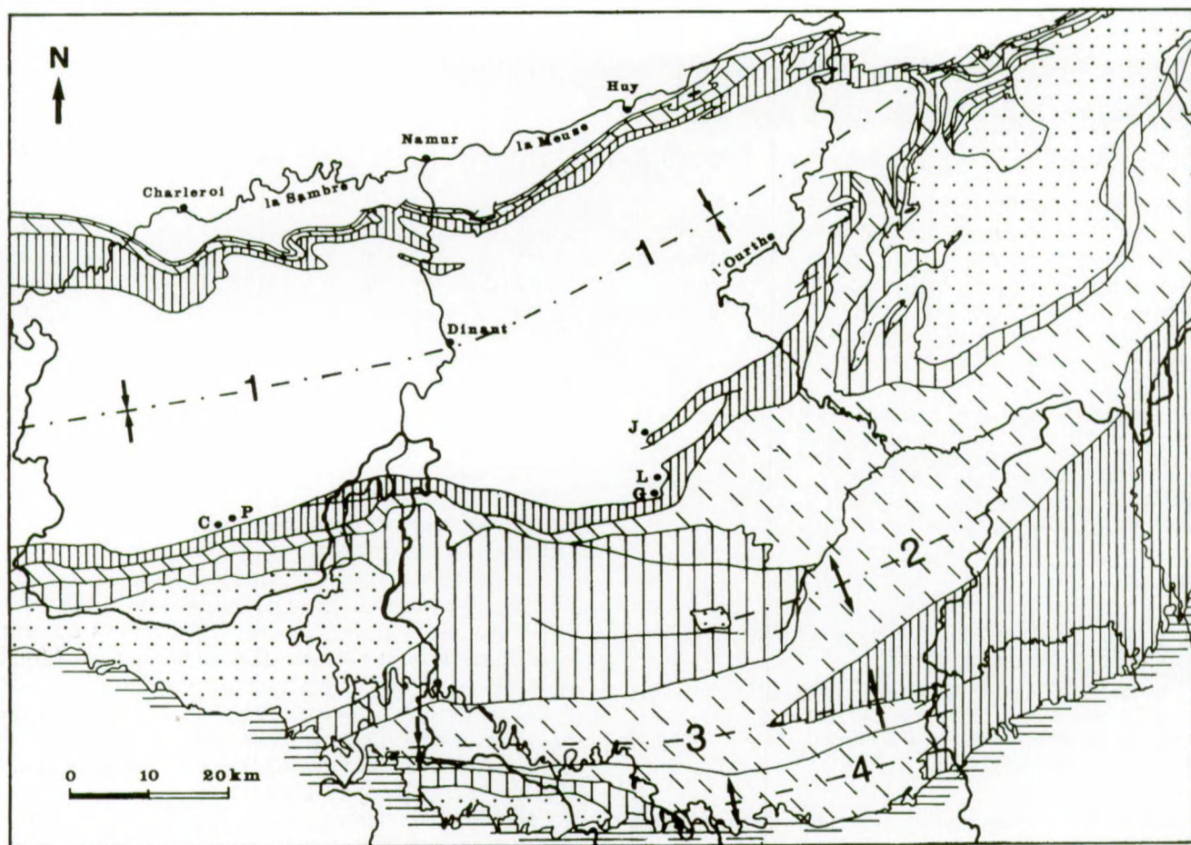
Fig. 1 — Carte géologique schématique du sud de la Belgique avec localisation des gisements fossilifères.
