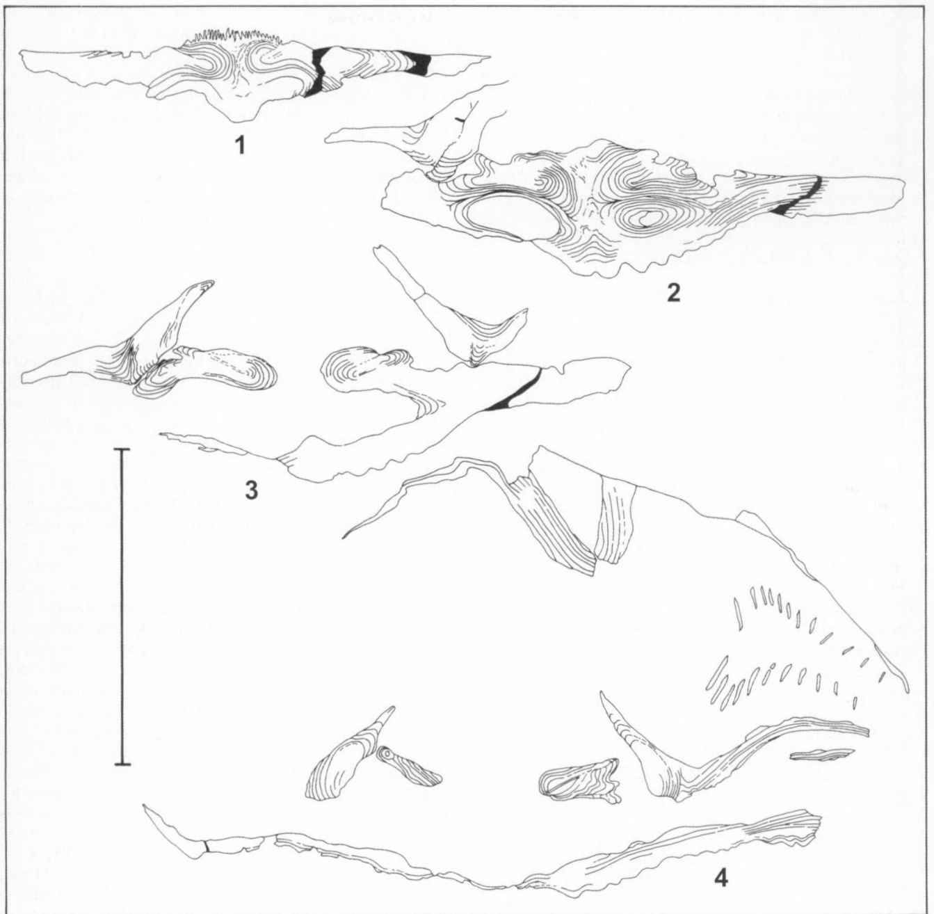
Fig. 3 — Subcuspidella cf. subcuspidata (SCHNUR, 1851). Spécimen IRScNB a11269. Grupont, coupe de la gare, partie sud, banc 1. Coupes séries transverses dans une valve brachiale. Distances entre les différentes sections non mesurées. La barre correspond à 1 cm.
