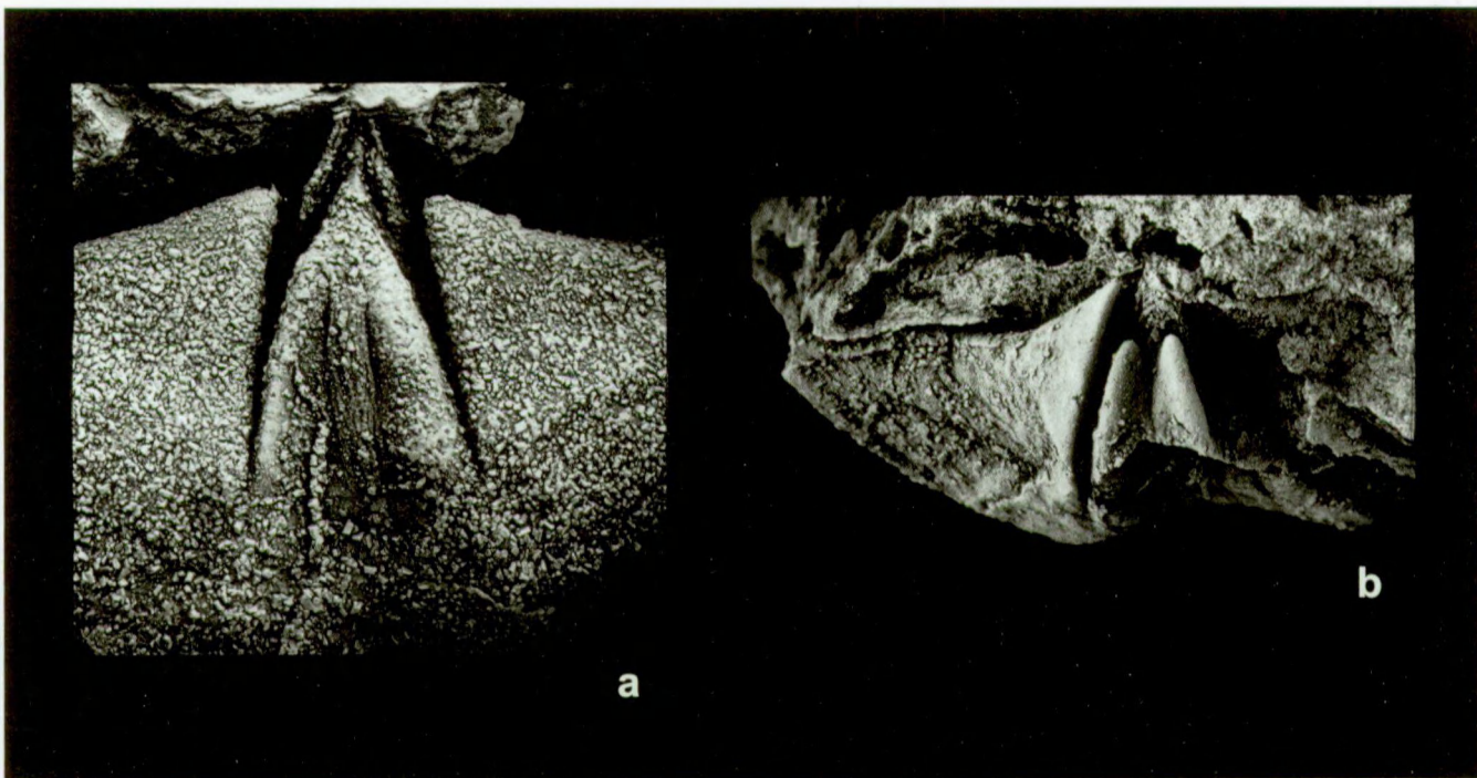
Fig. 7 — Tenuicostella dumonti n. sp. Moules internes montrant la partie postérieure de la valve pédonculaire correspondant à la plaque delthyriale et à la callosité. 7a: holotype, IRScNB a11287; 7b: paratype O, IRScNB a11303. X 3.
