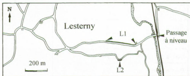
Fig. 4 — Carte de localisation des affleurements L1 et L2 à Lesterny.
