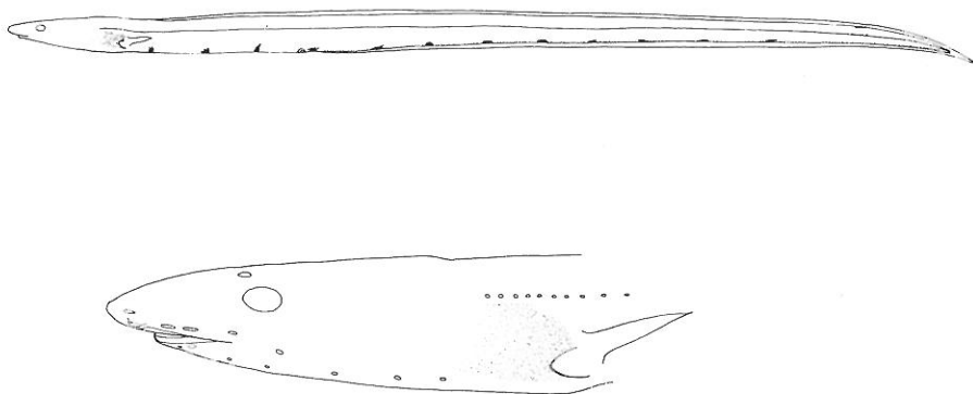
Fig. 1. Acromycter alcocki , juvenile, 116 mm TL, BPBM 21069.
