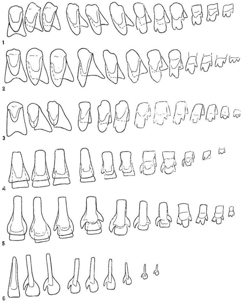
Fig. 3 Radulae
