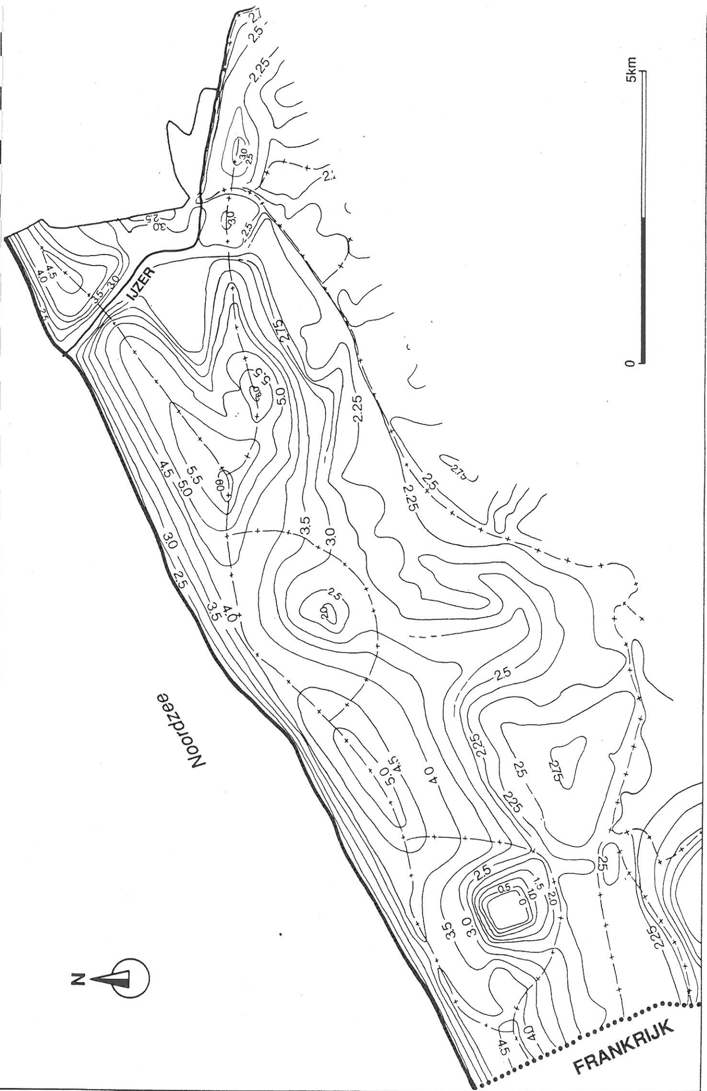
Figuur 4.4: Voedingsgebied voor de waterwinning (LEBBE et al., 1993)
