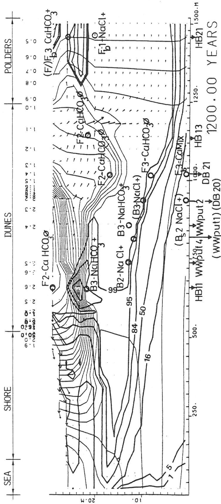
Figuur 3.35: Berekende verspreiding van de grondwaterkwaliteit in profiel K42,8 voor de actuele toestand in het duingebied ten oosten van De Haan. De resultaten van de grondwateranalyses worden weergegeven met de code van de classificatie van Stuyfzand(LEBBE et al., 1990)
