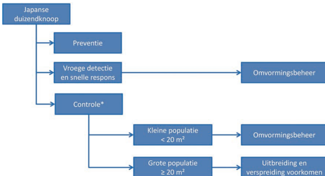
Figuur 74 Flowchart met de drietrapsaanpak voor de invasieve exoot Japanse duizendknoop ( Fallopia japonica ) en verwante soorten (*Controle wordt gedetailleerd in Figuur 76).
