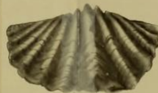
Figs. 1, 2, 2a. — Figures attribuées, avec doute, au Sp. Decheni , du Coblentzien de St-Michel. — F. BÉCLARD, 1887.
