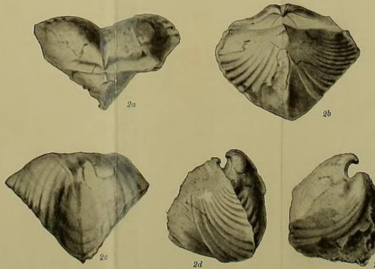
Figs. 2a-e. BURNOTIEN. — Loc. Petigny.
