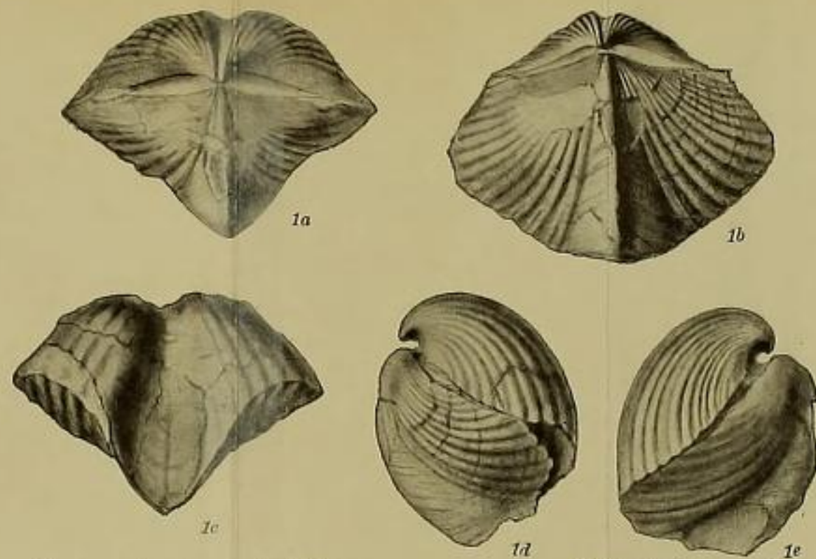
Figs. 1a-e. BURNOTIEN. — Loc. Petigny.
