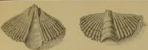
Figures de Sp. hystericus , de la Gravelle de Kayserstuhl. — Schuchert, 1891. T. IV.
