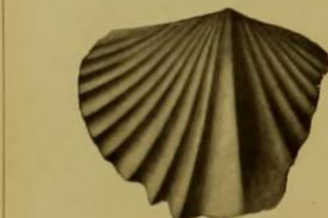
VI. Figures du Sp. Decheni , du Devonien inférieur de Joachimskopf. — F. KATSER, 1878.
