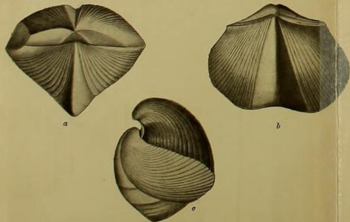
II. Figures du Sp. acuminatus , du Calcaire cornifère (Upper Helderberg group) des États-Unis d'Amérique. — J. HALL, 1861-66.
