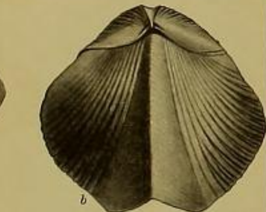
IV. Figures du Sp. cultrijugatus , a. Moule de la Grauwacke; b. Coquille du Calcaire de l'Eifel. — QUENSTEDT, 1871.
