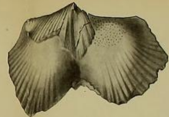
Fig. 3. BURNOTIEN. — Feuille de Couvin, n° 8711.
