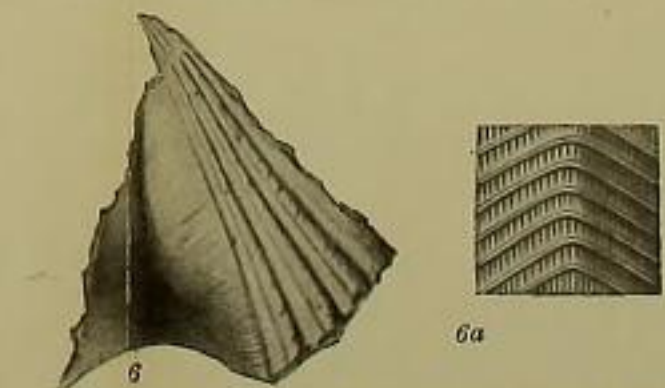
Figs. 6, 6a. BURNOTIEN. — Feuille de Treignes, n° 8370.
