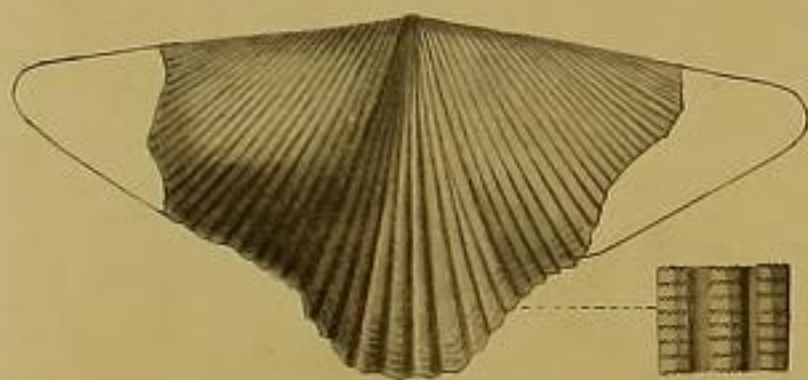
I. Figures du Sp. Triggeri , du Devonien inférieur de l'Asie Mineure. — DE VERNEUIL, 1866-69. TYPE.
