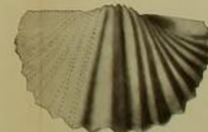
Fig. 10. TAUNUSIEN. — Feuille de Couvin, n° 8724.
