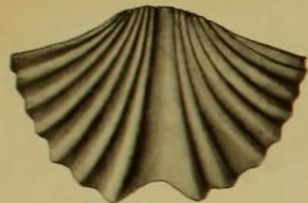
I. Figure du Sp. primævus , de la Grauwacke de Herdorf. — STERNBERG, 1853.
