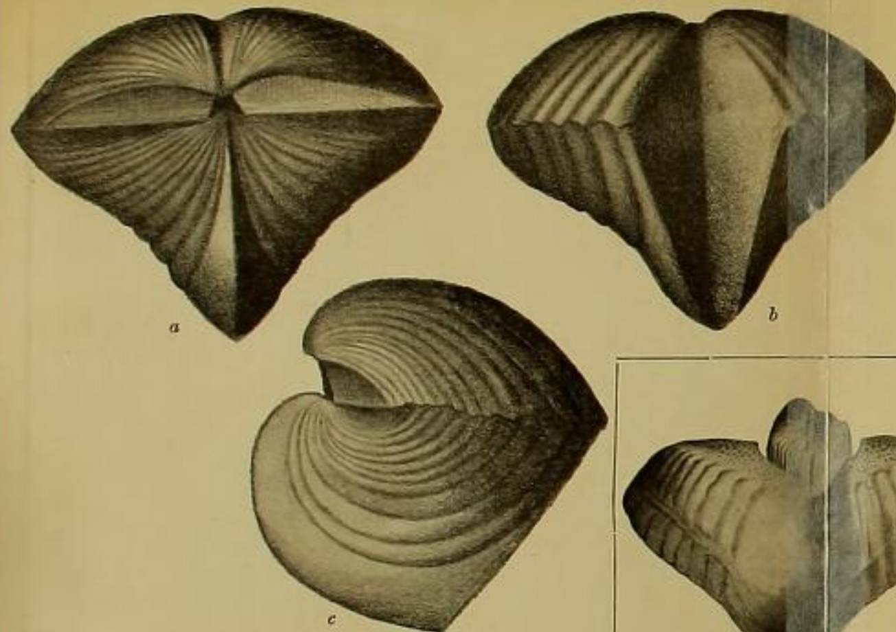
I. Figures du Sp. cultrijugatus , du Calcaire de l'Eifel. — C.-F. ROEMER, 1844. TYPE.
