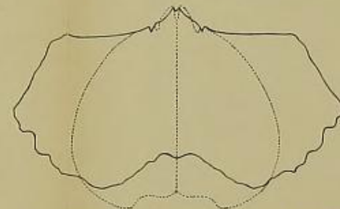
Fig. 4. — Contours superposés d'un moule de la forme auriculatus et d'un moule de la forme cultrijugatus , pour montrer les limites de variation.
