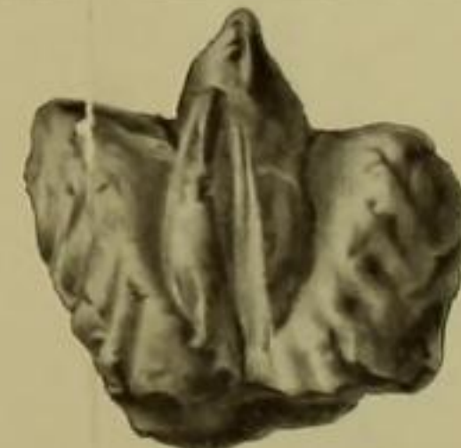
Fig. 5. HUNSBUCKIEN de St-Michel.
