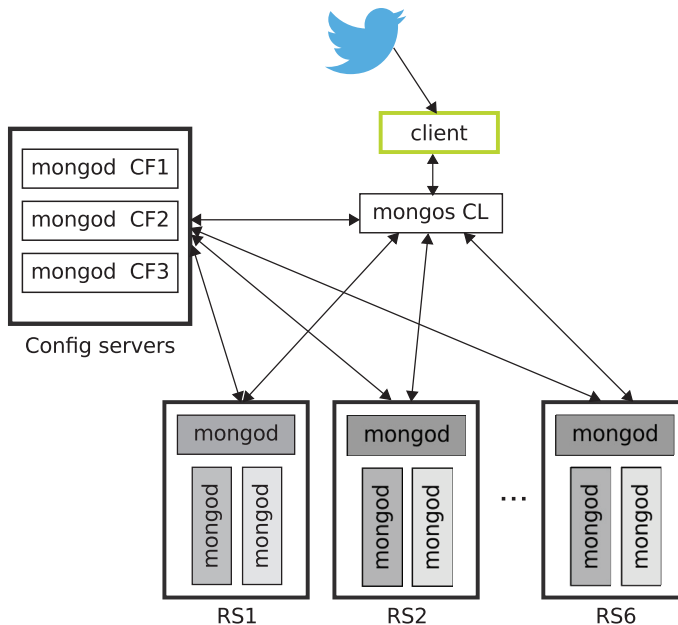
Fig. 3. Global MongoDB Configuration
