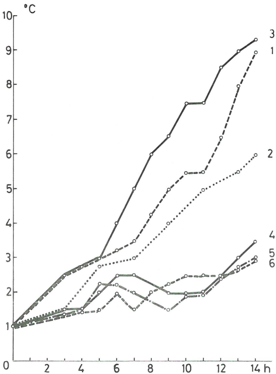
FIG. 9 — TEMPERATUURVERLOOP VAN DE MIDDENSTE VIS
