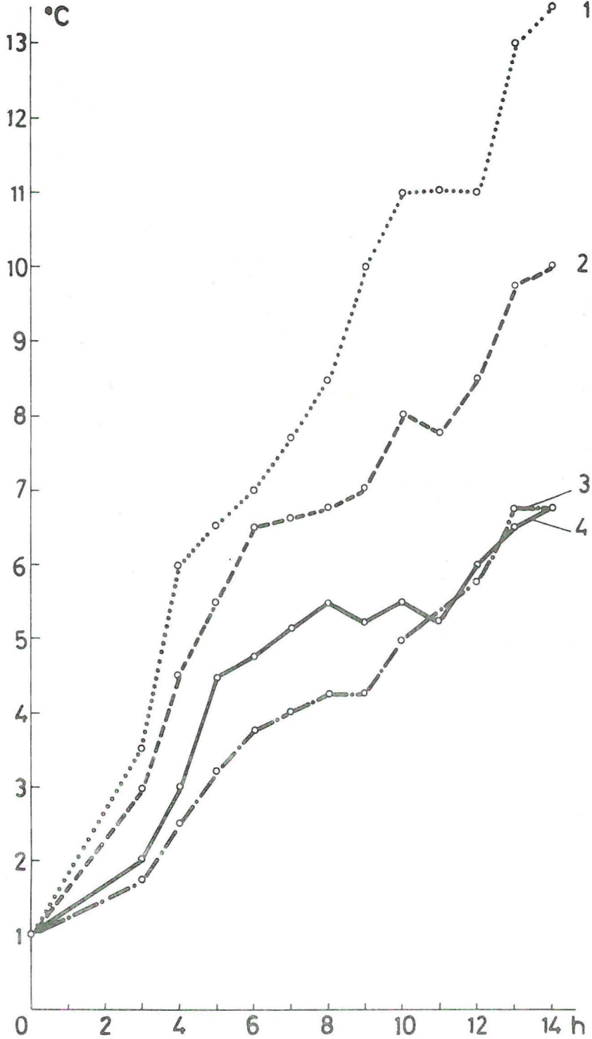
FIG. 11 — TEMPERATUURVERLOOP VAN NIET AFGEIJSDE VIS IN, OP ELKAAR GESTAPELDE PLASTIEKEN KISTEN
