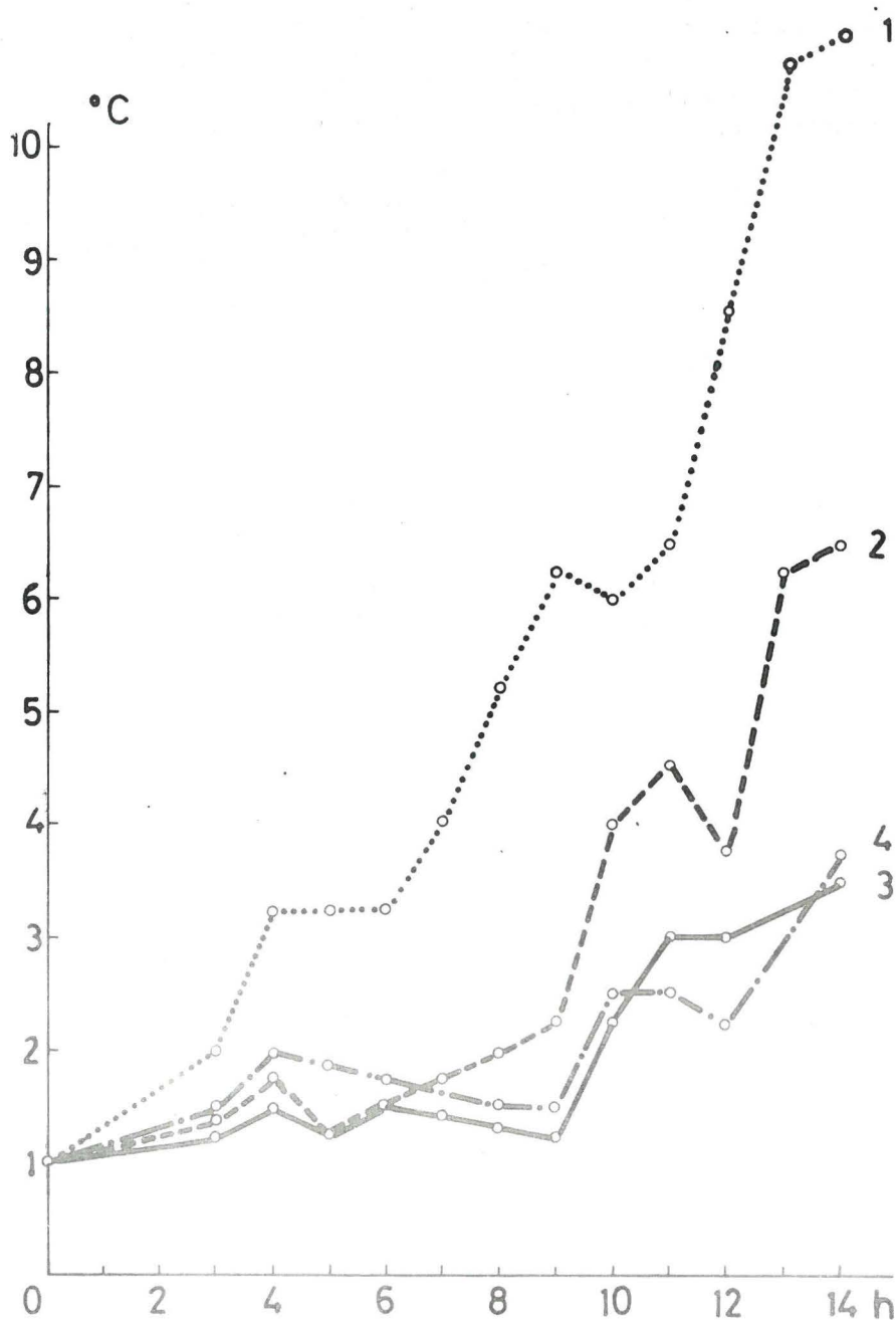
FIG. 12 — TEMPERATUURVERLOOP VAN DE AFGEIJSTE VIS IN, OP ELKAAR GESTAPELDE PLASTIEKEN KISTEN
