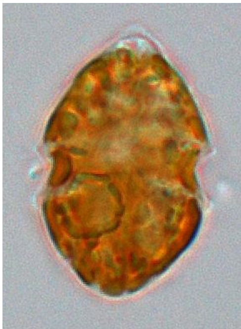
Fig. 30. Heterocapsa circularisquama in Japan.
