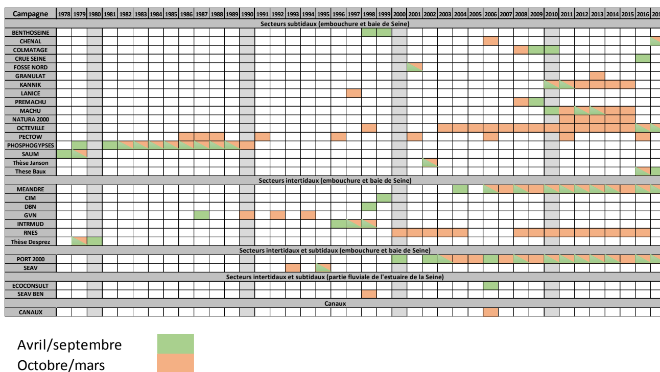
Figure 3: Etendue temporelle des suivis intégrés dans la BD MABES de 1978 à 2017.
