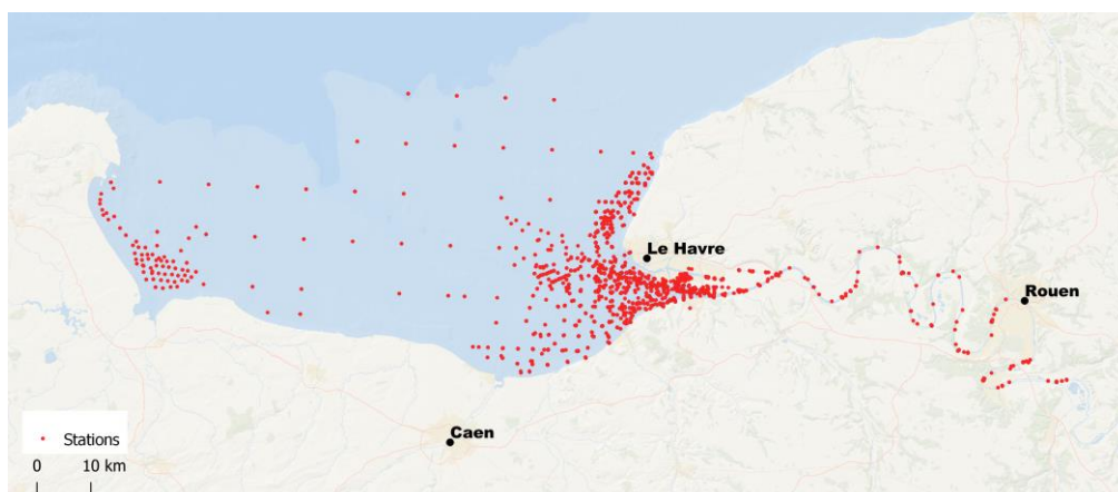
Figure 4: Carte de l'emprise spatiale des suivis intégrés dans la BD MABES.
