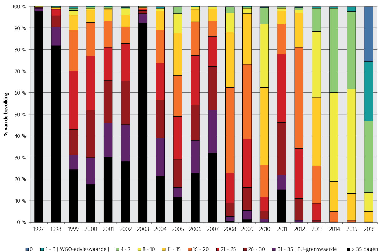
Figuur 5.8: Aandeel bevolking blootgesteld aan dagen met een gemiddelde concentratie > 50 µg/m 3 (RIO)
