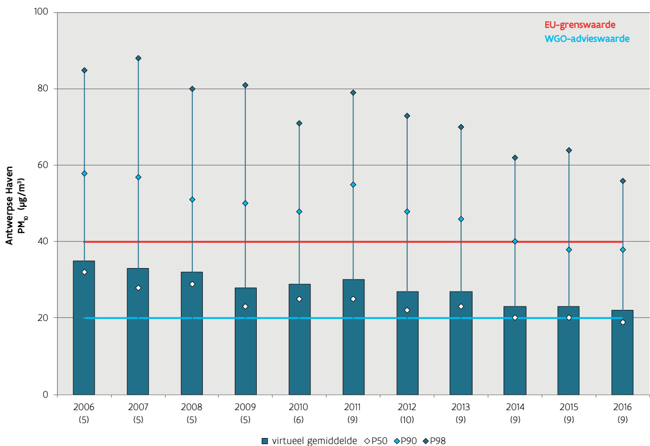
Figuur 11.15: Trend PM_{10} voor de virtuele meetplaats 'Antwerpse haven', 2006-2016
