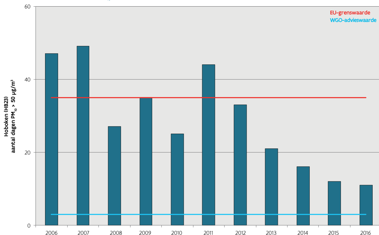
Figuur 11.46: Aantal dagen met PM_{10} -concentratie > 50 \mu\text{g}/\text{m}^3 in Hoboken, 2006-2016
