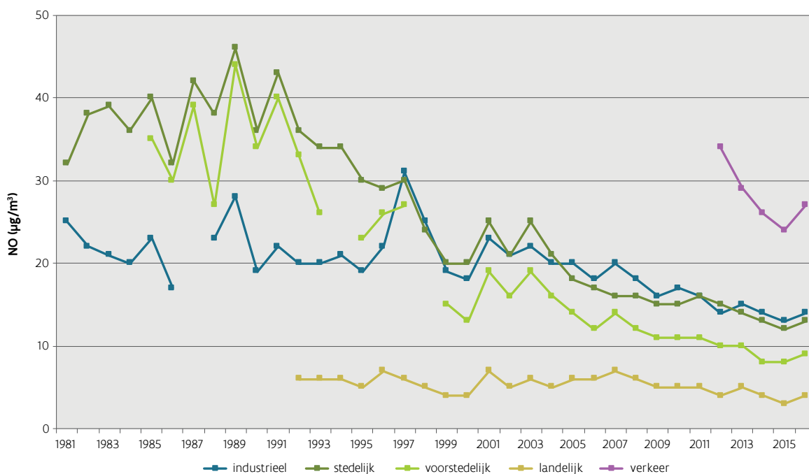
Figuur 3.5: Trend van NO-jaargemiddelden voor de verschillende virtuele meetplaatsen, 1981-2016
