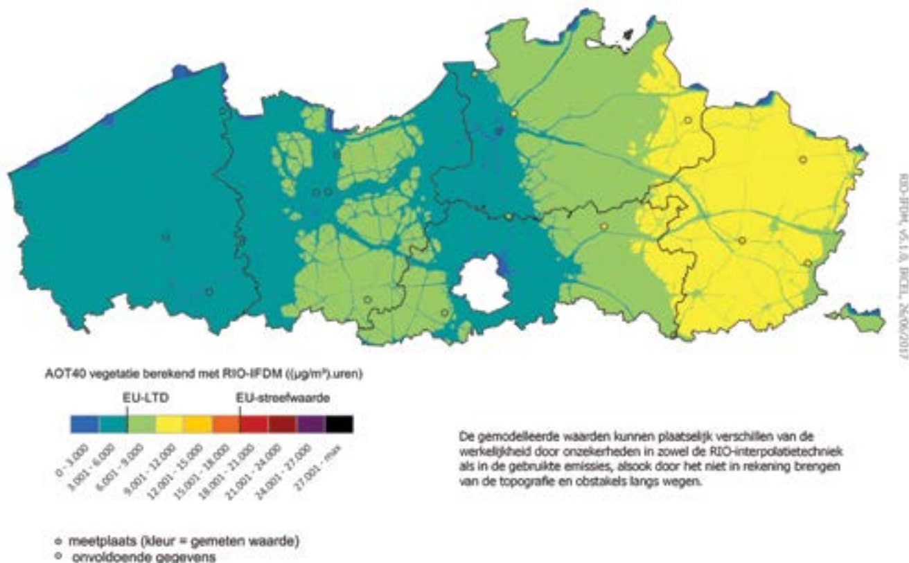
Figuur 4.9: Ruimtelijke spreiding van AOT40 ppb -vegetatie voor de bescherming van gewassen en seminatuurlijke vegetatie in 2016
