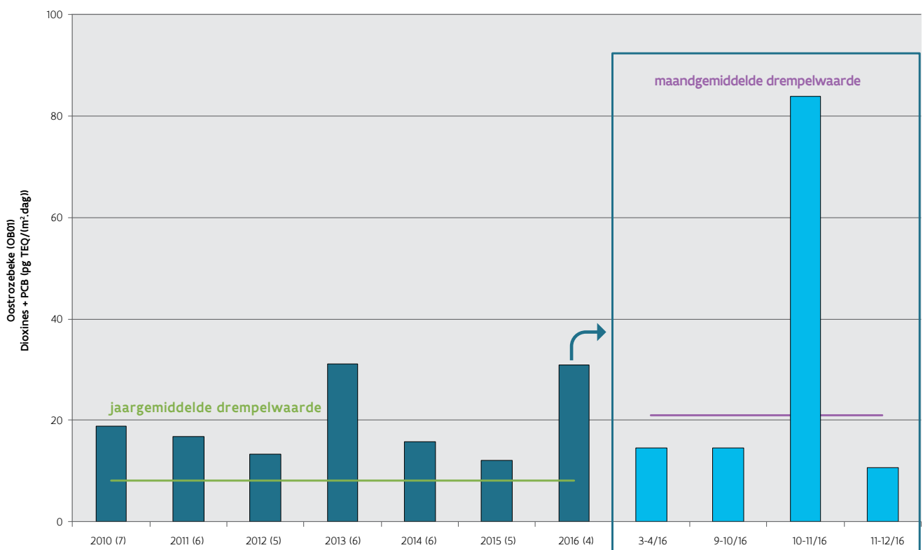
Figuur 11.54: Toetsing van jaargemiddelde en maandgemiddelde dioxine- en PCB-depositie op meetplaats OB01 aan de drempelwaarden
