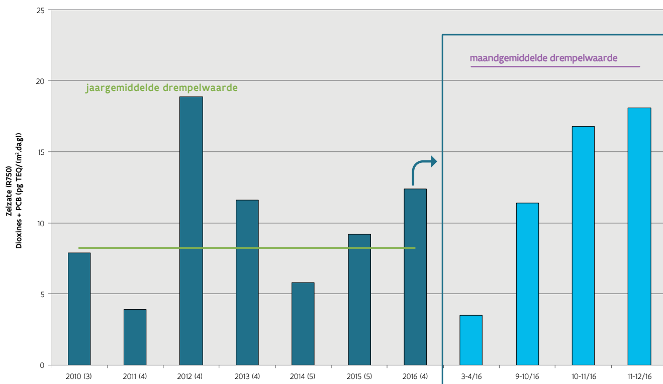
Figuur 11.29: Toetsing van jaargemiddelde en maandgemiddelde dioxine- en PCB-depositie op R750 in Zelzate aan de drempelwaarden
