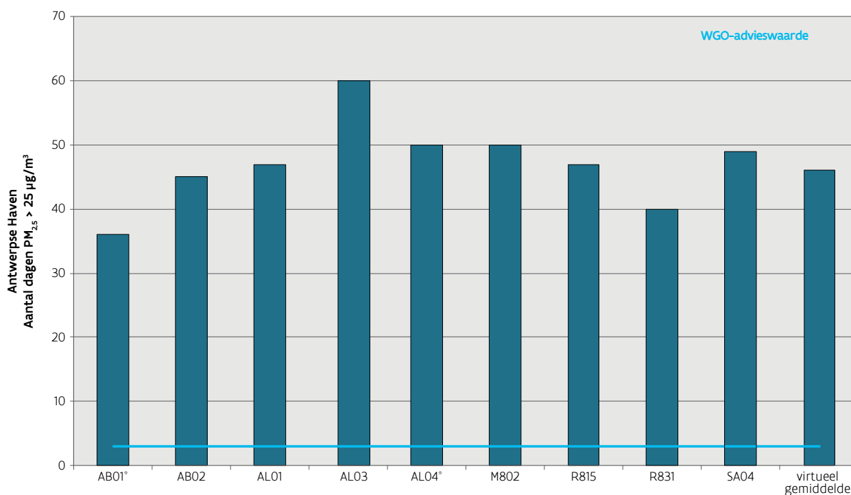
Figuur 11.18 : Aantal dagen met PM_{2.5} -concentratie > 25 \mu\text{g}/\text{m}^3 voor de meetplaatsen in de Antwerpse haven in 2016
