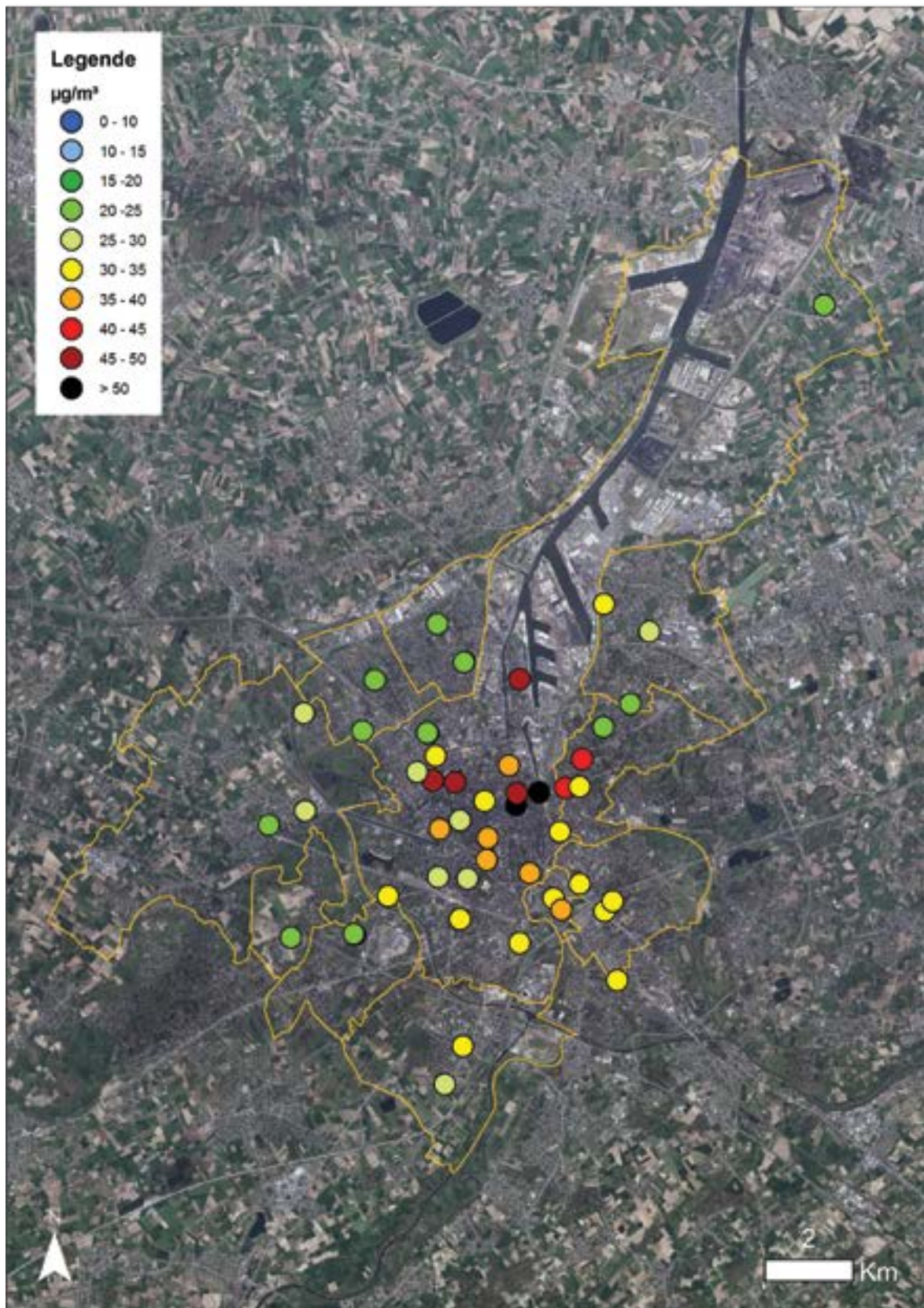
Figuur 13.1: Indicatieve jaargemiddelde \text{NO}_2 -concentratie in Gent
