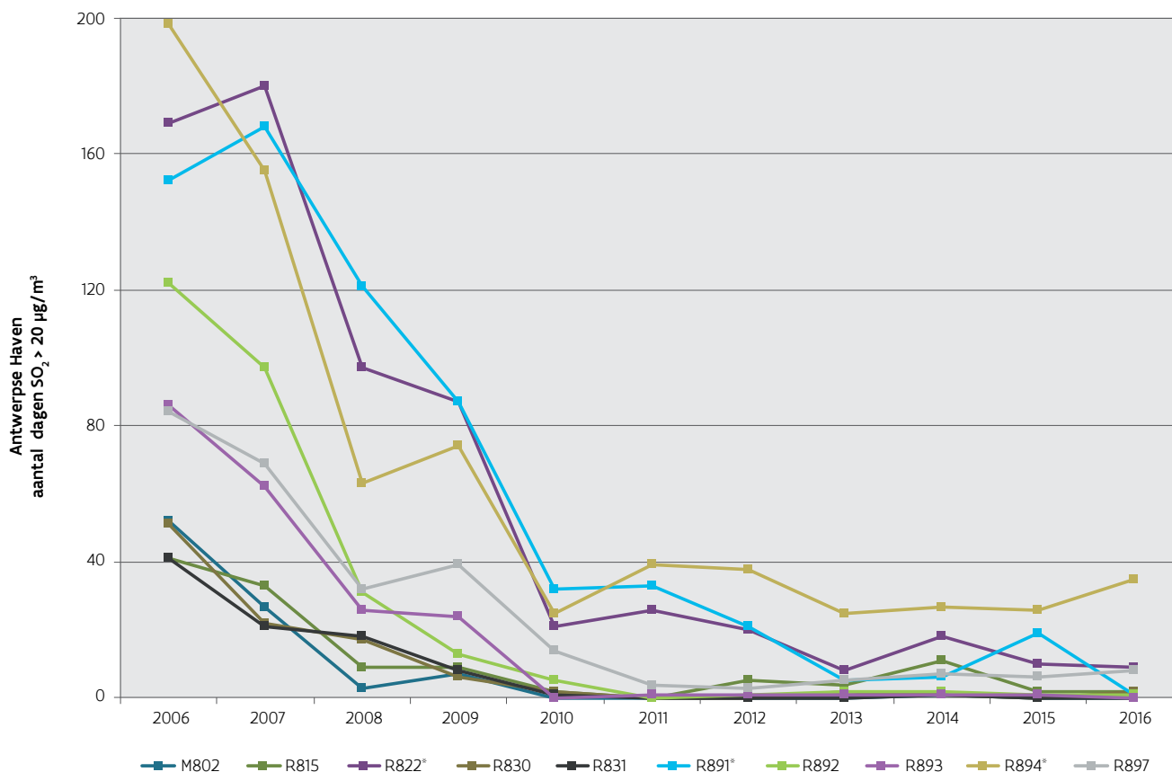
Figuur 11.22: Aantal dagen met een SO 2 -concentratie > 20 µg/m 3 voor de meetplaatsen in de Antwerpse haven, 2006-2016
