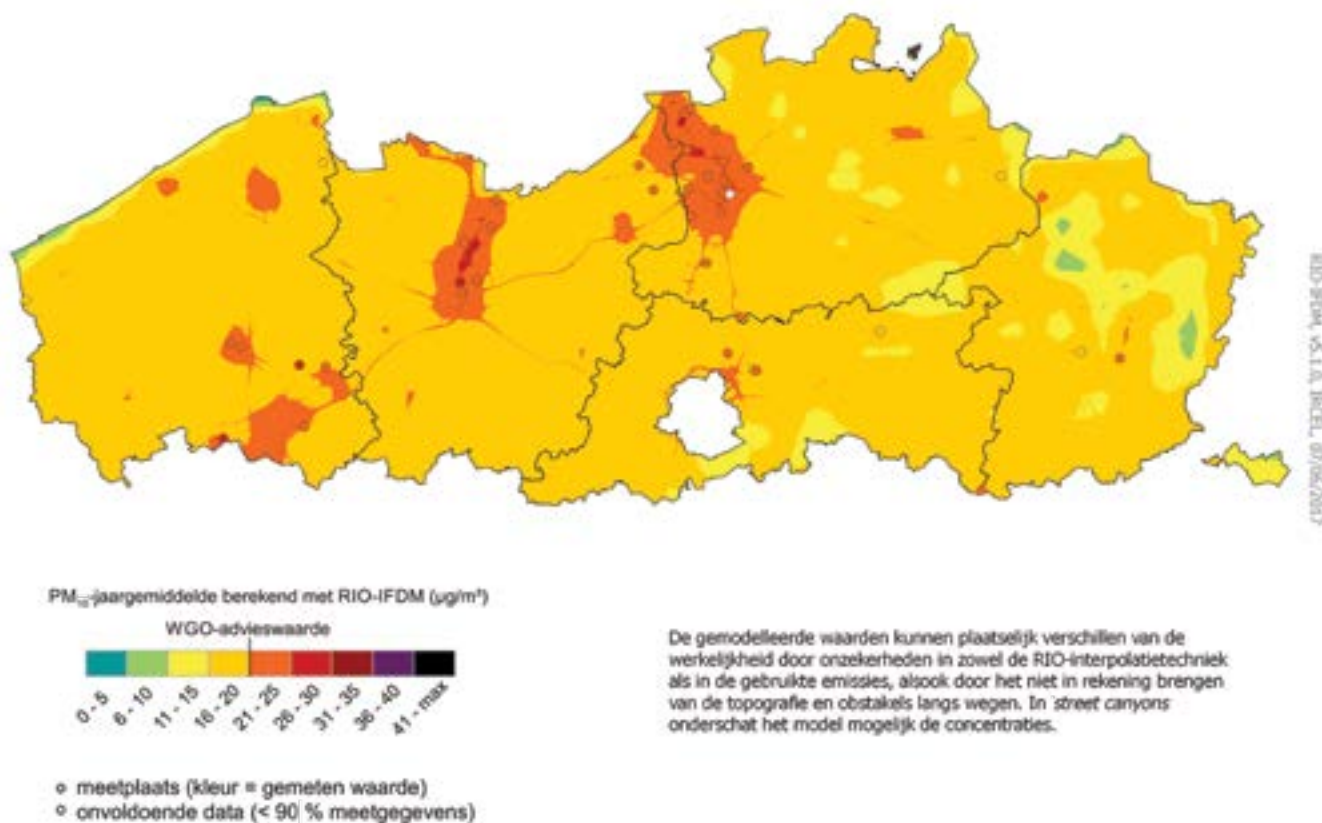
Figuur 5.3: Gemodelleerde PM_{10} -jaargemiddelden in 2016 getoetst aan de WGO-jaaradvieswaarde
