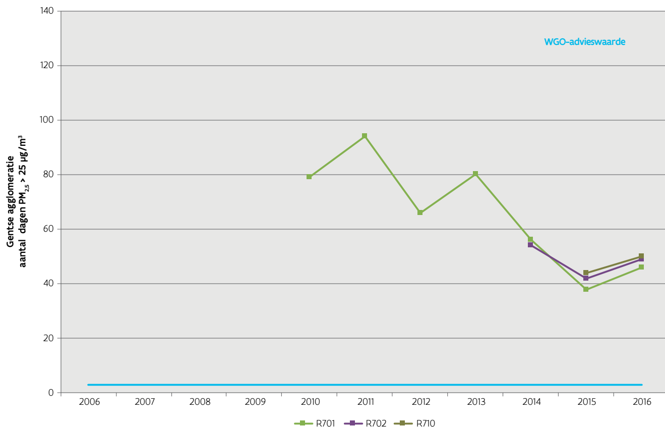
Figuur 11.13: Aantal dagen met PM_{2.5} -concentratie > 25 \mu\text{g}/\text{m}^3 voor de meetplaatsen in de agglomeratie Gent, 2006-2016
