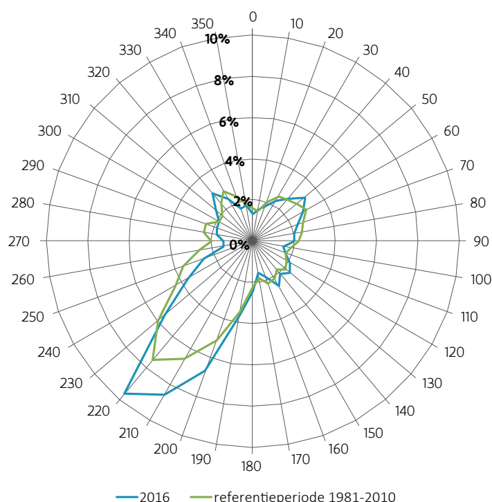
Figuur 1.2: Windroos van de meetplaats Antwerpen-Luchtbal voor het jaar 2016 en de referentieperiode (1981-2010)
