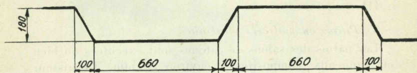
Cloisons étanches en tôles embouties
