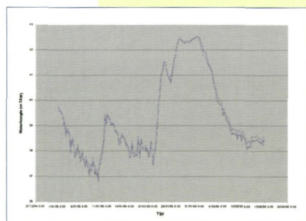
Ijkingsresultaten van het model van de Gemeenschappelijke Maas.
