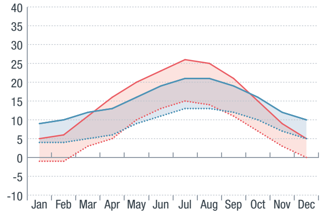
BREST — Temp. max. (°C) ..... Temp. min. (°C) STRASBOURG — Temp. max. (°C) ..... Temp. min. (°C)
