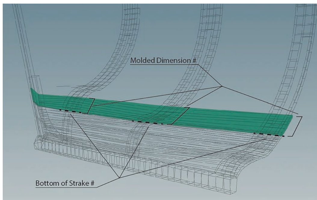
Fig. 8.8 Planking parameters
