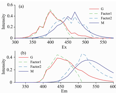
图 6 GM 混合油样本各组分真实光谱与解析光谱
