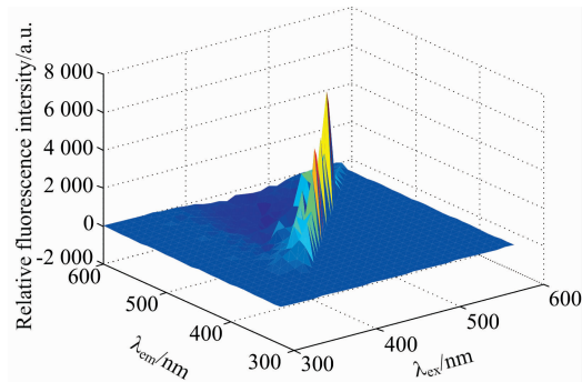
图 2 GM 5 三维荧光导数光谱
