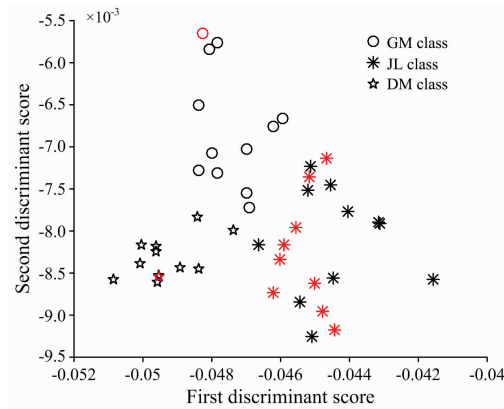
图 4 混合油样本的判别式得分散点图
