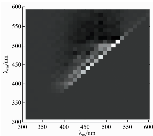
图 3 GM 5 三维荧光导数光谱灰度图
