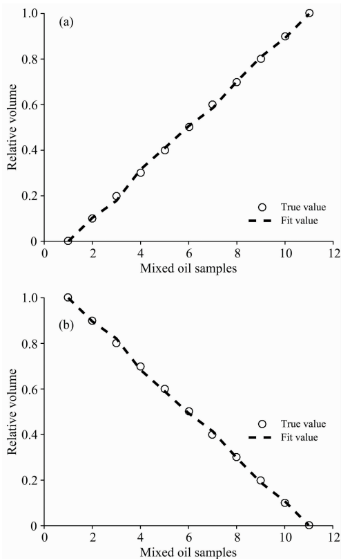
图 5 GM 混合油样本的定量模型
