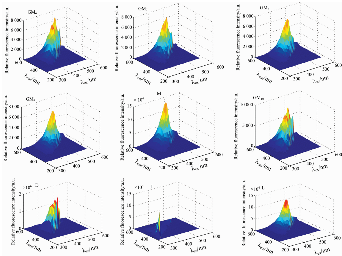
图 1 部分样本的三维荧光光谱
