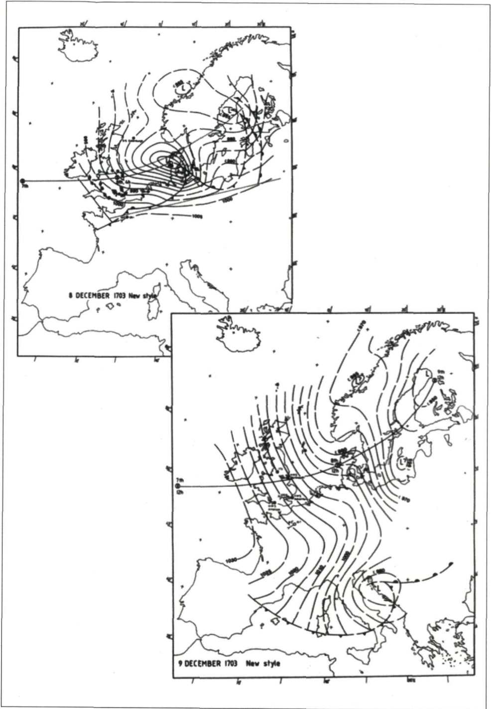
Figuur 2. Synoptisch weer in West-Europa op 8 en 9 december 1703 (Lamb 1991: 68).
