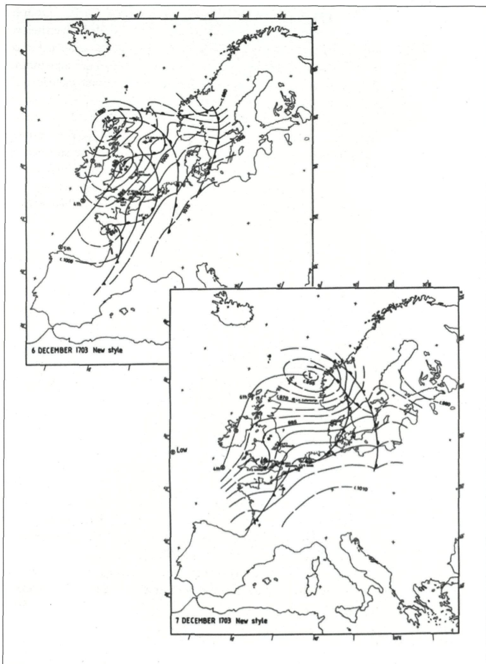
Figuur 1. Synoptisch weer in West-Europa op 6 en 7 december 1703 (Lamb 1991: 67).
