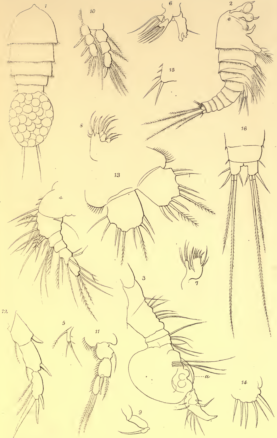
Tachidius brevicornis
