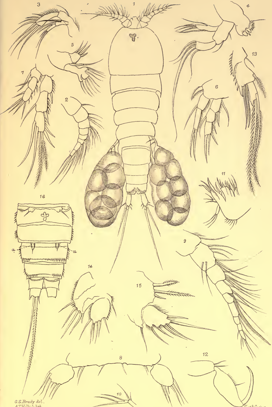
1-8 Delavalia palustris . ♀ 9-16 Thalestris harpactoides .
