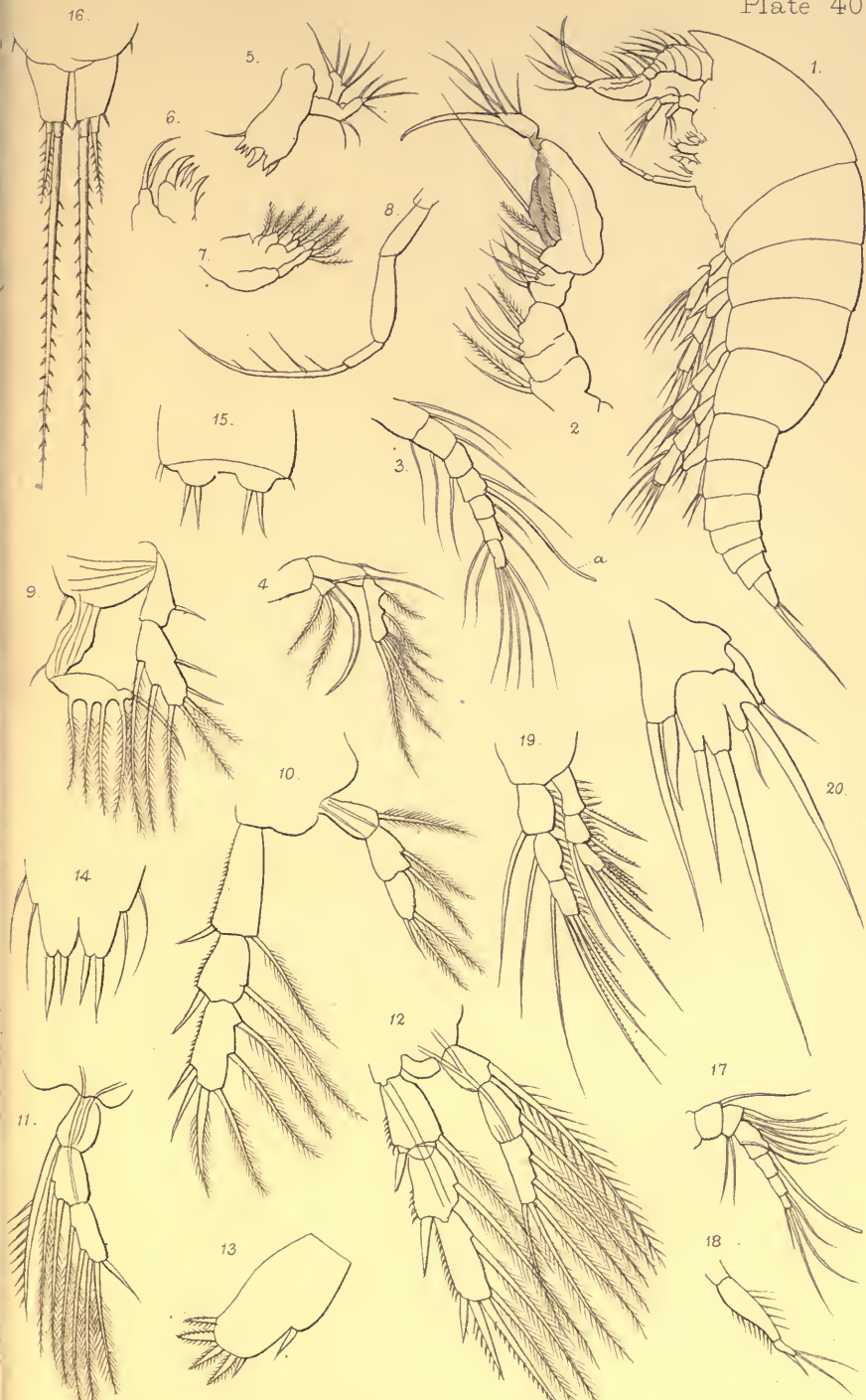
1-16. Euterpe gracilis . 17-20. Ectinosoma melaniceps .
