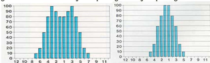
Afbeelding 43: Spuitbeeld van een holle (links) en een volle (rechts) werveldop
