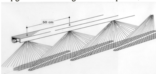
Afbeelding 39: Standaard spleetdop
