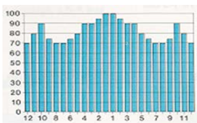
Afbeelding 44: Vloeistofverdeling van een ketskop
