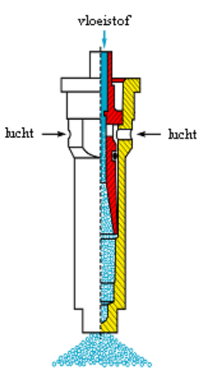
Afbeelding 42: Luchtmengdop
