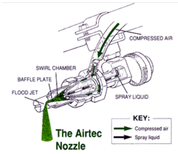
Afbeelding 45: Airtec spuitdop (Cleanacres Machinery Ltd)
