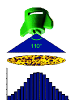
Afbeelding 40: Vloeistofverdeling bij spleetdoppen met een tophoek van 110°
