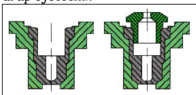
Afbeelding 41: Constructie standaard spleetdop (links) en driftreducerende spleetdop (rechts)
