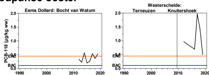
Figuur 35 Gehalten van PCB-118 uit monitoringsjaren 1991 t/m 2019 uitgedrukt op basis van natgewicht gemeten in de levers van Bot en Schol en schelpdiervlees van Blauwe mossel en Japane oester uit de passieve biologische monitoring in zoutwater t.b.v. OSPAR. De blauwe lijn geeft de BAC aan en de oranje lijn de EAC.
