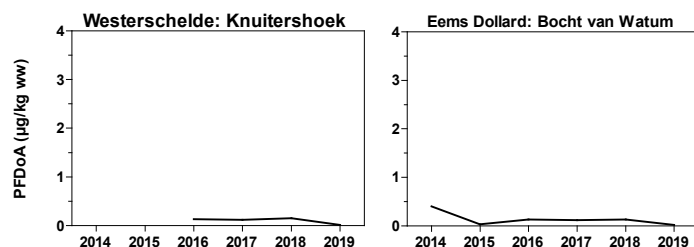
Figuur 55 Gehalten van PFDoA uitgedrukt op basis van natgewicht gemeten in de levers van Bot en Schol en schelpdiervees van Blauwe mossel en Japanse oester uit de passieve biologische monitoring in zoutwater.
