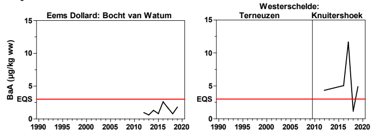
Figuur 11 KRW toetswaarden van benzo(a)antraceen 1992 t/m 2019 uitgedrukt in natgewicht standaard schelpdier gemeten in de passieve biologische monitoring van schelpdieren in zoutwater. De rode lijn geeft de EQS biota aan.
