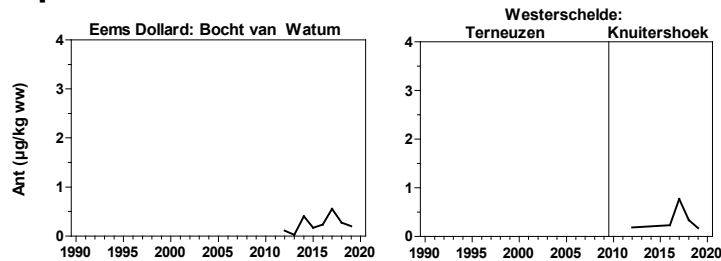
Figuur 9 Gehalten van antraceen 1992 t/m 2019 uitgedrukt in drooggewicht gemeten in de passieve biologische monitoring van Blauwe mossel en Japane oester in zoutwater t.b.v. OSPAR.
