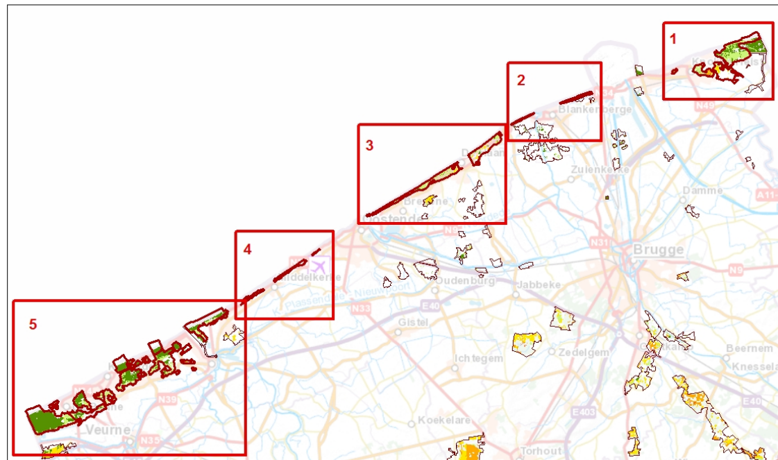
Figuur 2.1 Overschrijding van de kritische depositiewaarde van de actueel aanwezige habitats, op basis van de gemodelleerde stikstofdeposities volgens het VLOPS17-model, dat gebruik maakt van emissie- en meteorologische gegevens van het jaar 2012, en de vectoriële habitatkaart, uitgave 2016 (De Saeger et al. 2016)
