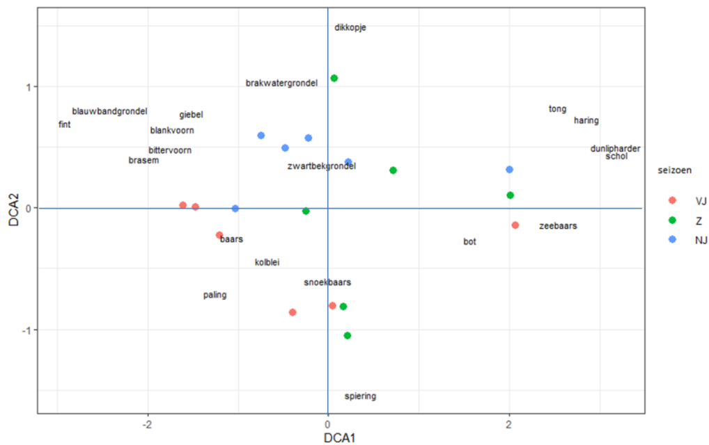
Figuur 12. DCA-ordinatie van de vangsten (n= 18) in functie van de seizoenen, op basis van de relatieve abundantie van de 20 meest gevangen soorten tijdens de fuikcampagnes in 2020 in het voorjaar (VJ), de zomer (Z) en het najaar (NJ) op zes locaties in de Zeeschelde (eigenwaarden eerste en tweede as 0,644 en 0,324).
