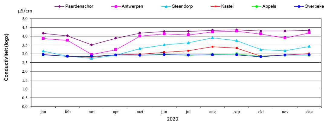
Figuur 5. Maandelijkse waarden (logx getransformeerd) van de conductiviteit ( \mu\text{Scm}^{-1} ) op zes plaatsen in het Zeeschelde-estuarium (www.vmm.be; meetdatabank 2020).
