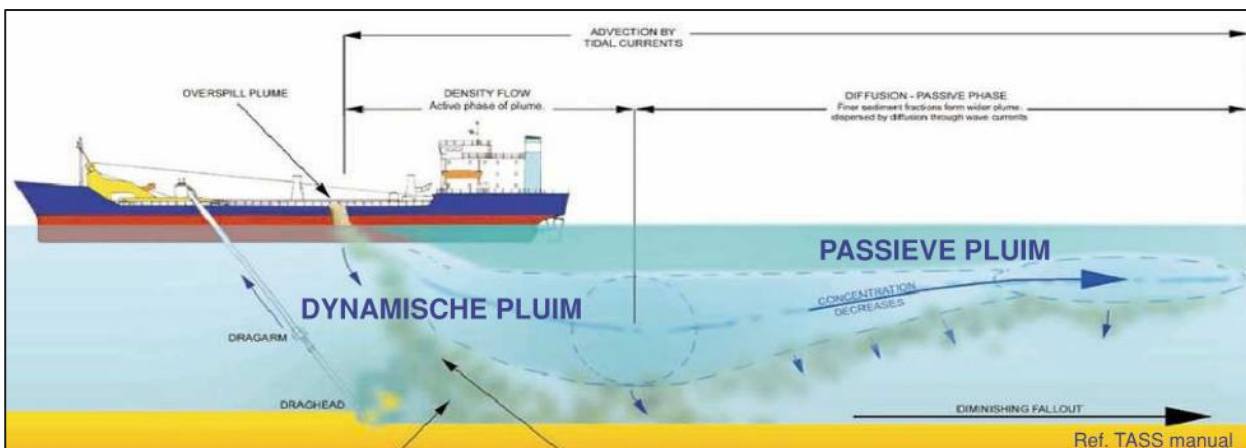
Figuur 5.2–7: Visualisatie dynamische en passieve pluim (Spearman et al. , 2011)
