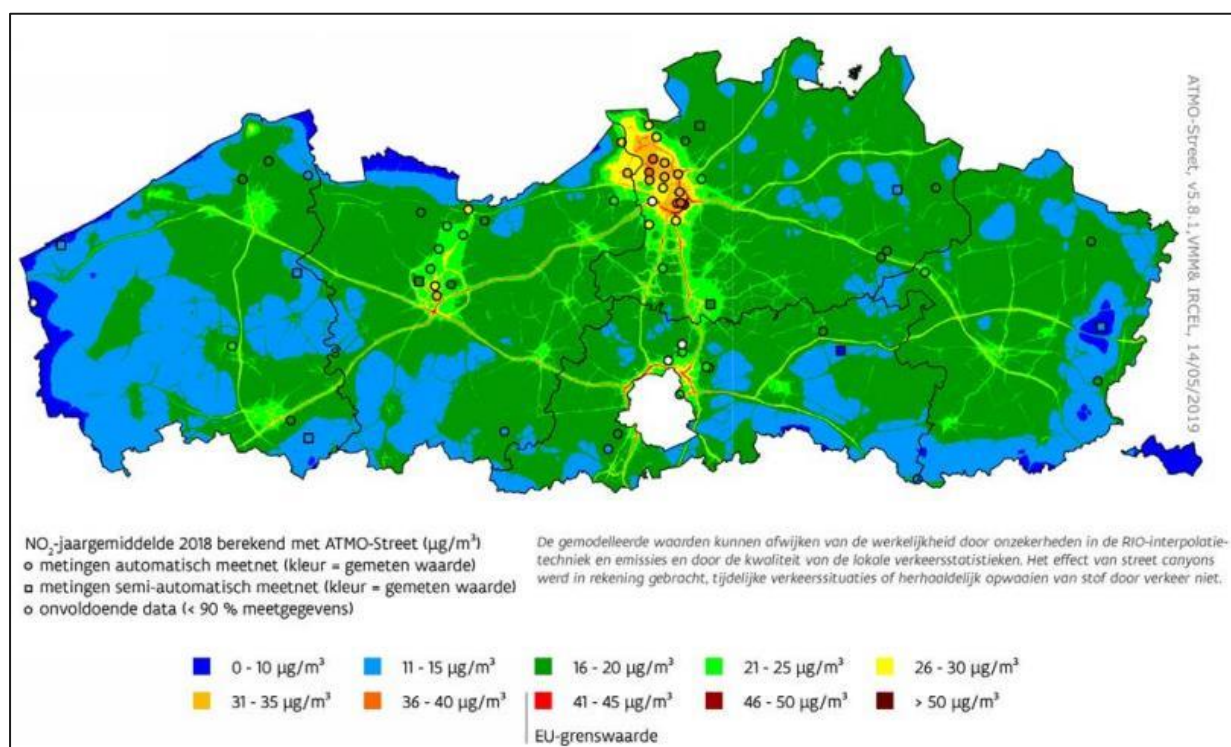
Figuur 5.4-2: Gemodelleerde NO 2 -jaargemiddelden in 2018 (Bron: VMM, 2019)
