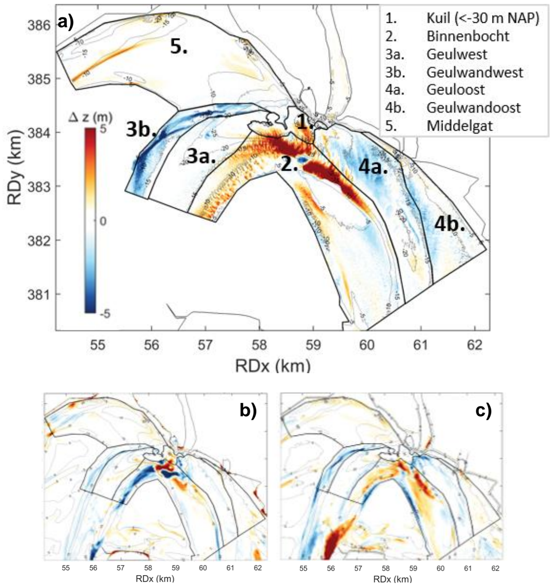
Figuur 3.6 Bathymetrische ontwikkeling van de Put van Hansweert na het plaatsen van de proefstortingen voor de periode van Maart 2016 tot April 2019 (paneel a) en voor de referentieperiodes voor en na stortingen bij het Gat van Ossenisse van 2002 tot 2005 (paneel b) en van 2011 tot 2014 (paneel c). (Huismans et al, 2020)
