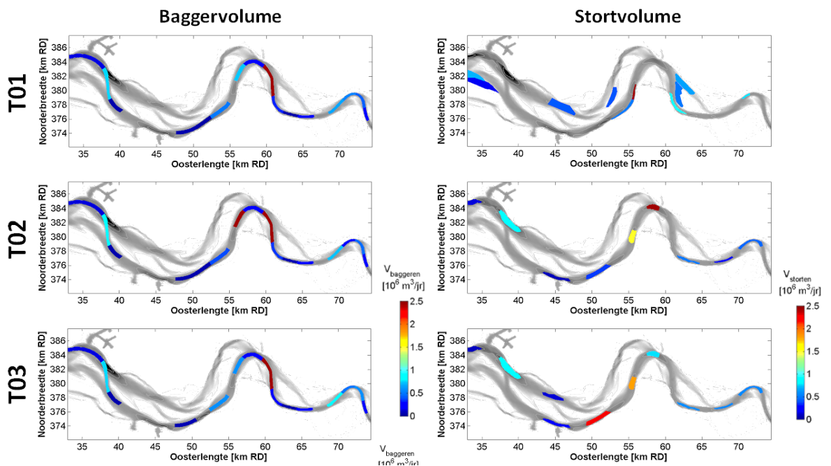
Figuur 3.9 Overzicht van bagger- en stortlocaties met bijbehorende stortvolumes voor strategie T01 t/m T03 op basis van modelresultaten voor het 'opgevulde putten' model (voor jaar 2). Deze figuren zijn bedoeld om een indicatief overzicht te geven van de locaties waar gestort en gebaggerd wordt (Huisman et al., 2018).
