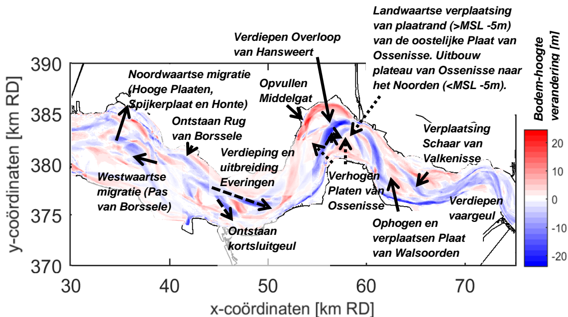
Figuur 2.8 Vershilplot bodemhoogte in de periode 1964 tot 2011 met karakteristieke ontwikkelingen (figuur uit Huisman et al., 2018 op basis analyse van Cleveringa, 2013).
