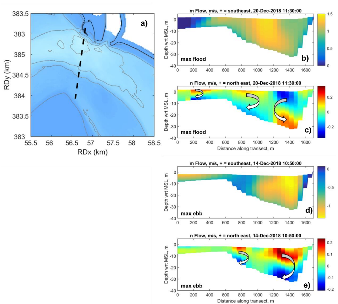
Figuur 2.3 Berekende stroomsnelheden in de Put van Hansweert op 20 December 2018 tijdens de vloed (paneel b en c) en eb fase (paneel d en e) (Van der Wegen et al., 2019).
