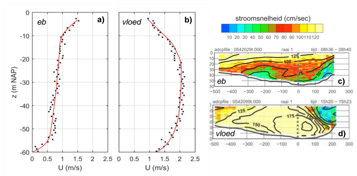
Figuur 2.4 Gemeten stroomsnelheden in de Put van Borssele voor 28 November 2011 (Van der Wegen et al., 2019)
