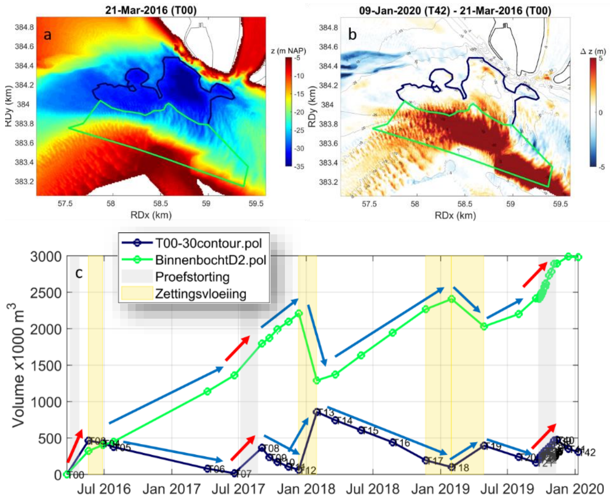
Figuur 3.3 Ontwikkeling van het volume in de Put van Hansweert en op de binnenbocht. Links-boven: Bodemhoogte in de diepe put van Hansweert; Rechts-boven : Bathymetrische verandering over de periode tussen 21 maart 2016 (T0) en 9 januari 2020 (T42); Onder: volumeverandering in de diepe put (zwarte lijn) en op de binnenbocht (groene lijn). Merk op dat er tijdens het storten een toename kan zijn in zowel de put als op de binnenbocht (rode pijlen) en dat er in de rest van de periode sprake is van een tegengestelde volumeontwikkeling van de put en de binnenbocht (blauwe pijlen). (bron : Huismans et al, 2020)
