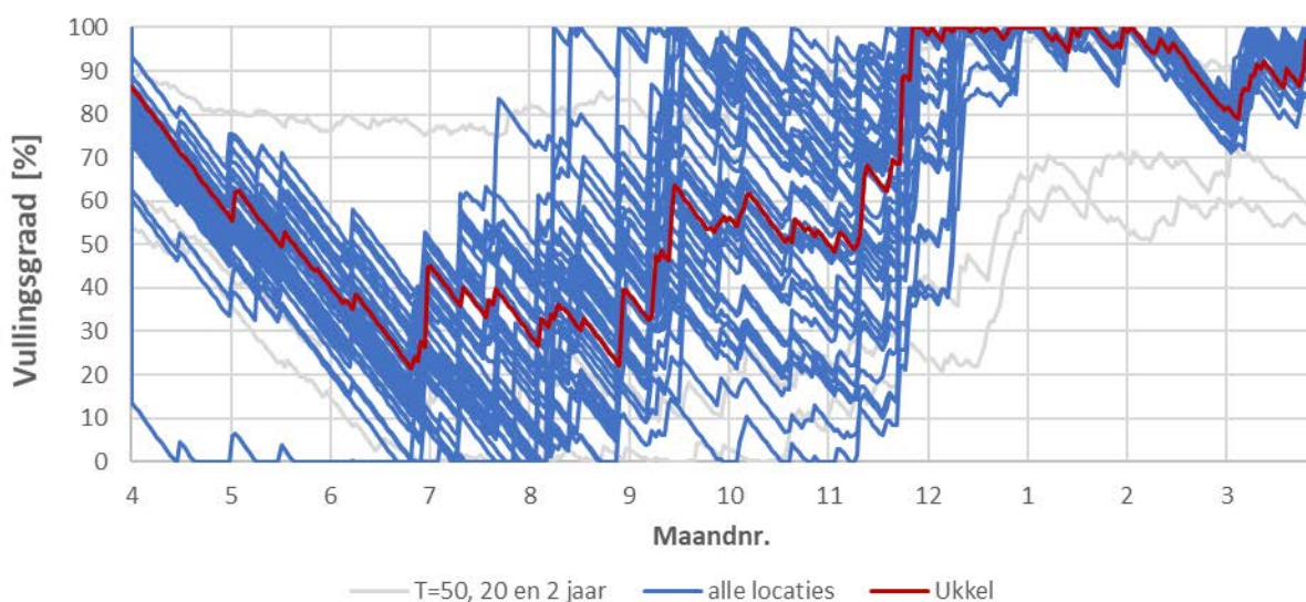
Figuur 109: % vullingsgraad voor een hemelwaterput met een capaciteit van 10 000 liter, voor een woning met een dakoppervlakte van 100 m 2 en een regenwaterverbruik van 100 liter/dag: resultaten voor alle waterinfo-pluviograaflocaties en het jaar 2017 en voor terugkeerperioden van 2, 20 en 50 jaar.
