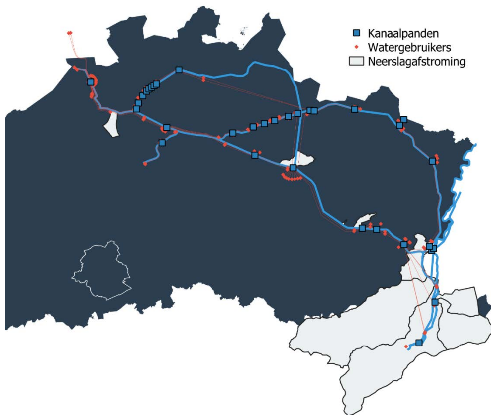
Figuur 225: Het beschouwde oppervlaktewatersysteem van Albertkanaal en Kempische kanalen, met aanduiding van de beschouwde kanaalpanden, de locaties van de beschouwde watergebruikers en de beschouwde neerslagafstromingsgebieden buiten Vlaanderen en de op- en afwaartse randen voor de Maas.
