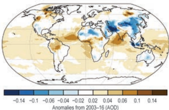
(z) Total Aerosol
