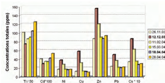
Figure 115. Évolution temporelle des teneurs métalliques dans le prodelta de la Têt. Les dates du 12/12/2003 et du 18/04/2006 correspondent aux prélèvements après des crues. Seule la première a donné lieu à un dépôt de sédiment frais au site étudié (emplacement de la bouée Poem-LR). Les concentrations métalliques, fortement liées aux teneurs en argile, diminuent après la crue de décembre qui va provoquer la remise en suspension de la fraction fine du dépôt, tandis que les concentrations en Ti augmentent, cet élément étant connu pour son association avec les silts (entre 2 et 63 µm).
