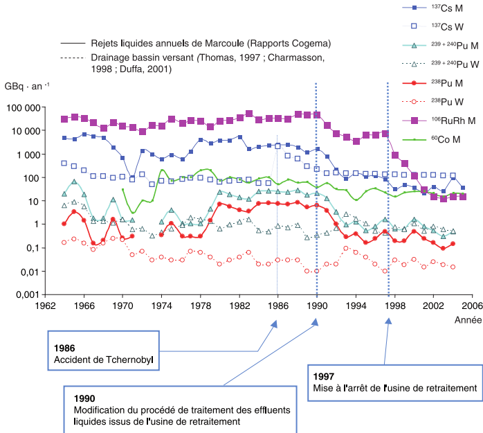
Figure 43. Chronique des apports annuels (en \text{GBq} \cdot \text{an}^{-1} ) dans les eaux du Rhône, depuis 1964, de radionucléides artificiels issus du drainage des sols du bassin versant (W) et des rejets de Marcoule (M).
