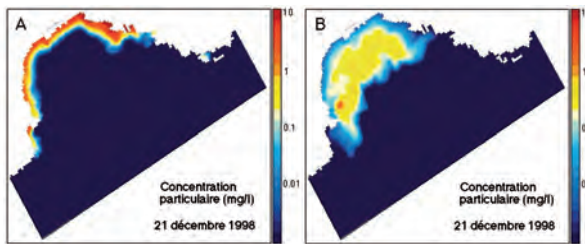
Figure 109. Simulations de la concentration particulaire près du fond pendant l'hiver 1998-1999. En A, le matériel particulaire provient uniquement de la resuspension naturelle du sédiment, provoquée par les vagues et les courants. En B, le matériel en suspension provient de l'activité d'une flottille de chalutiers. On note que dans le premier cas, seul le domaine proche du littoral est concerné ; dans le deuxième cas, l'impact est sensible sur le plateau externe, et plus particulièrement sur la partie sud du golfe, qui est la zone ayant la plus forte activité de pêche.
