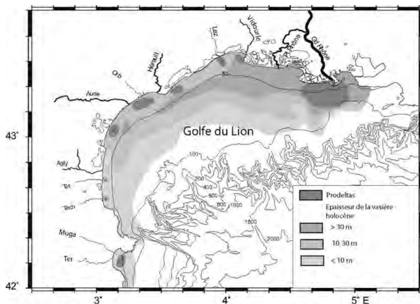
Figure 8. Carte morpho-sédimentaire du golfe du Lion montrant la répartition des prodeltas (zones de dépôt silto-argileux devant les fleuves) et de la vasière holocène sur le plateau (< http://cefrem.univ-perp.fr >). Les fleuves côtiers espagnols Muga et Ter, représentés sur la carte au sud de la zone, ne sont pas pris en compte dans les bilans de cette étude.
