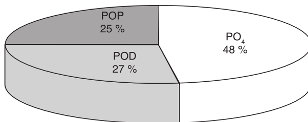
Figure 34. Répartition des différentes formes de phosphore (P) dans les eaux du Rhône : POP = phosphore particulaire, POD = phosphore organique dissous, PO 4 = orthophosphate.
