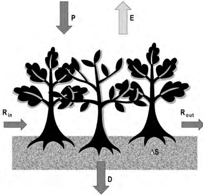
Figure 15. Termes du bilan hydrologique d'une parcelle agricole ou d'un écosystème terrestre. \Delta S est la variation de stock en eau du sol, P représente l'apport de précipitations sur la période considérée, R_{in} et R_{out} représentent respectivement le ruissellement en provenance des zones amont et le ruissellement exporté, E est l'évapotranspiration réelle et D le drainage profond.
