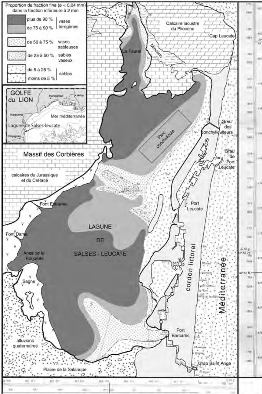
Figure 69. Carte sédimentologique de la lagune de Salses-Leucate (réalisée par R. Buscaill). In: cartes géologiques au 1/ 50 000 de Perpignan et de Leucate.
