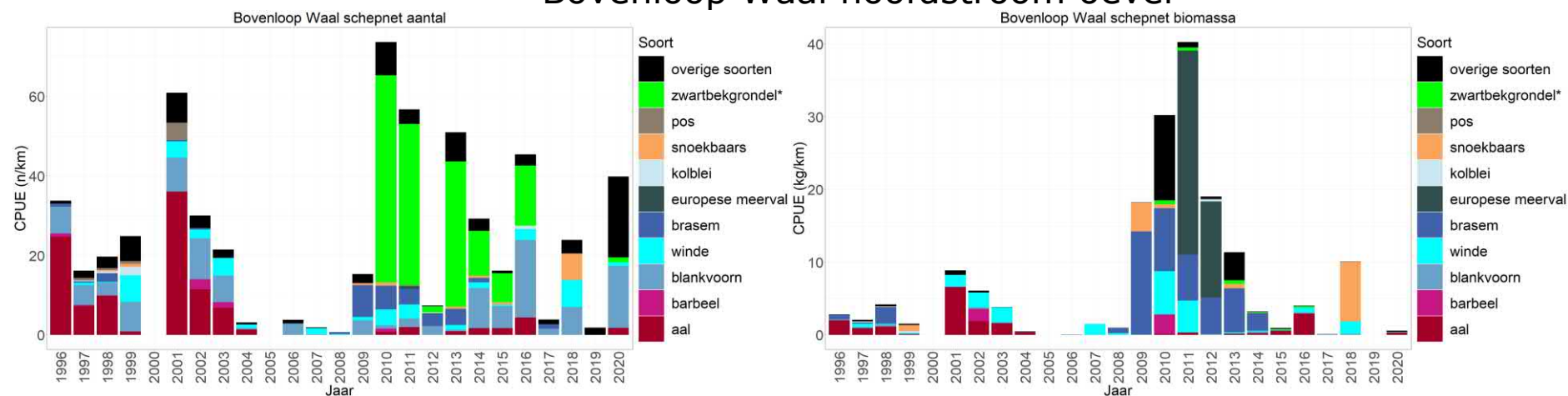
Figuur 2.90 Gemiddelde CPUE van de tien meest algemene vissoorten en overige vissoorten in het open water (n/ha-kg/ha bevist oppervlak) en langs de oever (n/km-kg/km bevist oppervlak) gevangen met een boomkor en electroschepnet in de hoofdstroom van de Bovenloop Waal tijdens de actieve monitoring van 1996-2020, * = exoot.
