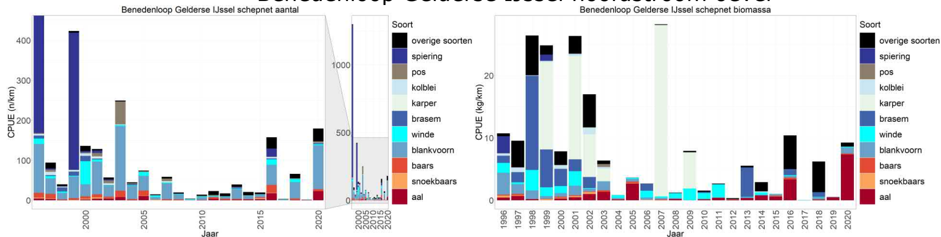
Figuur 2.66 Gemiddelde CPUE van de tien meest algemene vissoorten en overige vissoorten in het open water (n/ha-kg/ha bevist oppervlak) en langs de oever (n/km-kg/km bevist oppervlak) gevangen met een boomkor en electroschepnet in de hoofdstroom van de Benedenloop Gelderse IJssel tijdens de actieve monitoring van 1996-2020.
