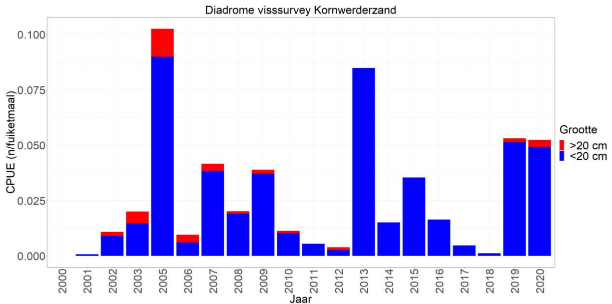
Figuur 4.11 Het gemiddelde vangstsucces (aantal per fuiketmaal) per jaar van Noordzeehouting in de diadrome vissurvey Kornwerderzand (zoute zijde).
