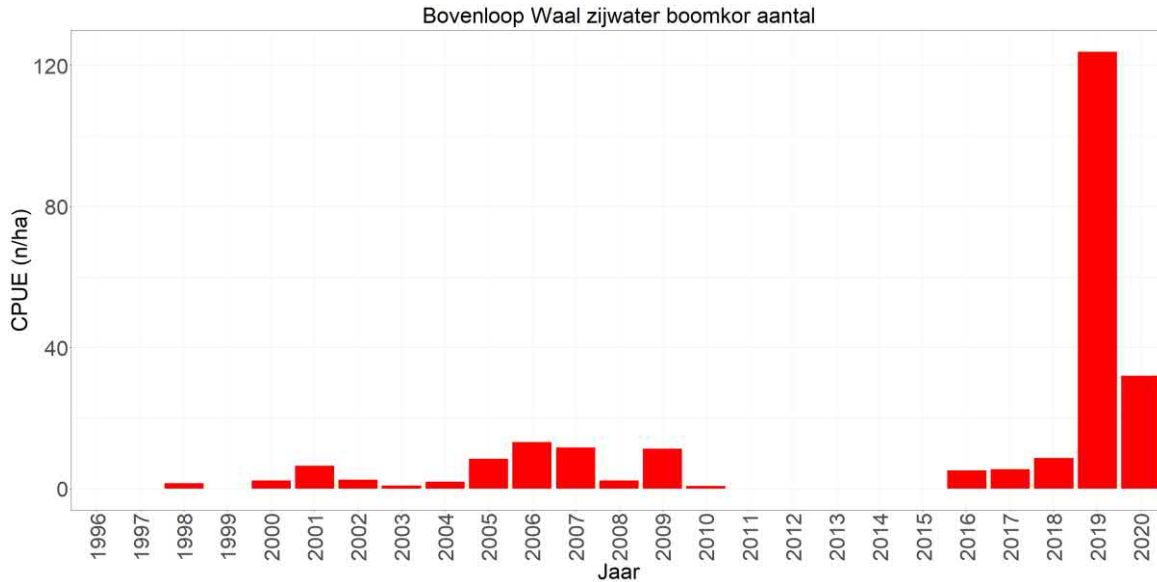
Figuur 2.94 Gemiddelde CPUE (n/ha bevist oppervlak) per jaar van de Chinese wolhandkrab in de zijwateren van de Bovenloop Waal gevangen met de boomkor.
