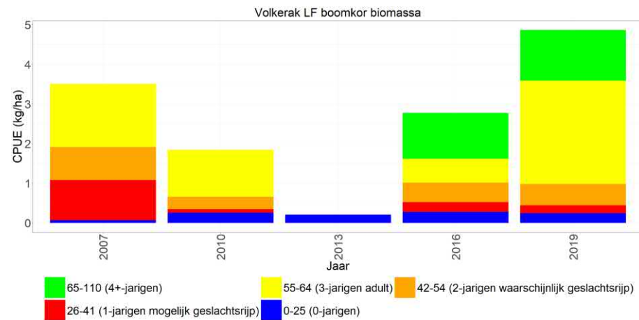
Figuur 4.70 Gemiddelde CPUE (n/km-n/ha en kg/km-kg/ha bevistoppervlak) per jaar met lengteverdeling (cm) van snoekbaars gevangen met de boomkor in het open water en met het electroschepnet langs de oevers van de Volkerak.
