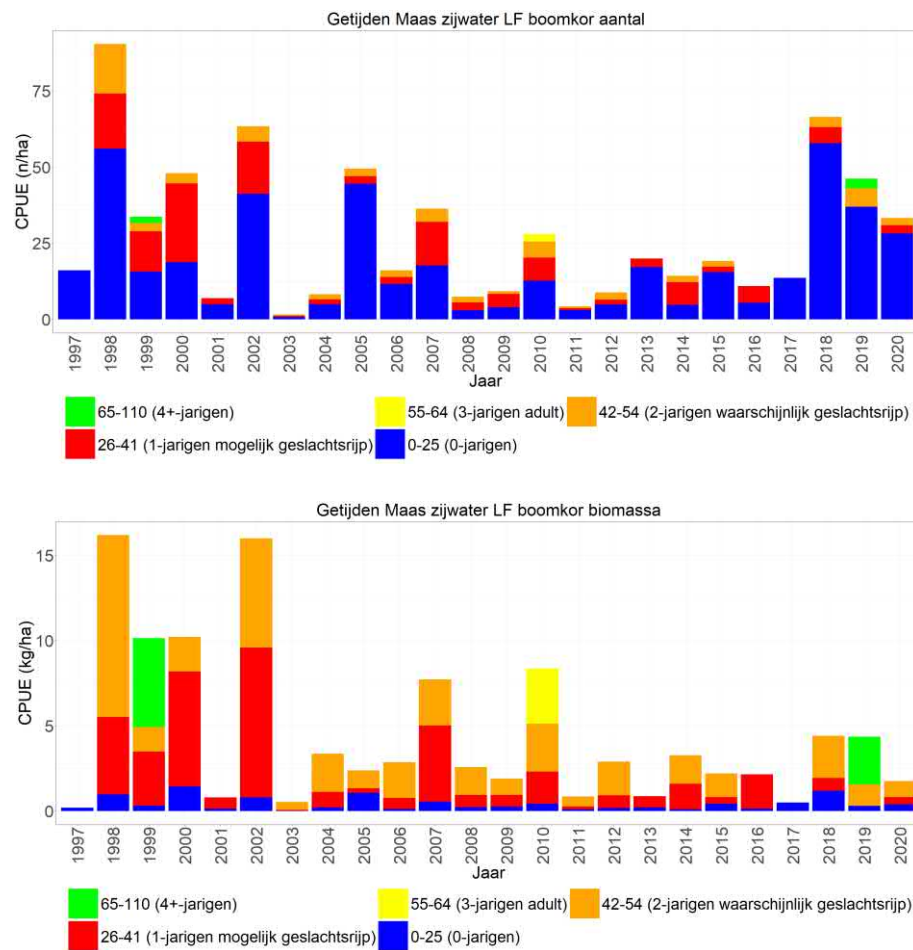
Figuur 4.58 Gemiddelde CPUE (n/km-n/ha en kg/km-kg/ha bevistoppervlak) per jaar met lengteverdeling (cm) van snoekbaars gevangen met de boomkor in de zijwateren en met het elektroscopnet langs de oevers van de Getijden Maas.
