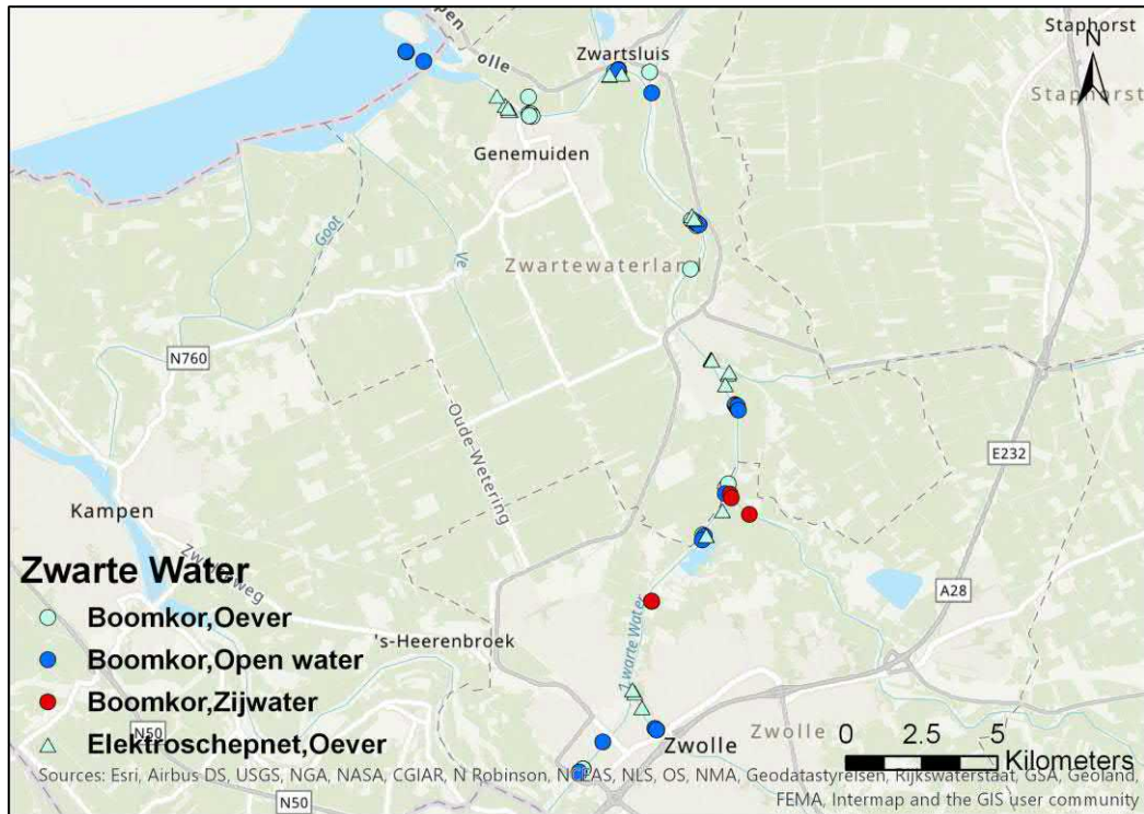
Figuur 2.60 Bemonsteringslocaties van de actieve monitoring in de Zwarte Water van 2010-2019 per tuig per habitat.
