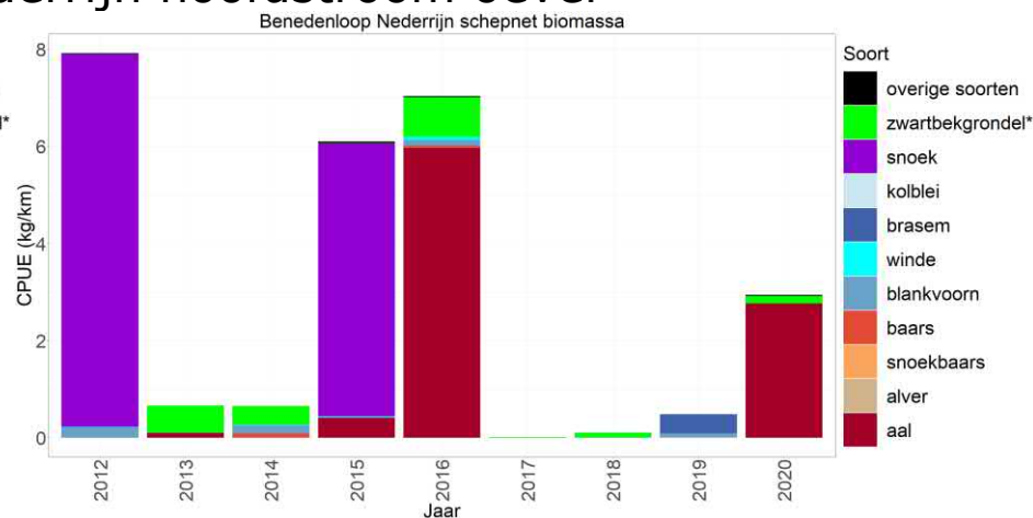
Figuur 2.135 Gemiddelde CPUE van de tien meest algemene vissoorten en overige vissoorten in het open water (n/ha-kg/ha bevist oppervlak) en langs de oever (n/km-kg/km bevist oppervlak) gevangen met een boomkor en electroschepnet in de hoofdstroom van de Benedenloop Nederrijn tijdens de actieve monitoring van 2012-2020, * = exoot.
