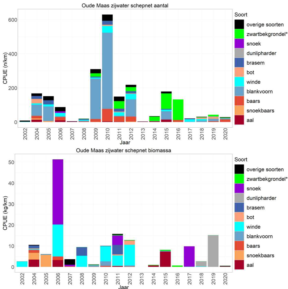
Figuur 2.145 Gemiddelde CPUE van de tien meest algemene vissoorten en overige vissoorten langs de oever (n/km-kg/km bevist oppervlak) gevangen met een electroschepnet in zijwateren van de Oude Maas tijdens de actieve monitoring van 2002-2020, * = exoot.
