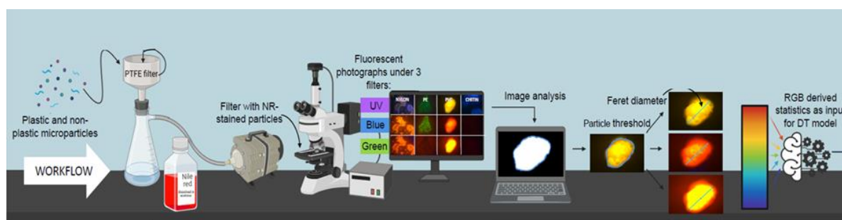
Figuur 2. Werkwijze voor de analyse van micro-partikels opgesteld door het ANDROMEDA consortium ( Meyers et al., 2022 )
