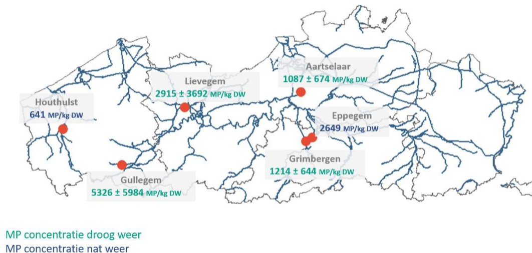
Figuur 5. Microplastic concentraties in het sediment voor de staalnamelocaties uit de studie Vercauteren et al. (2021) . Om de distributie van microplastics in zoetwatermilieus in Vlaanderen te bestuderen werden zowel concentraties gemet bij perioden met minder (droog weer) als meer (nat weer) regenval.
