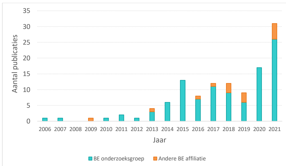
Figuur 10. Aantal geselecteerde A1 publicaties (WoS) per jaar van publicatie, geaffiliëerd aan een Belgische universitaire associatie of wetenschappelijke instelling (turquoise), en met overige Belgische affiliatie (oranje). Het jaar 2022 werd niet opgenomen in de figuur.
