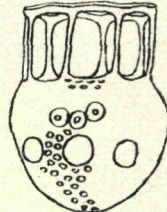
Fig. 30. Dictyoecysta lepida Ehrbg. — 300:1; Mittel- meer. — Struktur des Wohnfaches nur ange- deutet; in der Mitte 3 Kokkolithen.
