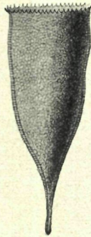
Fig. 16. Favella denticulata typicala Jörg., (Ehrbg.) Jörg. kleine Form; 300:1, Bergen.
