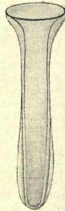
Fig. 13. Amphorella steenstrupi (Clap. & Lachm.) Dad.
