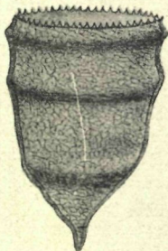
Fig. 24. Ptychocyliis urnula (Clap. & Lachm.) Bdt. var. minor Jörg. Beide von Bergen; 300:1.
