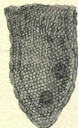
Fig. 22. Coxiella pseudannulata Jörg. — 300:1; Norwegische See.
