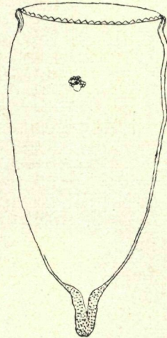
Fig. 17. Favella serrata (Möb.) Jö-z. 300:1; Barcelona. Mündungszähne nur vorn, die zwei Wandlamellen nur oben abgebildet, die Wandstruktur nur angedeutet.
