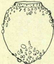
Fig. 6. Stenosemella ventricosa (Clap. & Lachm.) Jörg.
