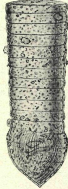
Fig. 4. Tintinnopsis tubulosa var. subacuta (Jörg.). 300:1; Bergen.
