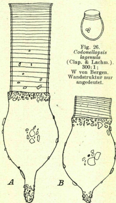
Fig. 27. Codonellopsis orthoceras Haeck. A 300:1; Mittelmeer. B Ein Individuum mit kürzerem Fortsatz und Aufsatz, letzterer höchst- wahrscheinlich noch unvollendet; Belag nur angedeutet.
