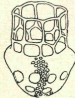
Fig. 29. Dictyoecysta elegans Ehrbg. var. speciosa Jörg. 300:1; Mittelmeer. Struktur des Wohn- faches nur längs der Mitte vollstän- dig dargestellt.
