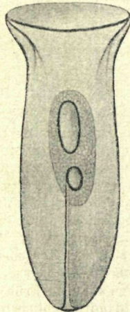
Fig. 12. Amphorella quadrilineata (Clap. & Lachm.) Jörg.
