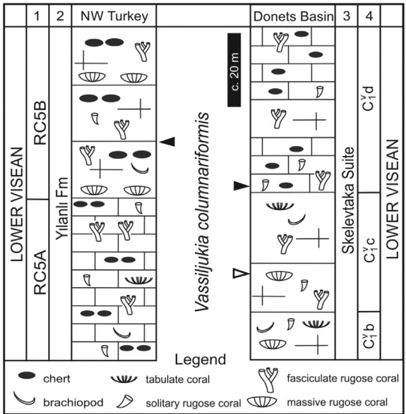
Fig. 2. Schematic lithostratigraphic succession of the Lower Visean in NW Turkey and the Donets Basin with stratigraphic position of Vassiljukia columnariformis (holotype: white arrow, and additional material: black arrows). Modified after Denayer (2014) and Ogar (2010). Column heads: 1: substages; 2: rugose coral zones (after Denayer, 2014); 3: formations; 4: subzones. Fig. 2. Succession lithostratigraphique schématique du Viséen inférieur de la Turquie du Nord-Ouest et du bassin du Donetz, avec position stratigraphique de l’holotype (flèche blanche) et spécimens additionnels (flèches noires) de Vassiljukia columnariformis . Modifié d’après Denayer (2014) et Ogar (2010); intitulé des colonnes: 1: Sous-étage; 2: zones à coraux rugueux (d’après Denayer, 2014); 3: formations; 4: Sous-zones.
