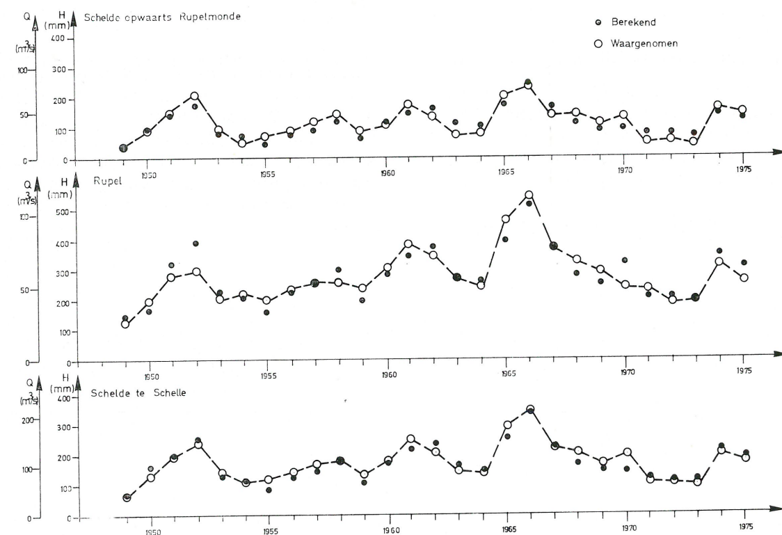
Fig. 10. — Waargenomen en berekende afvoer-(jaargemiddelden.)
