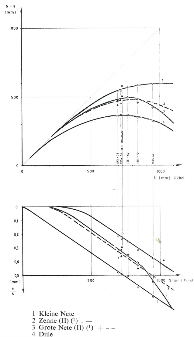
Fig. 4. — Gemiddelde neerslag-afvoerrelaties.
