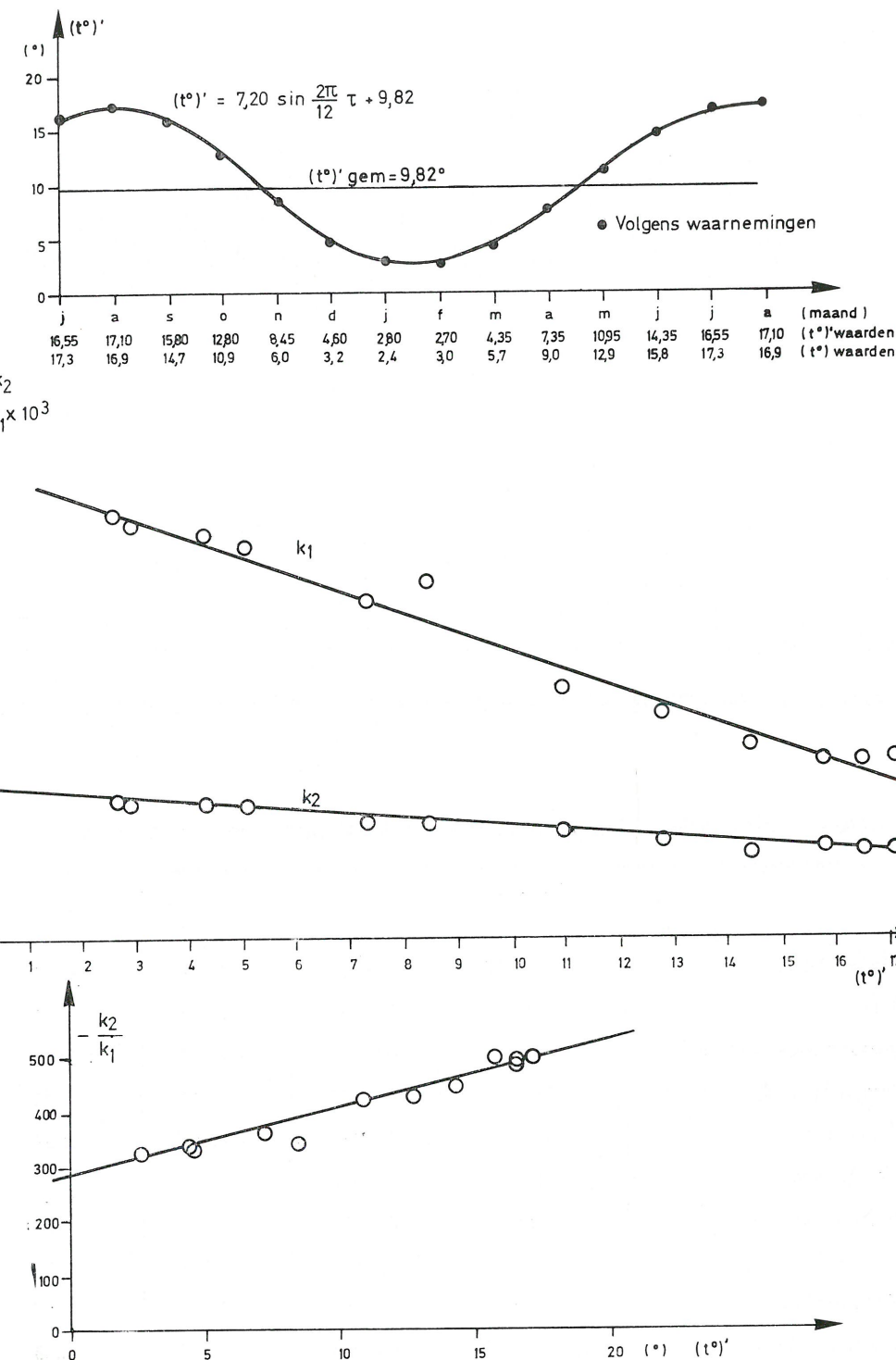
Fig. 32. — Verloop van maandgemiddelde representatieve temperatuur (t^\circ)' en van k_1 , -k_2 en -\frac{k_2}{k_1} in functie van (t^\circ)' .
