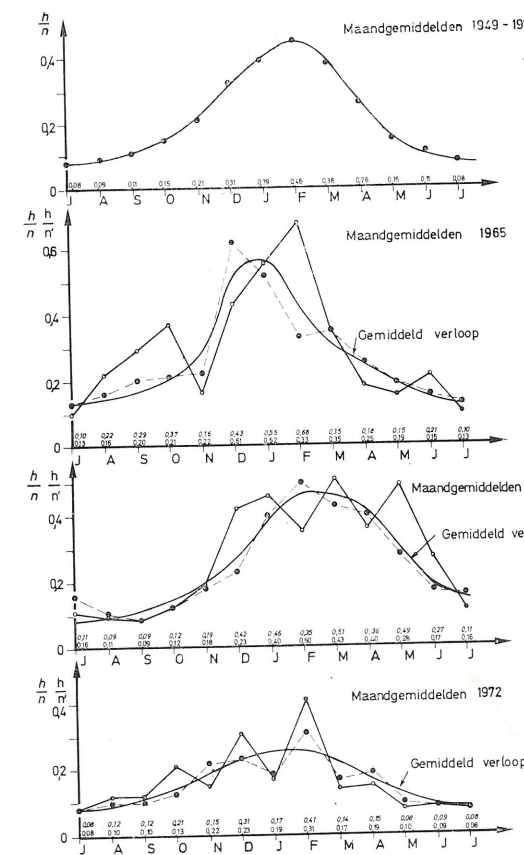
Fig. 12. — Afvoercoëfficiënten Schelde te Schelle — maandgemiddeld verloop voor verschillende perioden. (streeplijn: \frac{h}{n'} )
