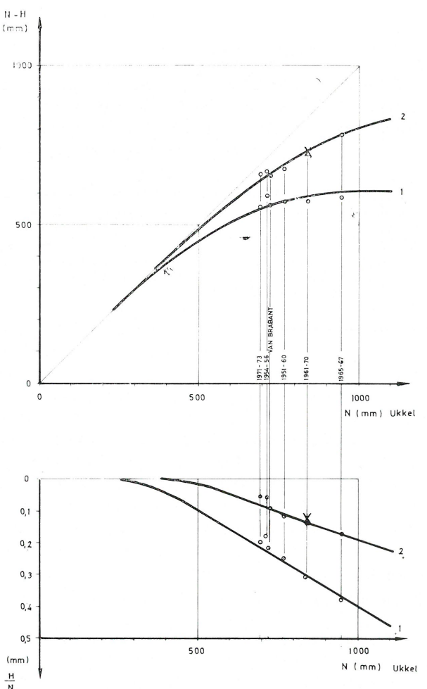
Fig. 5. — Gemiddelde neerslag-afvoerrelaties.
