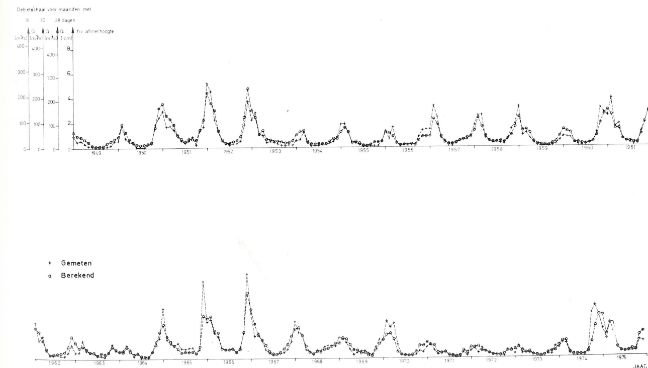
Fig. 27. — Waargenomen en berekende afvoer met neerslag over Vlaanderen voor Schelde opwaarts Rupel.
