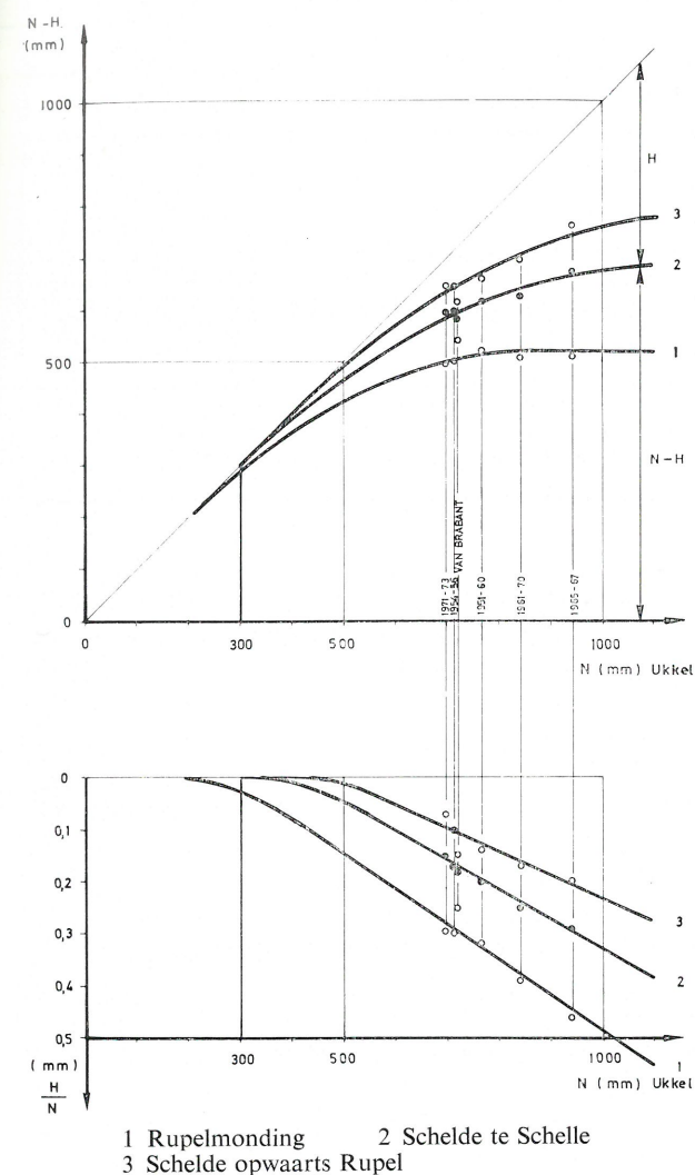
Fig. 3. — Gemiddelde neerslag-afvoerrelaties.
