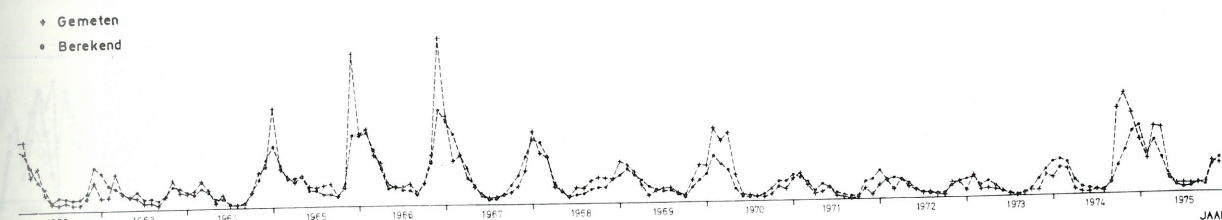
Fig. 18. — Waargenomen en berekende afvoer met neerslag te Ukkel voor Schelde opwaarts Rupel.
