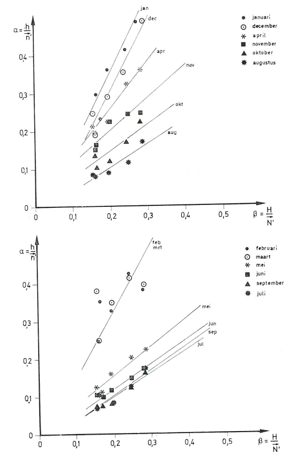
Fig. 13. — Maandgemiddelde afvoercoëfficiënt in functie van meerjaarlijkse afvoercoëfficiënt.
