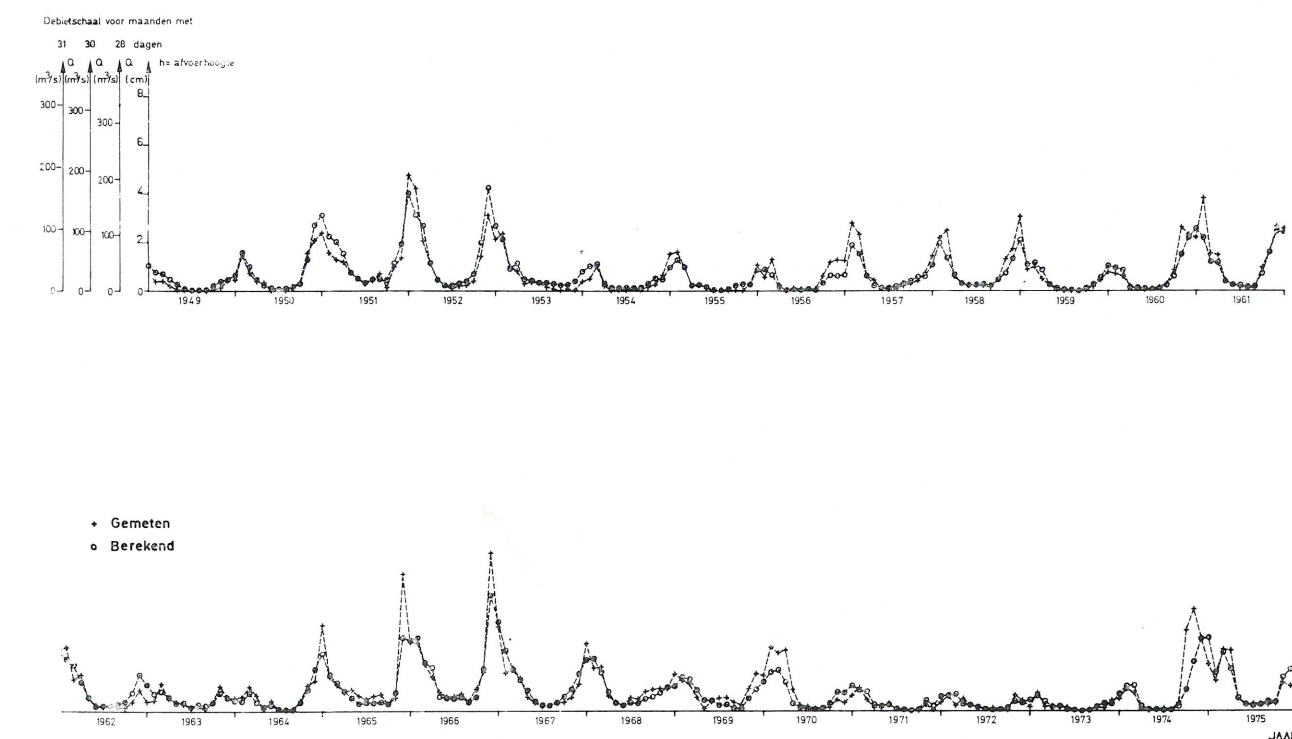
Fig. 39. — Waargenomen en berekende afvoer met afvoer-neerslag-temperatuurformule uitgaande van neerslag over Vlaanderen voor Schelde te Gent (en Merelbeke).
