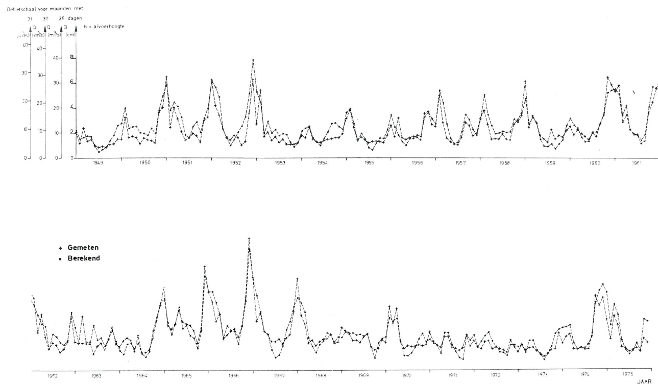
Fig. 36. — Waargenomen en berekende afvoer met afvoer-neerslag-temperatuurformule uitgaande van neerslag te Ukkel voor Zenne (II).
