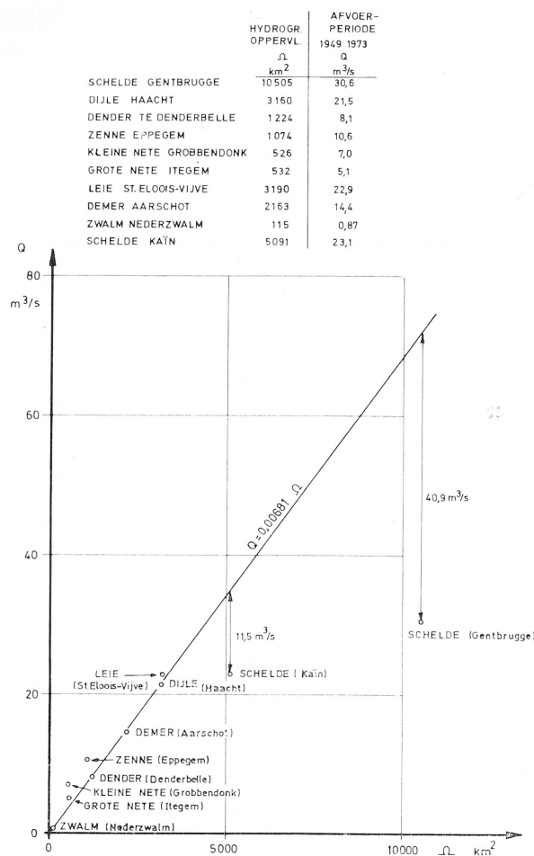
Fig. 6. — Afvoer in functie van hydrografisch oppervlak (1949-1973).
