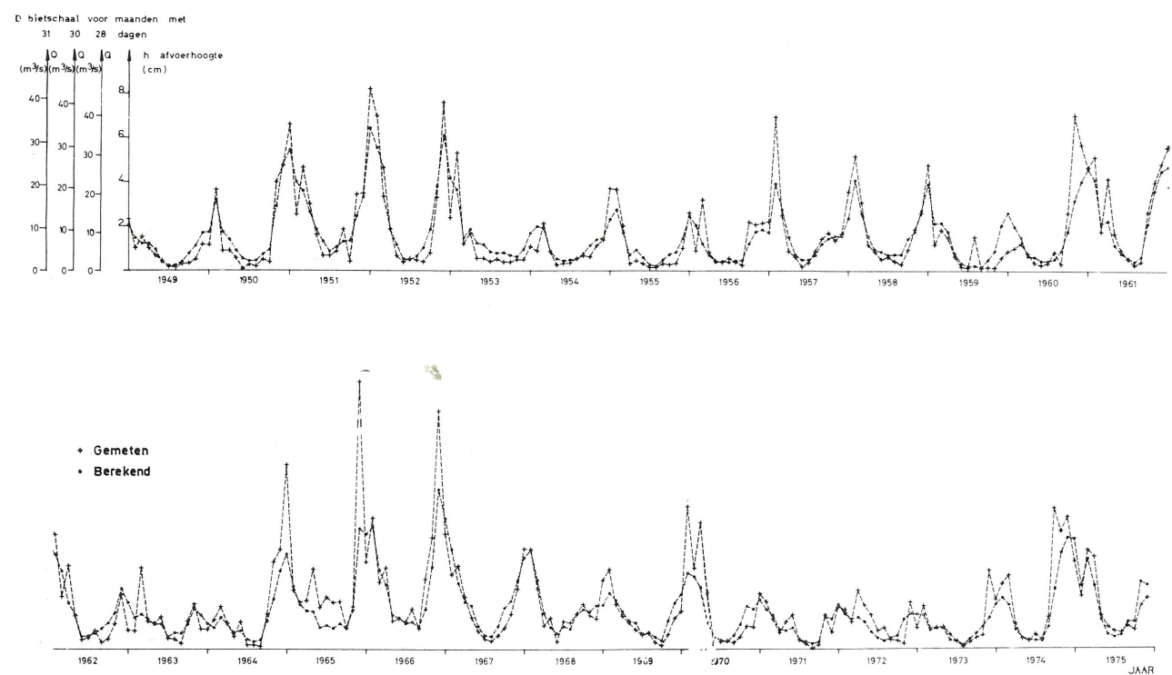
Fig. 37. — Waargenomen en berekende afvoer met afvoer-neerslag-temperatuurformule uitgaande van neerslag over Denderbekken voor Dender (monding).
