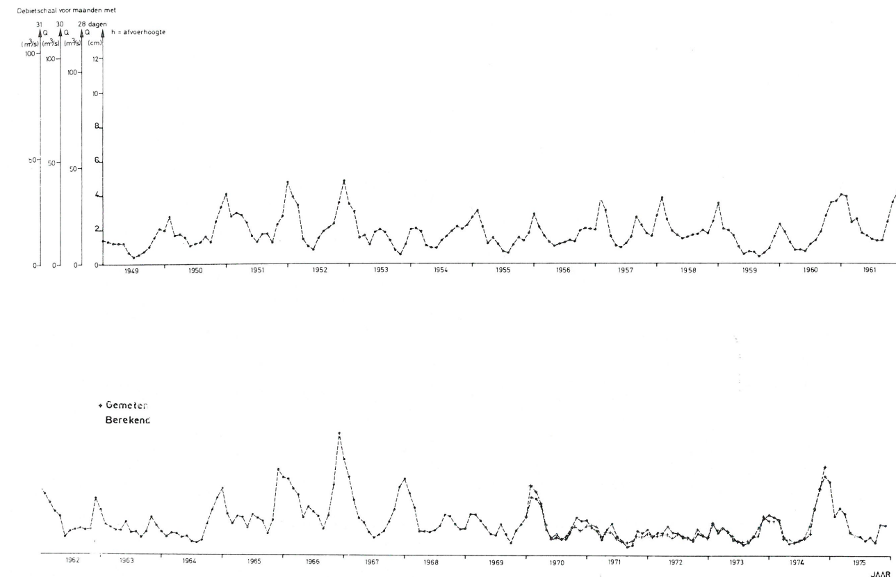
Fig. 42. — Waargenomen en berekende afvoer met afvoer-neerslag-temperatuurformule uitgaande van neerslag over Kempen voor Demer te Aarschot (alleen uitgegaan van neerslag over januari en juli 1973 voor bepaling van de coëfficiënten a, b, c, en d).
