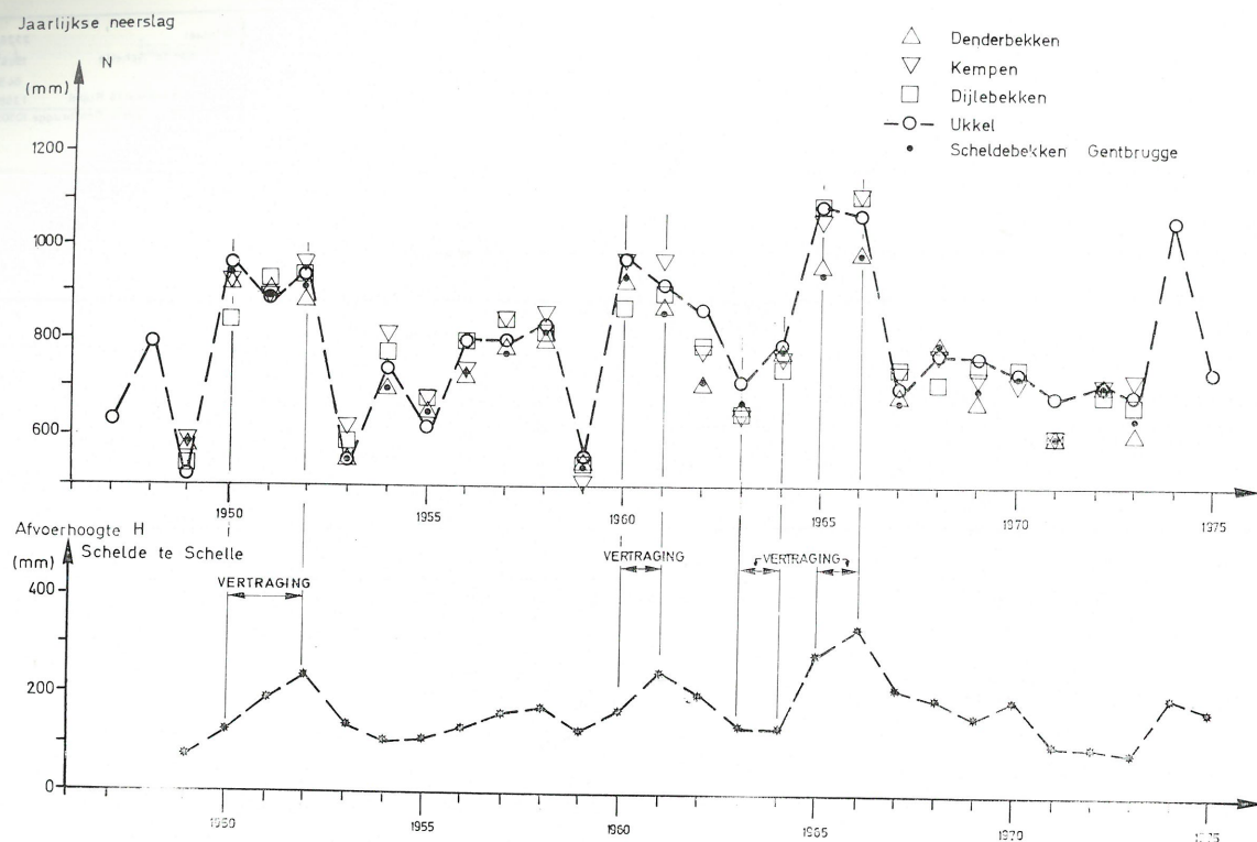
Fig. 2. — Jaargemiddeld neerslag- en afvoerloop.
