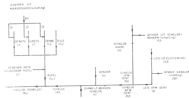
Fig. 7. — Gemiddeld afvoerbilan (m³/s).
