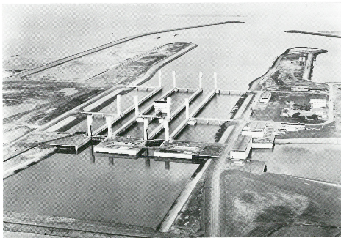
Photo 6. — Vue d'ensemble de l'écluse du Kreekrak. (Photo Barthofmeester - Rotterdam).
