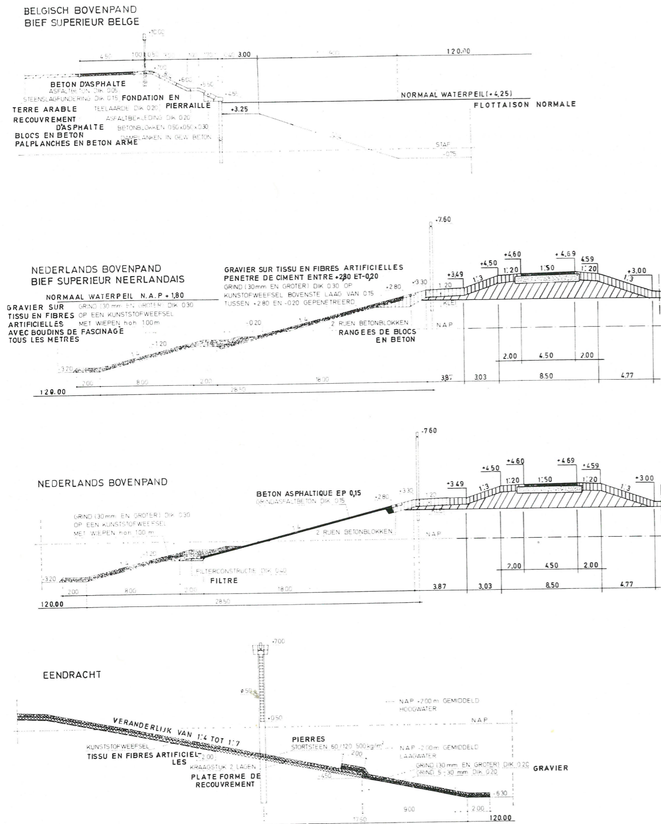
Fig. 4. — Consolidations de talus.
