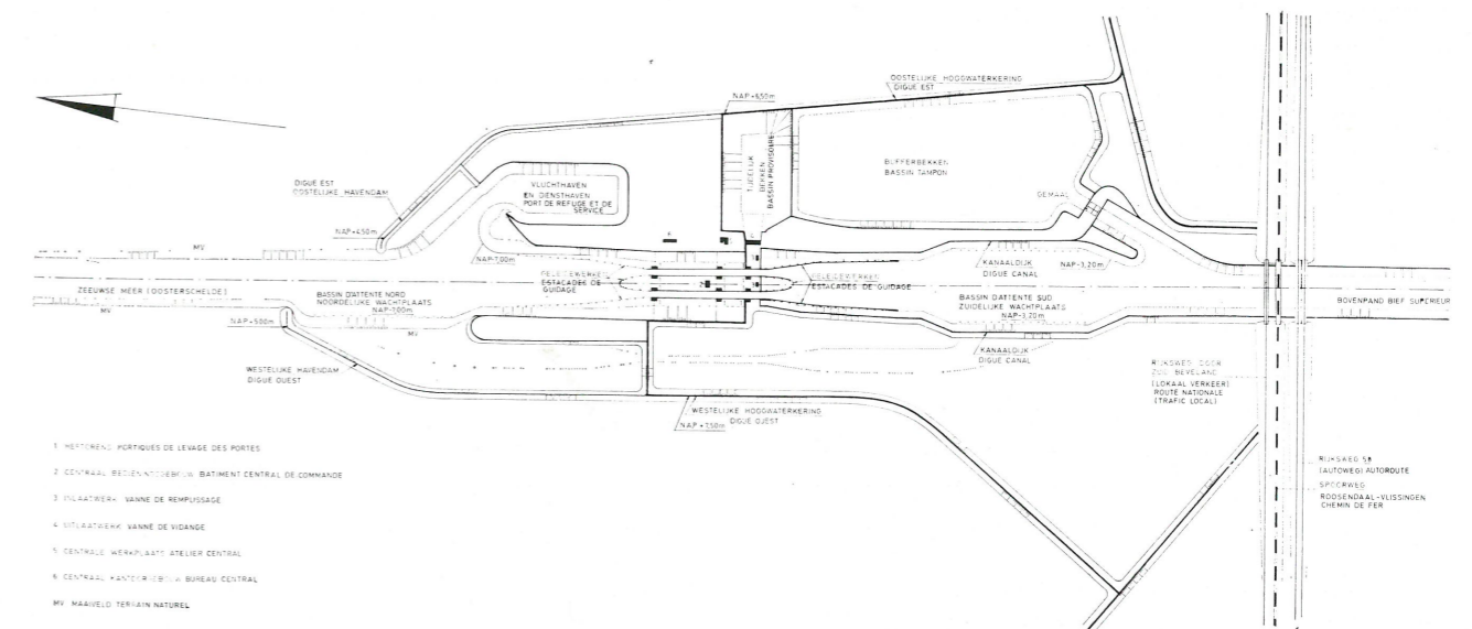
Fig. 5. — Plan de situation schématique des écluses du Kreekrak.
