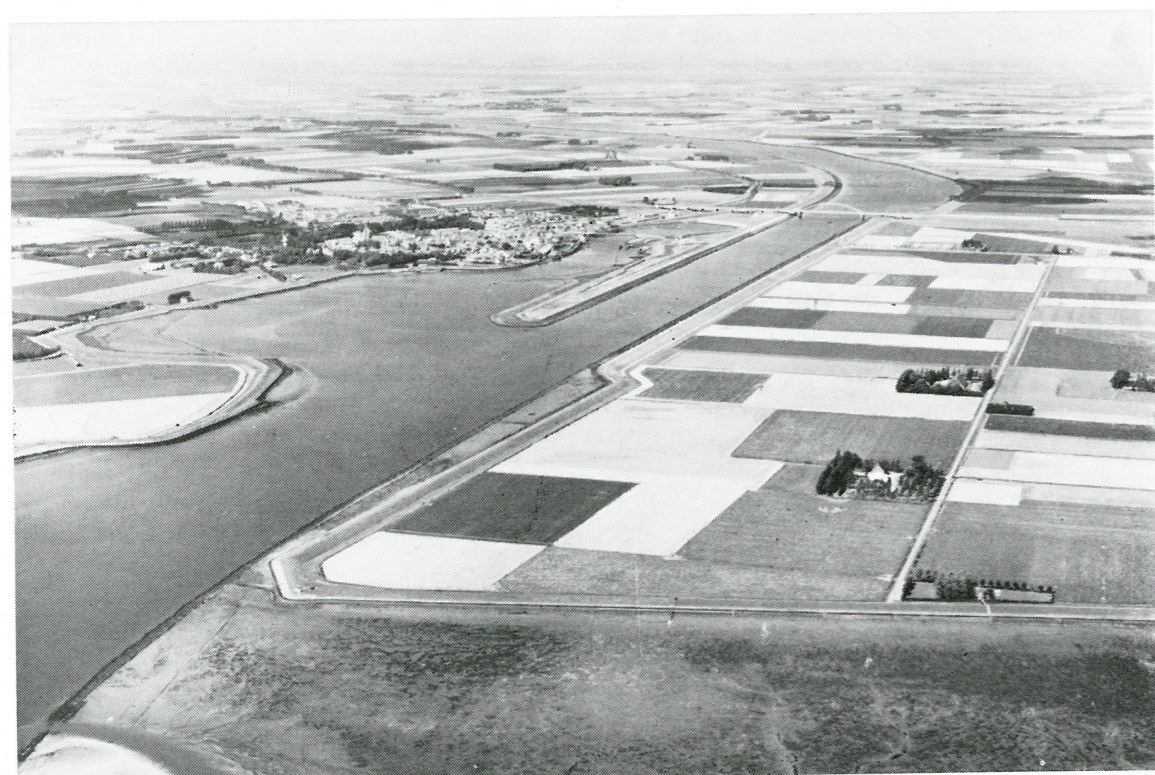
(Photo Barthofmeester - Rotterdam). Photo 4. — Bief inférieur dans l'Eendracht avec à l'avant-plan l'Escaut oriental et au centre le village et le pont de Tholen.
