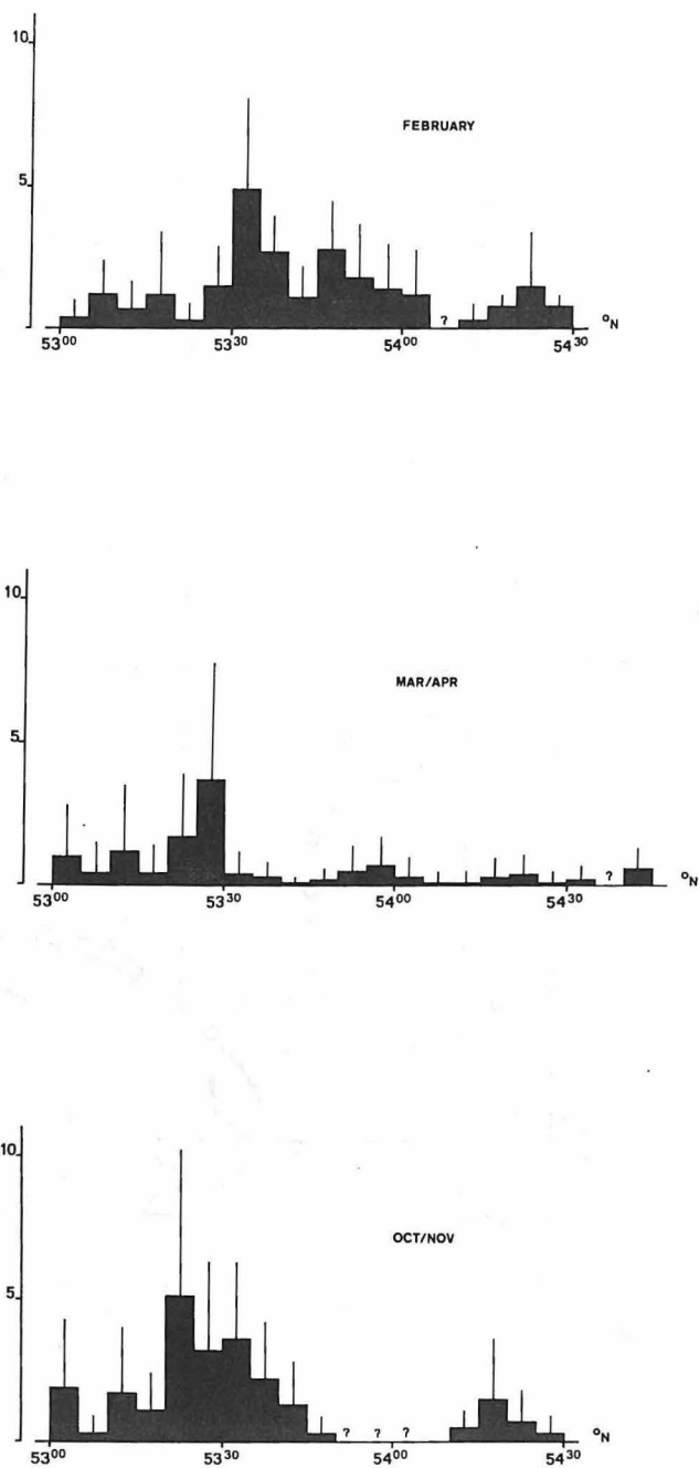
Fig. 15. Voorkomen van Zeekoeten in gemiddelde aantallen (blokken) met standaard deviaties (lijnen) per 10 observatie minuten, gerangschikt per 5 minuten NBr. A: februari. B: maart/april. C: oktober/november. Stippellijnen in C geven de gemiddelde aantallen, wanneer de tellingen van het kustwater in deze periode niet worden meegerekend.
