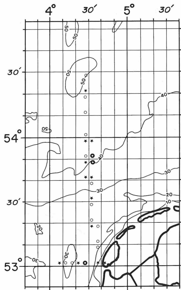
Fig. 13. Alk in februari. \circ : geen Alken aangetroffen. \star : < 0,50 Alk per telling van 10 minuten. \bullet : > 0,50 Alk per telling.
