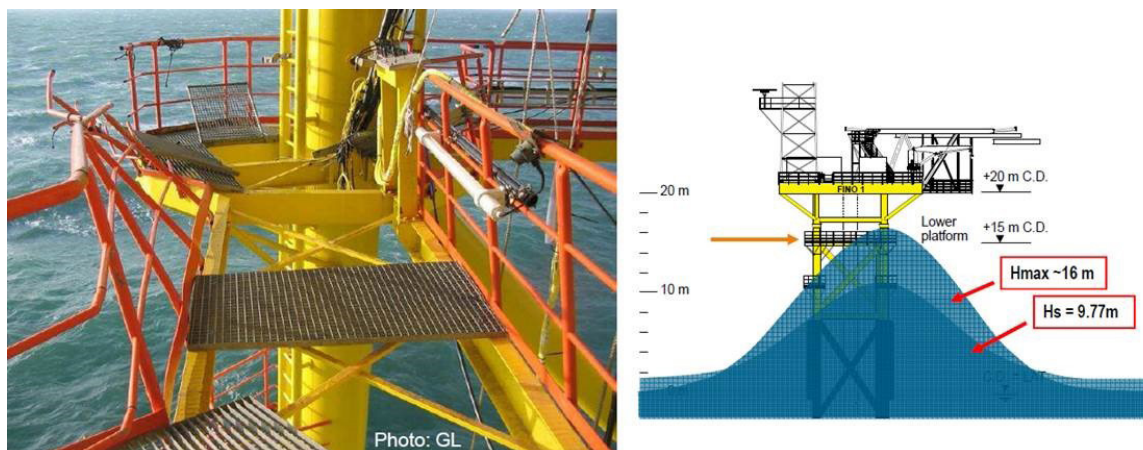
Figuur 10: (Links) Foto van de schade aan het FINO1 offshore platform als gevolg van rogue waves tijdens storm Britta (4/10/2009). (Rechts) Illustratie van de rogue wave in kwestie. Bron: DNV GL 2009.
