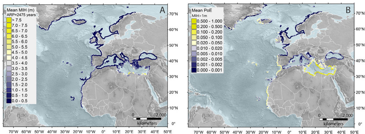
Figuur 5: (A) NEAMTHM18-gevaarkaart met weergave van de gemiddelde maximale inundatiehoogte (opzet) met een terugkeerperiode van 2.475 jaar en (B) NEAMTHM18-waarschijnlijkheidskaart voor een maximale inundatiehoogte groter dan 1 m op 2.475 jaar. Topo-bathymetrie is afkomstig van het ETOPO1 Global Relief Model (NOAA 2009, Amante en Eakins 2009). Bron: Basili et al. (2021).
