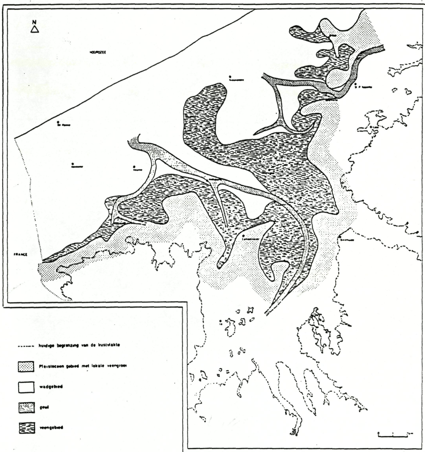
Figuur 1.19c : Paleografie van de kustvlakte omstreeks 3500 v.C. (Baeteman, 1981).
