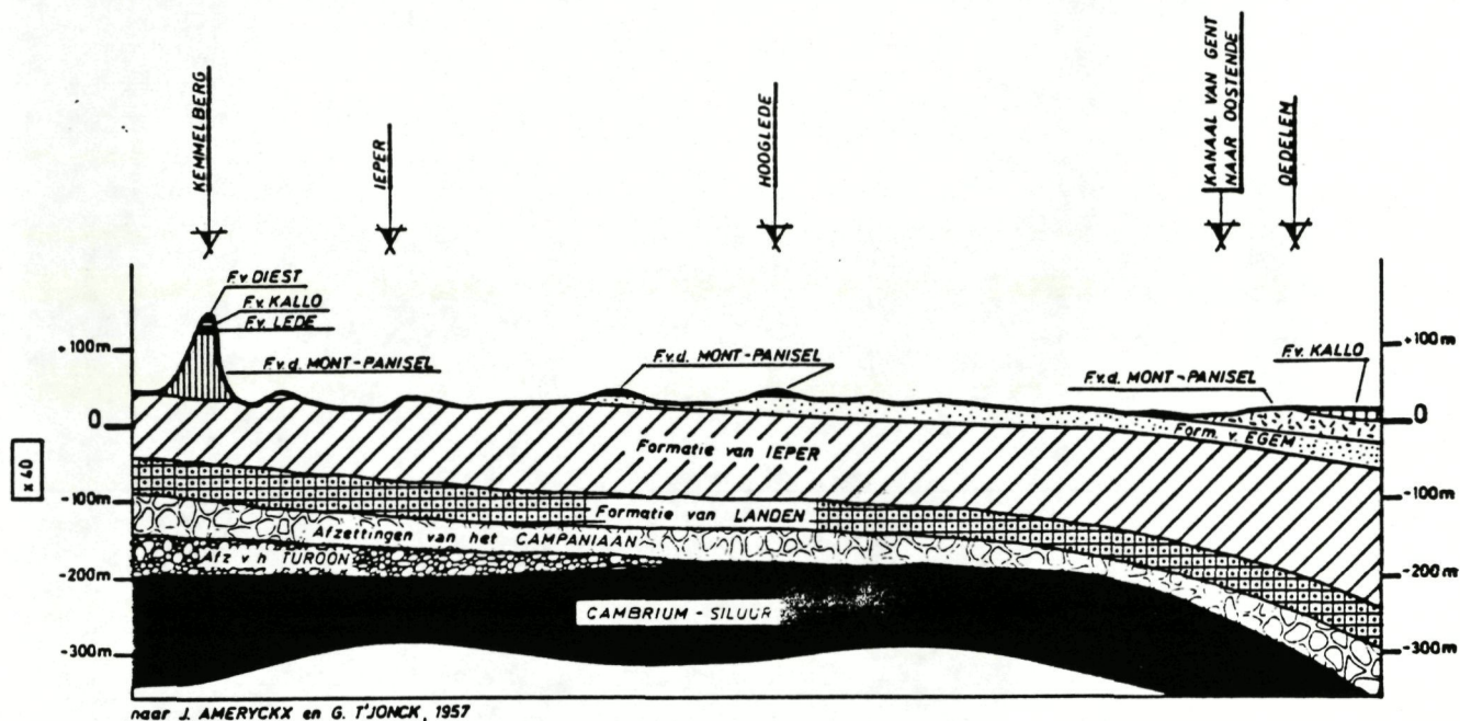
Figuur 1.6 : Geologisch profiel Kemmelberg - Oedelem (BAETEN, 1987).
