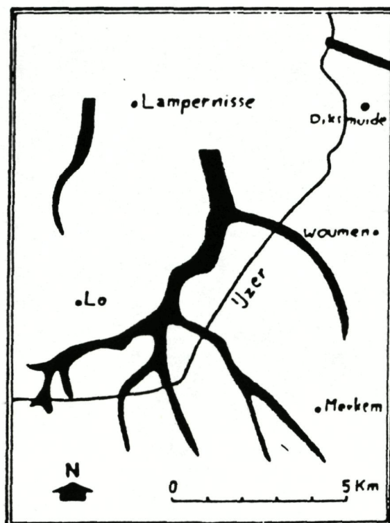
Figuur 1.17 : Het postglaciair valleienstelsel in de omgeving van Lo (MARECHAL, 1953).
