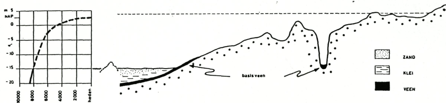
Figuur 1.18b : Enkele stappen uit het opvullingsproces van de kustvlakte : omstreeks 6000 jaar v.C. (BAETEMAN, 1987).
