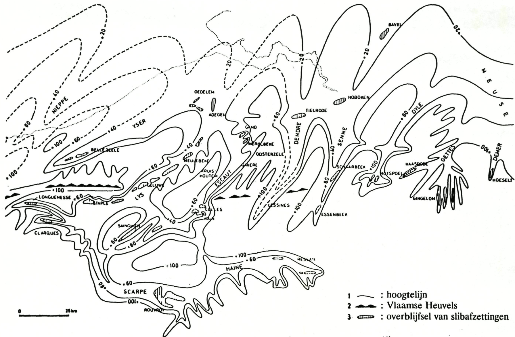
Figuur 1.9 : Reconstructie van de veralgemeende hoogtelijnen in het Scheldebekken op het einde van het Midden-Pleistoceen (TAVERNIER & DE MOOR, 1974).
