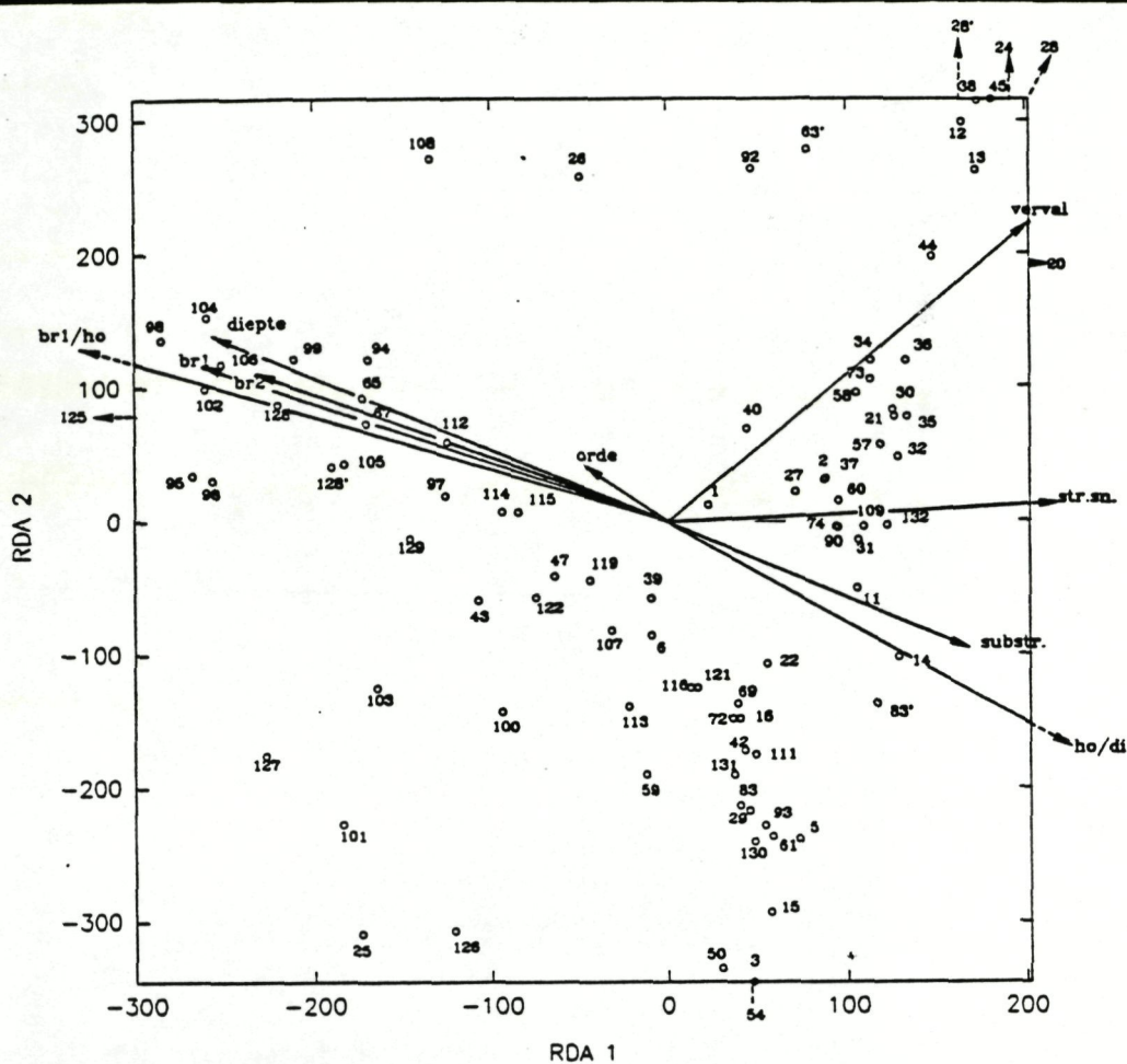
figuur 3.5 A : Inventarisatiepunten en morfometrische variabelen uitgezet volgens de eerste en de tweede as van de RDA-ordinatie diagram.
