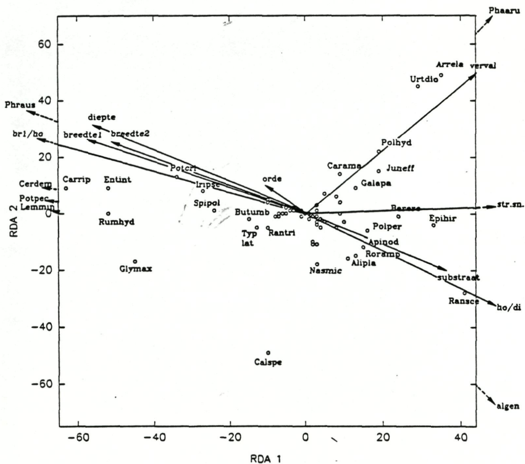
Figuur 3.5 B : Waterplanten en morfometrische variabelen uitgezet volgens de eerste en de tweede as van de RDA-ordinatie diagram. Enkel de soorten die bepalend zijn voor de samenstelling van de assen zijn weergegeven.
