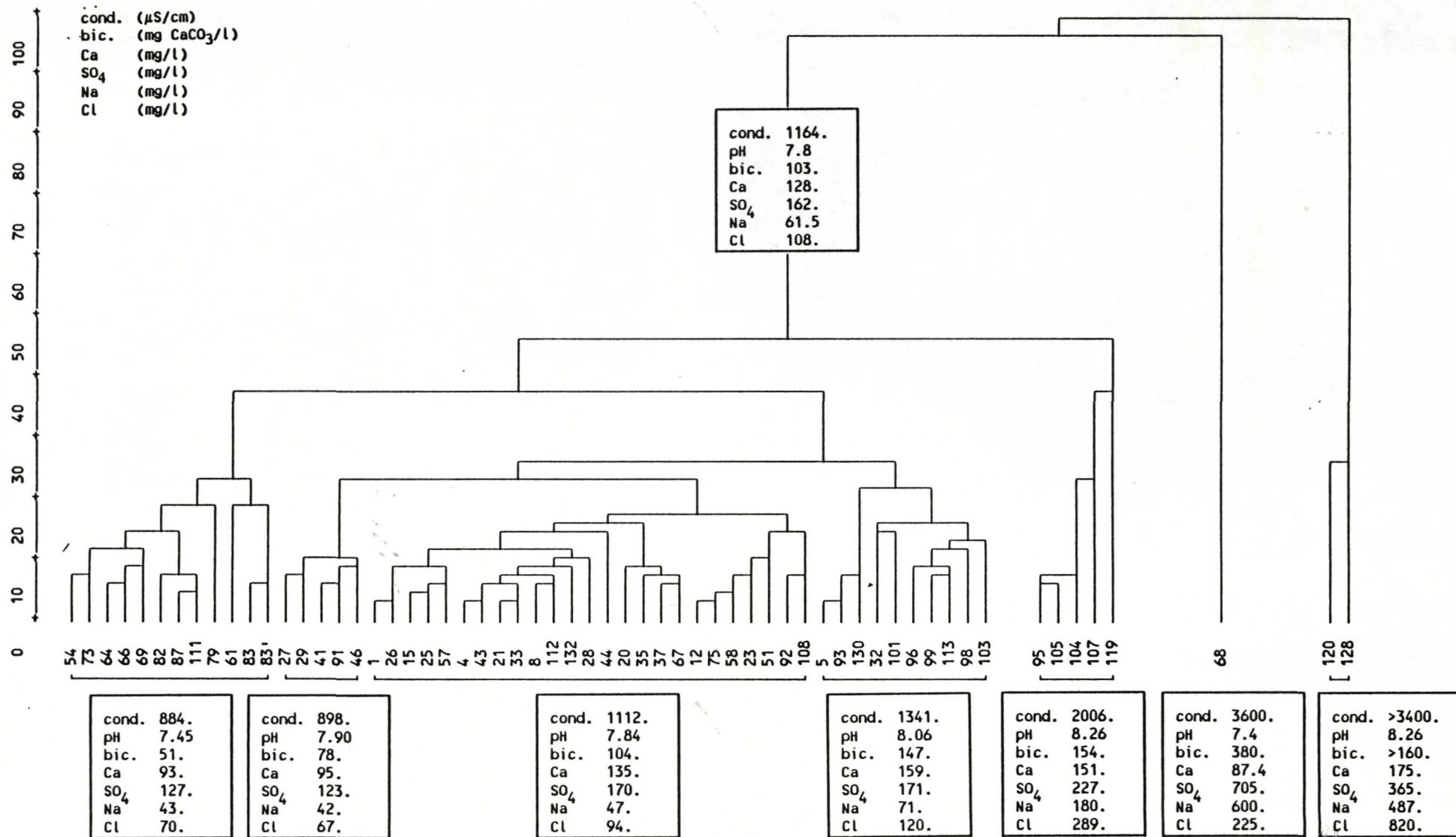
Figuur 3.9 : clusteranalyse van de fysico-chemische gegevens. Voor elke cluster worden de gemiddelde waarden van een aantal variabelen weergegeven.
