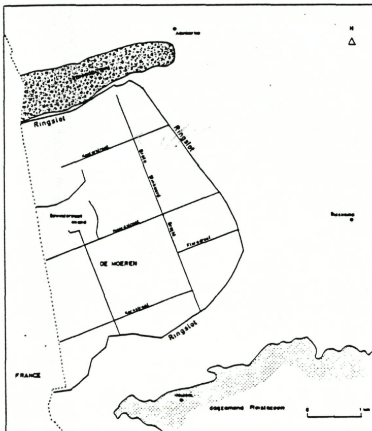
Figuur 1.25 : Kaart van de Moeren (BAETEMAN, 1981).
