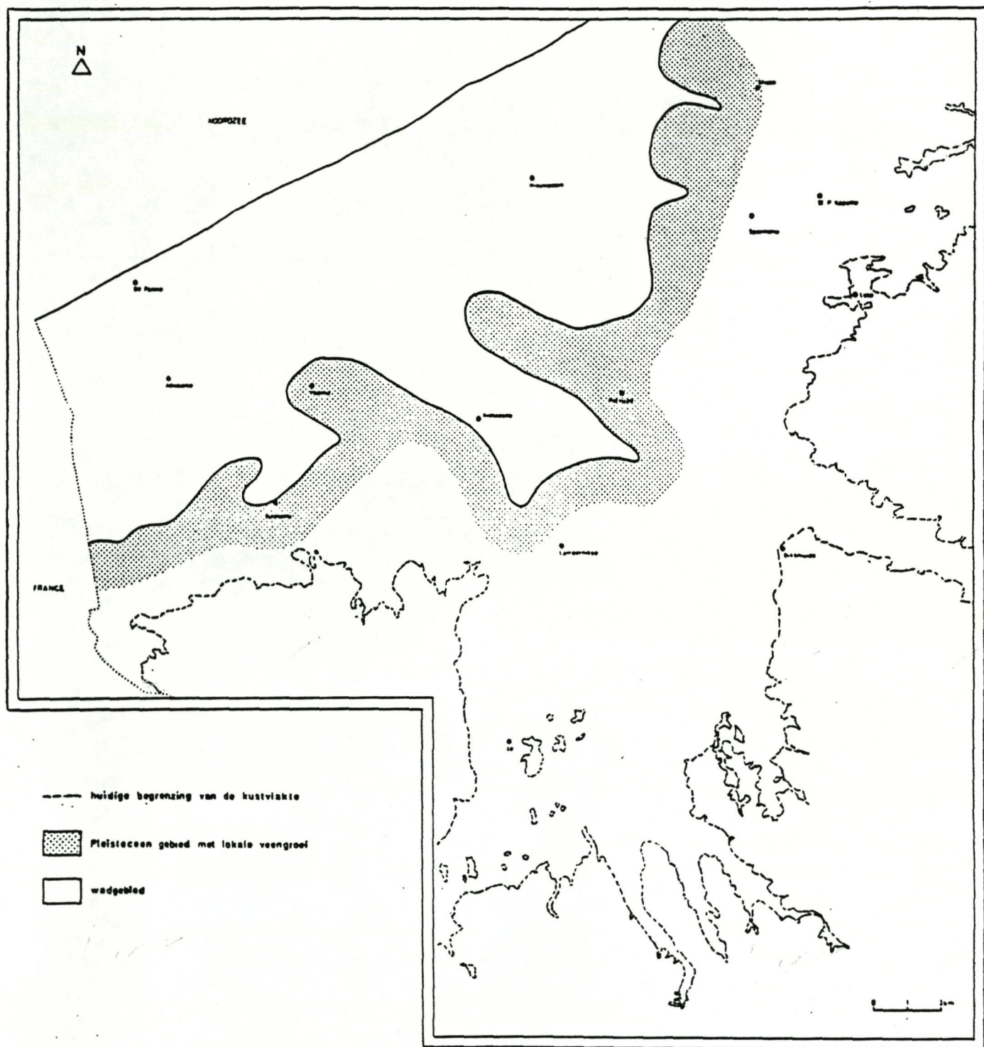
Figuur 1.19a : Paleografie van de kustvlakte omstreeks 5000 v.C. (Baeteman, 1981).
