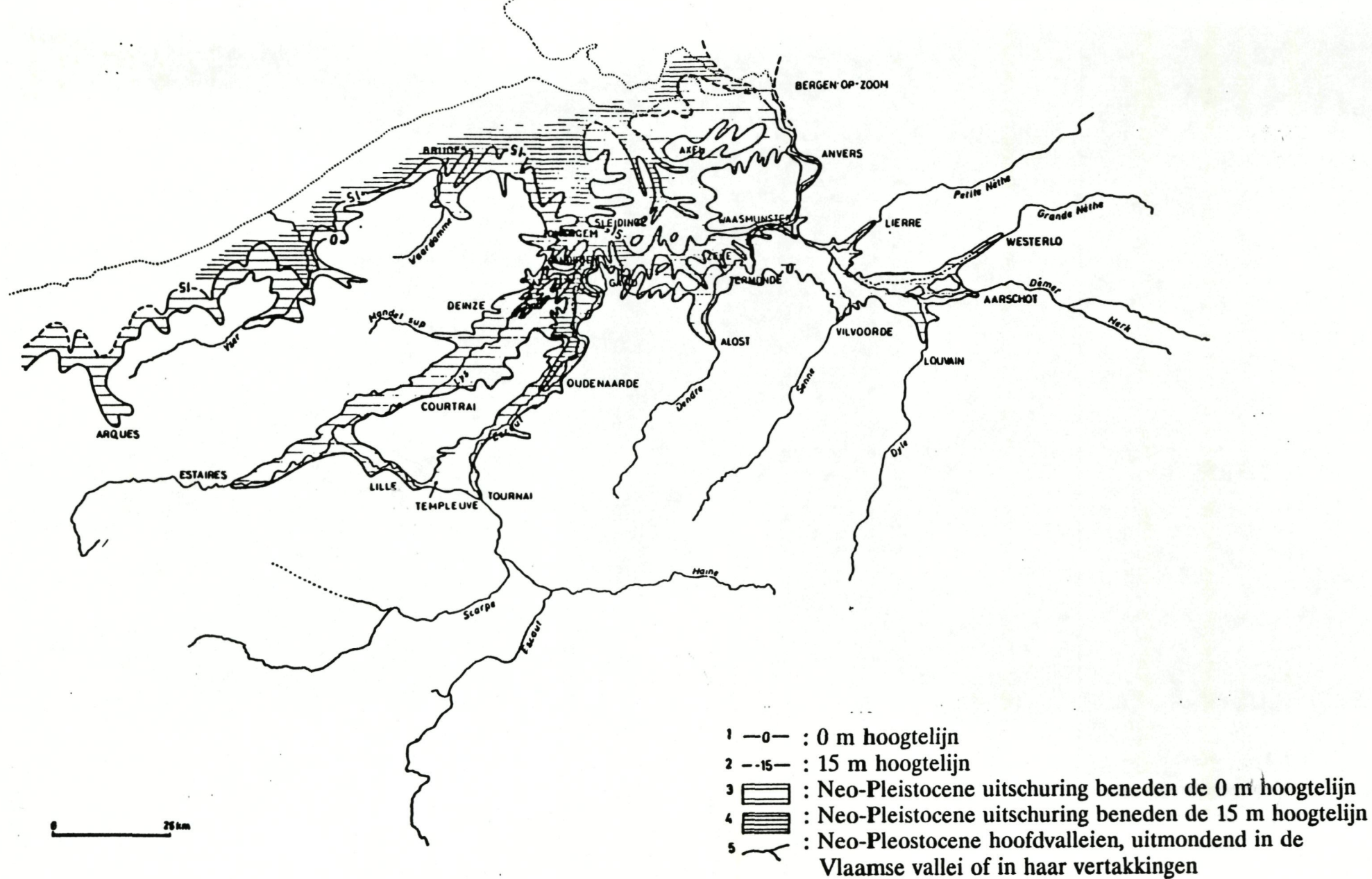
Figuur 1.8 : Het rivierstelsel van het Scheldebekken en de verbreiding van de Vlaamse vallei (TAVERNIER & DE MOOR, 1974).
