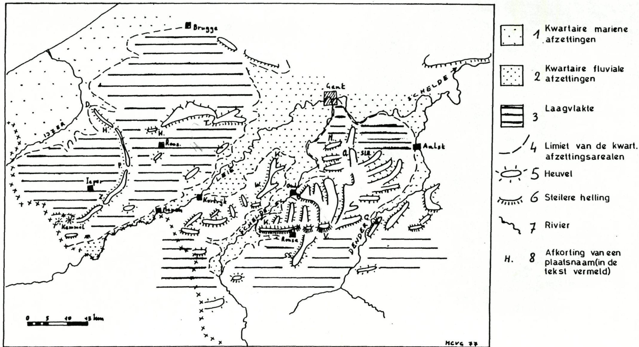
Figuur 1.27 : Het Zuidvlaamse Heuvelland en de omringende depressies (VANMAERKE-GOTTIGNY, 1978).
