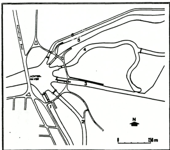
Figuur 1.3 : Het sluizencomplex Ganzepoot te Nieuwpoort (PROVOOST, 1990 - naar DECLERCQ, 1976).
