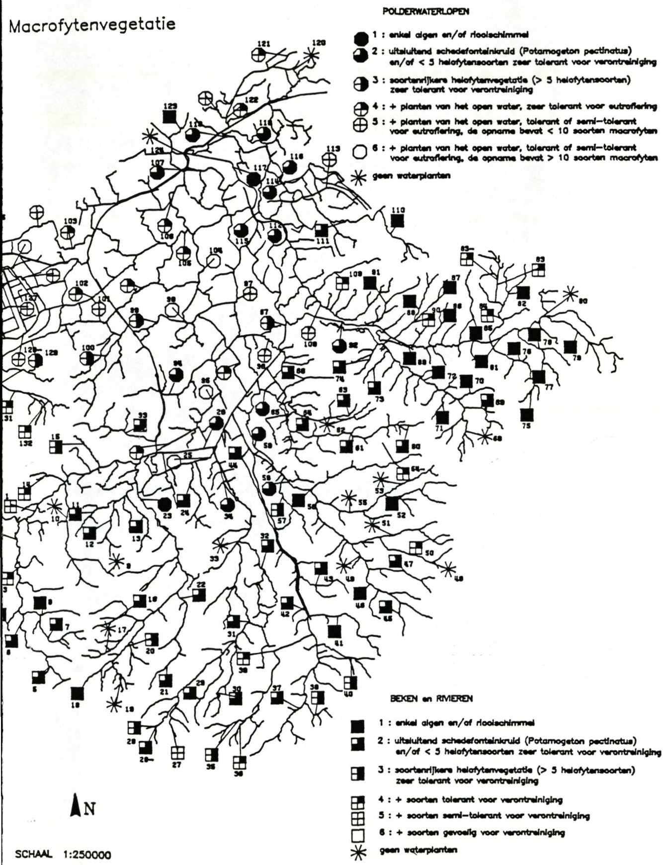
Figuur 2.9 : Beoordeling van de kwaliteit van de waterlopen, gebruik makend van de waterplanten aangetroffen in het IJzerbekken.
