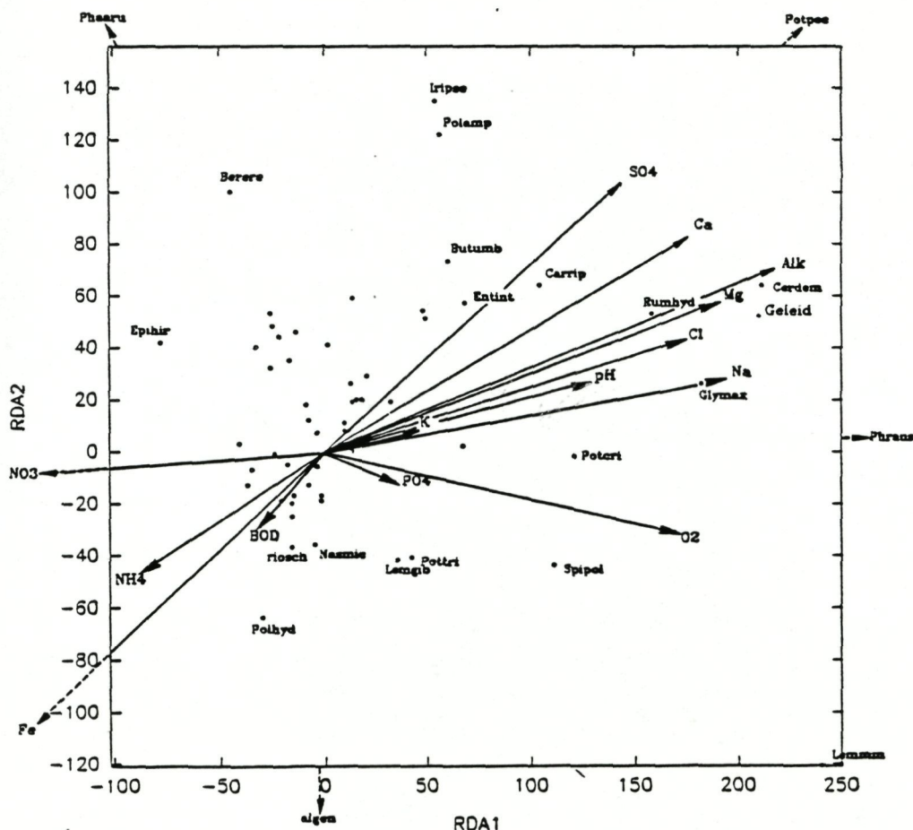
Figuur 3.6 B : Waterplanten en variabelen van de fysico-chemische analyses uitgezet volgens de eerste en de tweede as van de R.D.A.-ordinatie diagram. Enkel de soorten die bepalend zijn voor de samenstelling van de assen zijn weergegeven.
