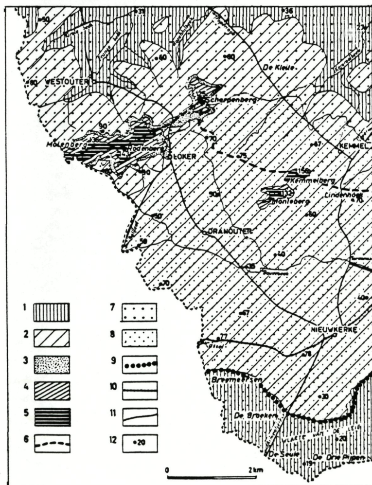
Figuur 1.7 : Vereenvoudigde geologische kaart ter hoogte van de Westvlaamse Heuvels en hun omgeving (HUBERT, 1962c).
