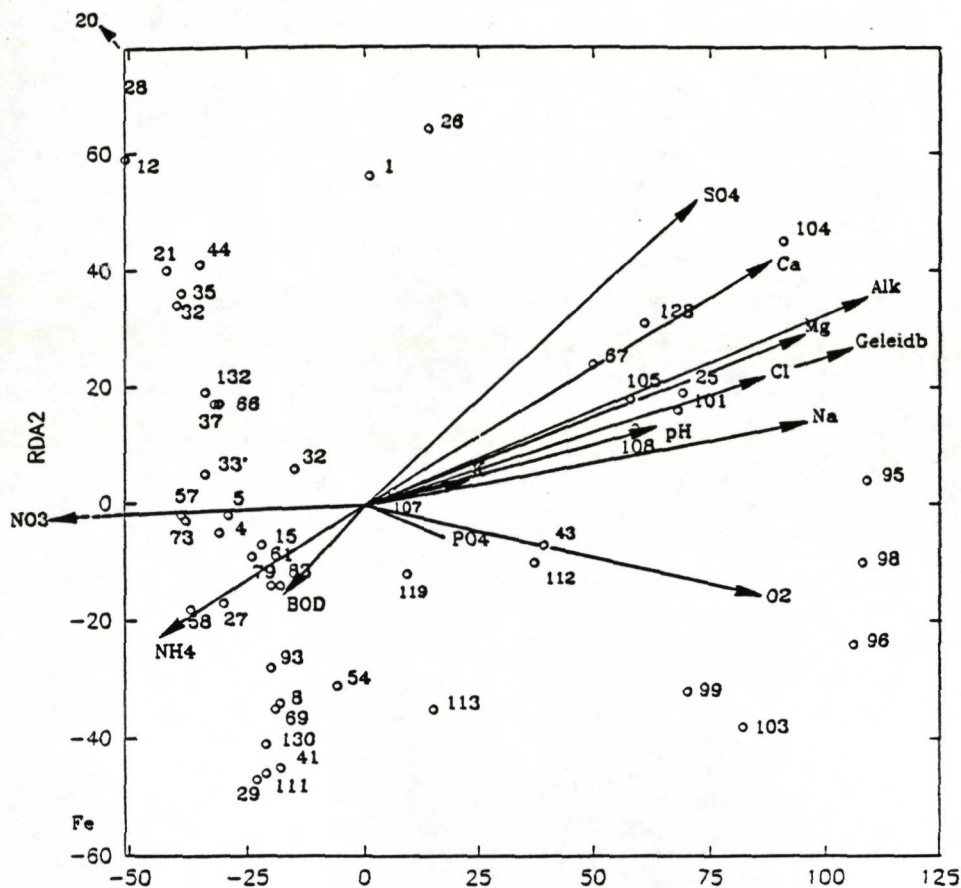
Figuur 3.6 A : Inventarisatiepunten en variabelen van de fysico-chemische analyses uitgezet volgens de eerste en de tweede as van de R.D.A.-ordinatie diagram.
