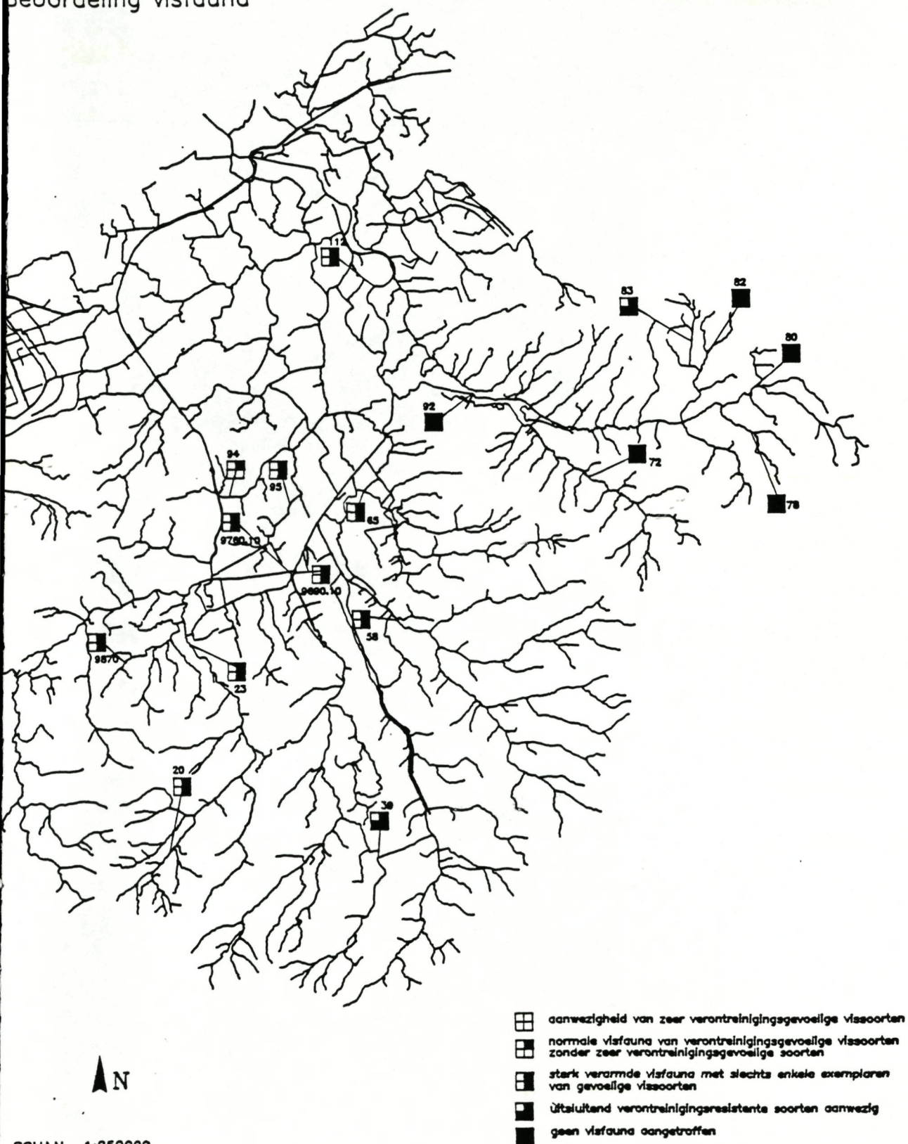
Figuur 2.8 : Overzicht van de visfauna aangetroffen in het IJzerbekken.
