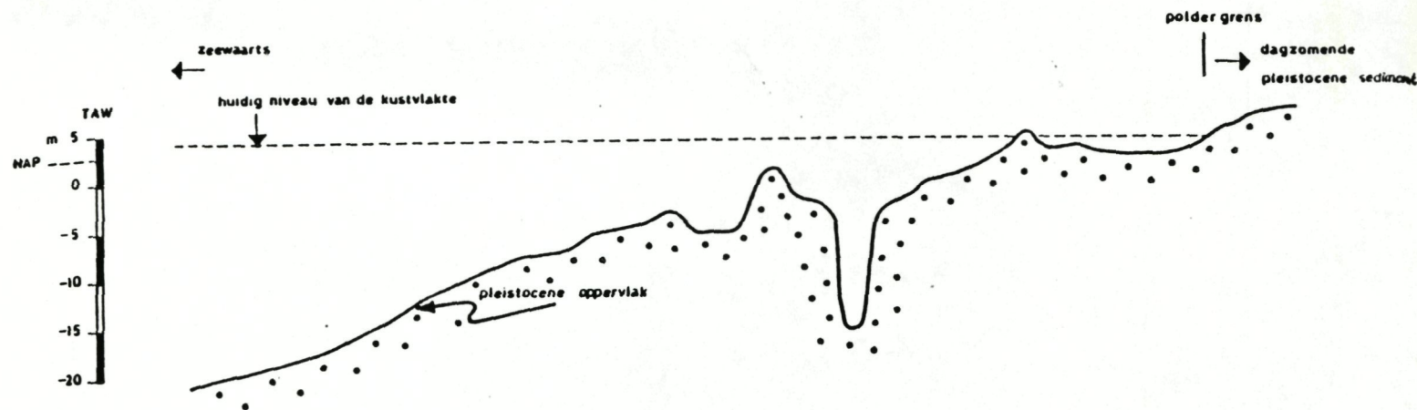
Figuur 1.18a : Schematische voorstelling van het Pleistocene oppervlak (BAETEMAN, 1987).
