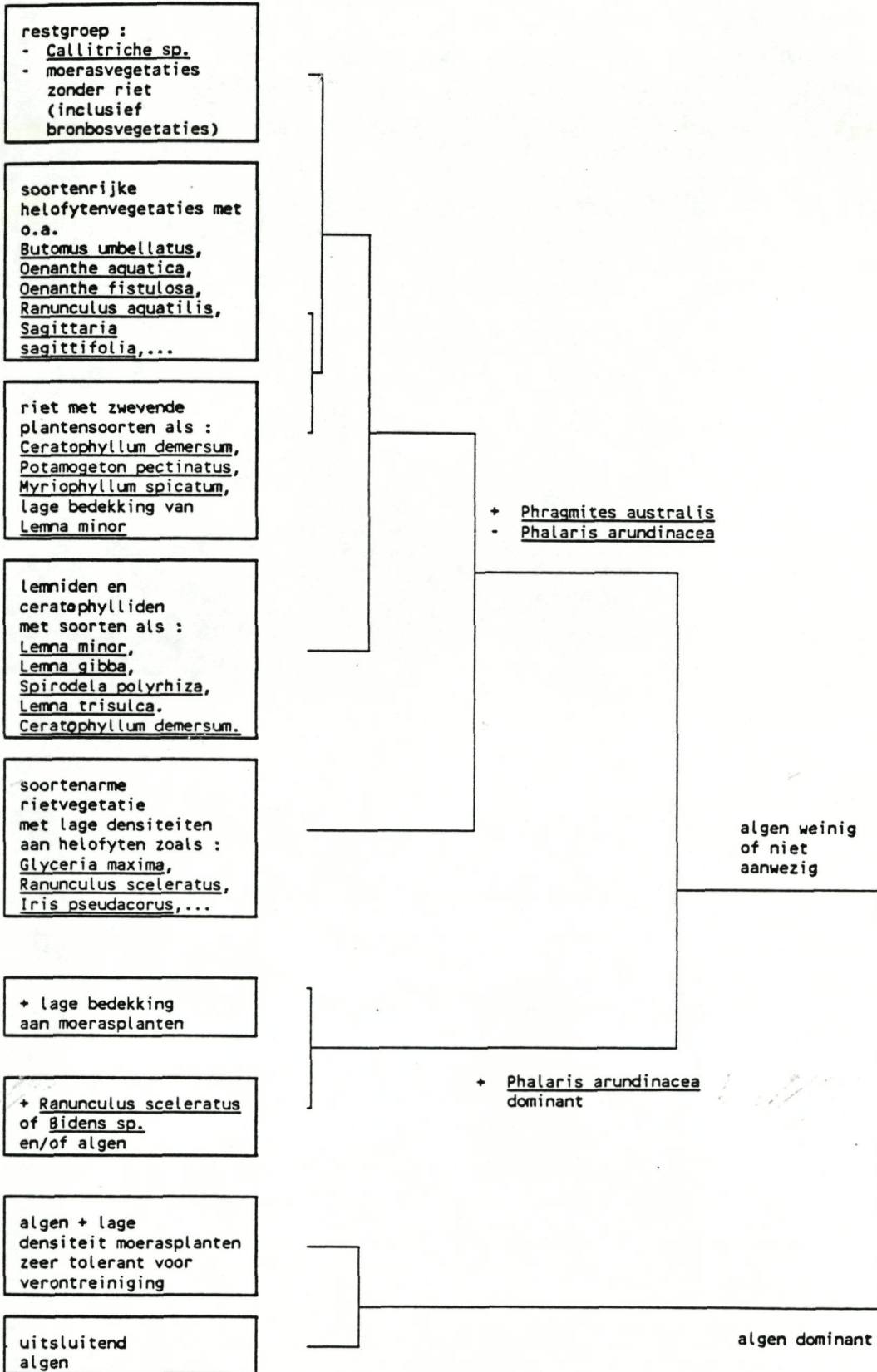
Figuur 3.4 : clusteranalyse van de waterplanten
