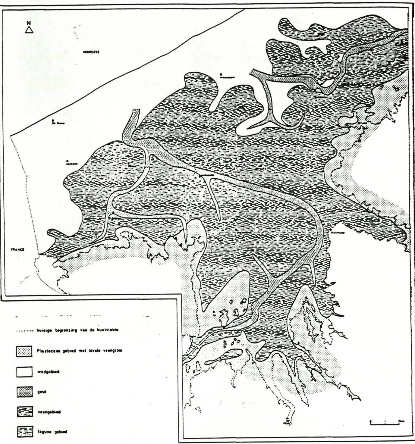
Figuur 1.19d : Paleografie van de kustvlakte omstreeks 2500 v.C. (Baeteman, 1981).
