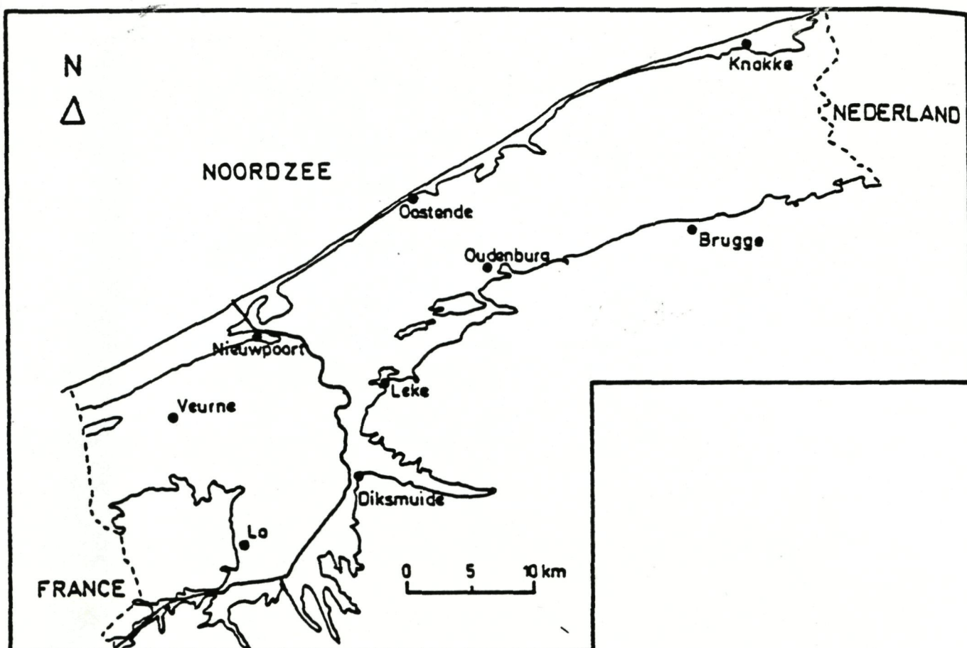
Figuur 1.12 : Kaart van de Belgische kustvlakte (BAETEMAN, 1981).
