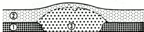
Figuur 1.22 : Veronderstelde ontstaanswijze van een inversiereliëf (TAVERNIER & AMERYCKX, 1970).
