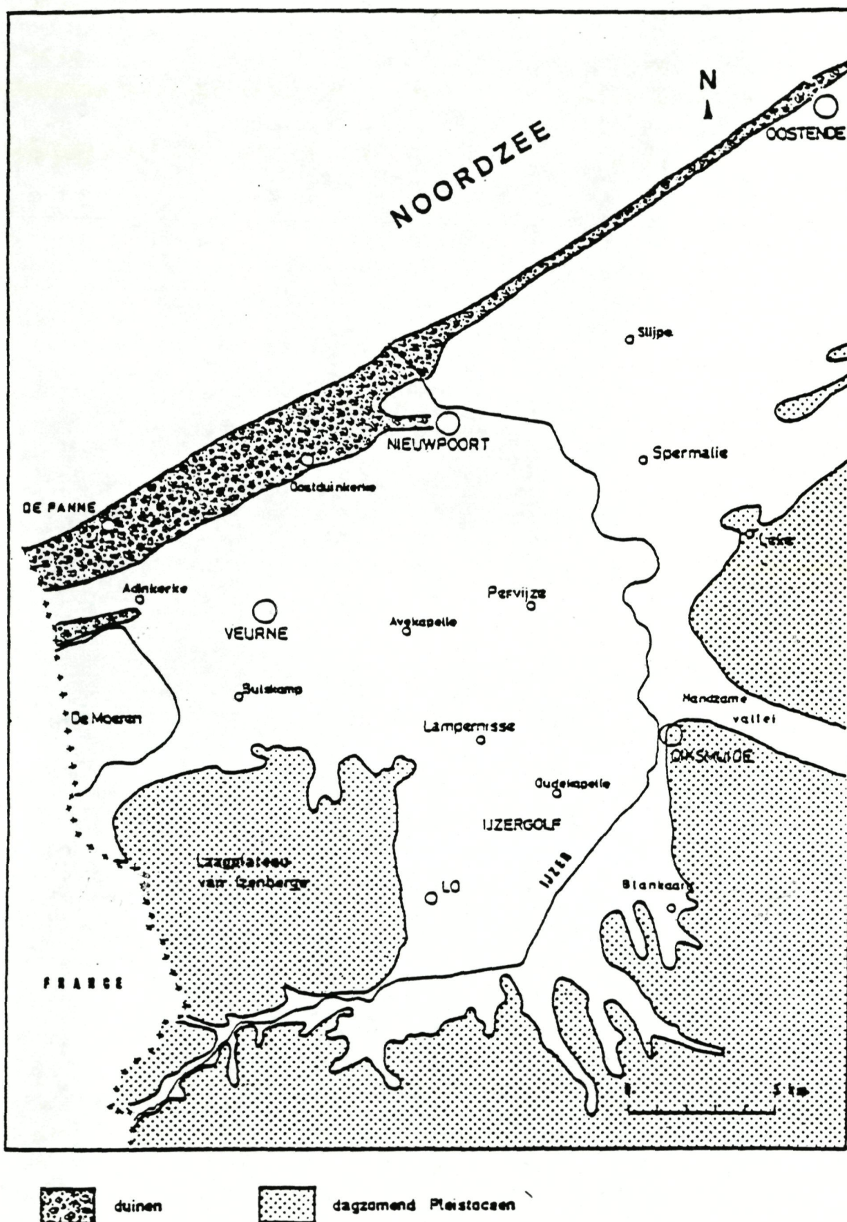
Figuur 1.13 : Begrenzing van de westelijke kustvlakte (BAETEMAN, 1981).
