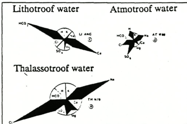
Figuur 1.31 : Maucha-diagrammen van een aantal watertypen in het studiegebied
