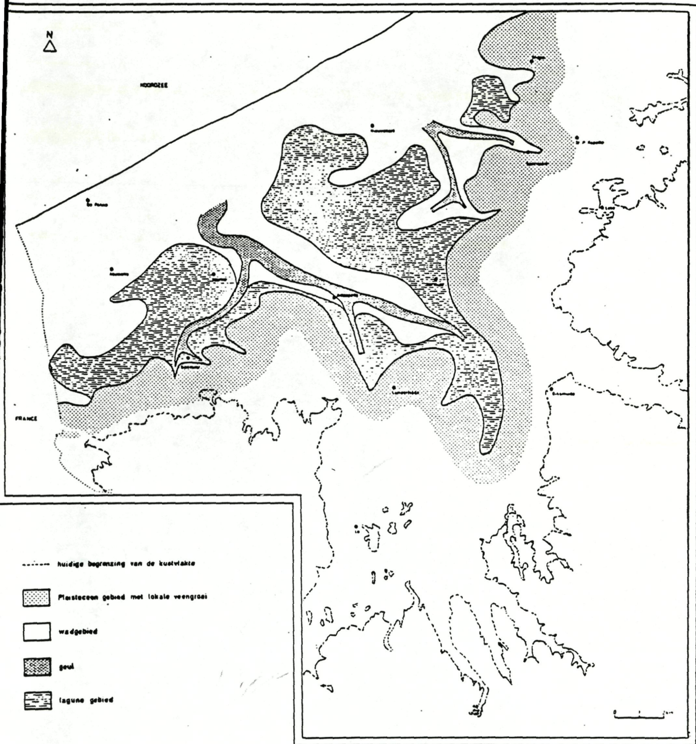
Figuur 1.19b : Paleografie van de kustvlakte omstreeks 4500 v.C. (Baeteman, 1981) .
