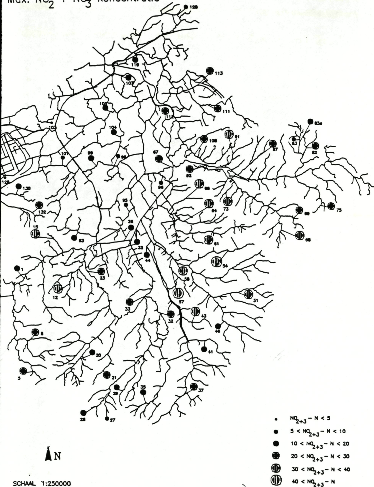
Figuur 2.4 : Overzicht van de maximaal gemeten nitraat- + nitrietconcentraties in het IJzerbekken
