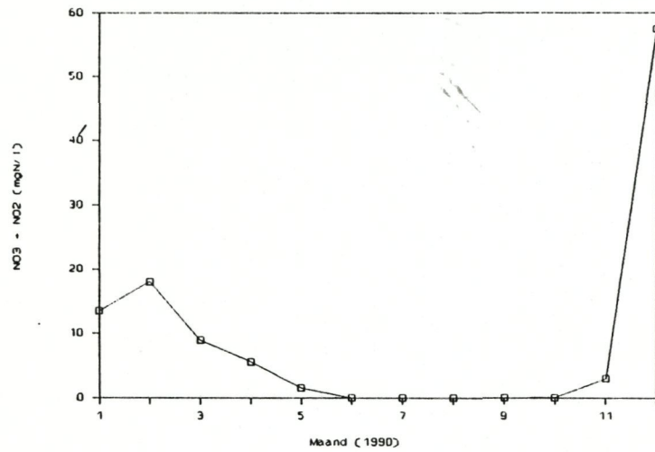
Figuur 2.5 : Verloop van de nitraat- en nitrietconcentraties gedurende 1990 (gegevens V.M.M.)
