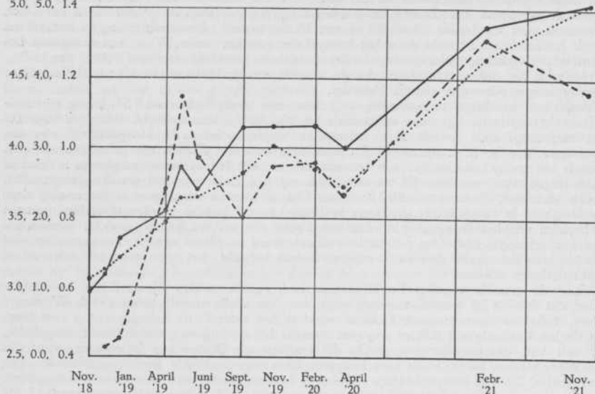
Fig. 2. Groei van mossels in de Wieringer Meer, lengte (getrokken lijn, cijfers links); vleeschgewicht (onderbroken lijn, cijfers rechts); schelpgewicht (stippelij, middenste cijfers).
