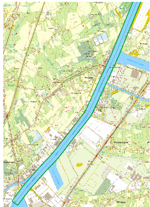
Figuur 10.7 Plaatsgebonden risico. Weergegeven is de ligging van de PR 10 -7 contour (blauw), de PR 10 -8 contour (groen)
