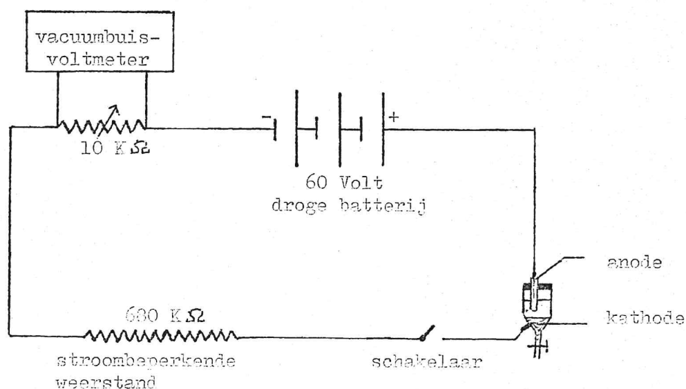
Fig. 2 : Schakelschema gebruikt bij het iken van de IMT-onlossingen. (gewijzigd naar PACKARD & FRANK 1958).
