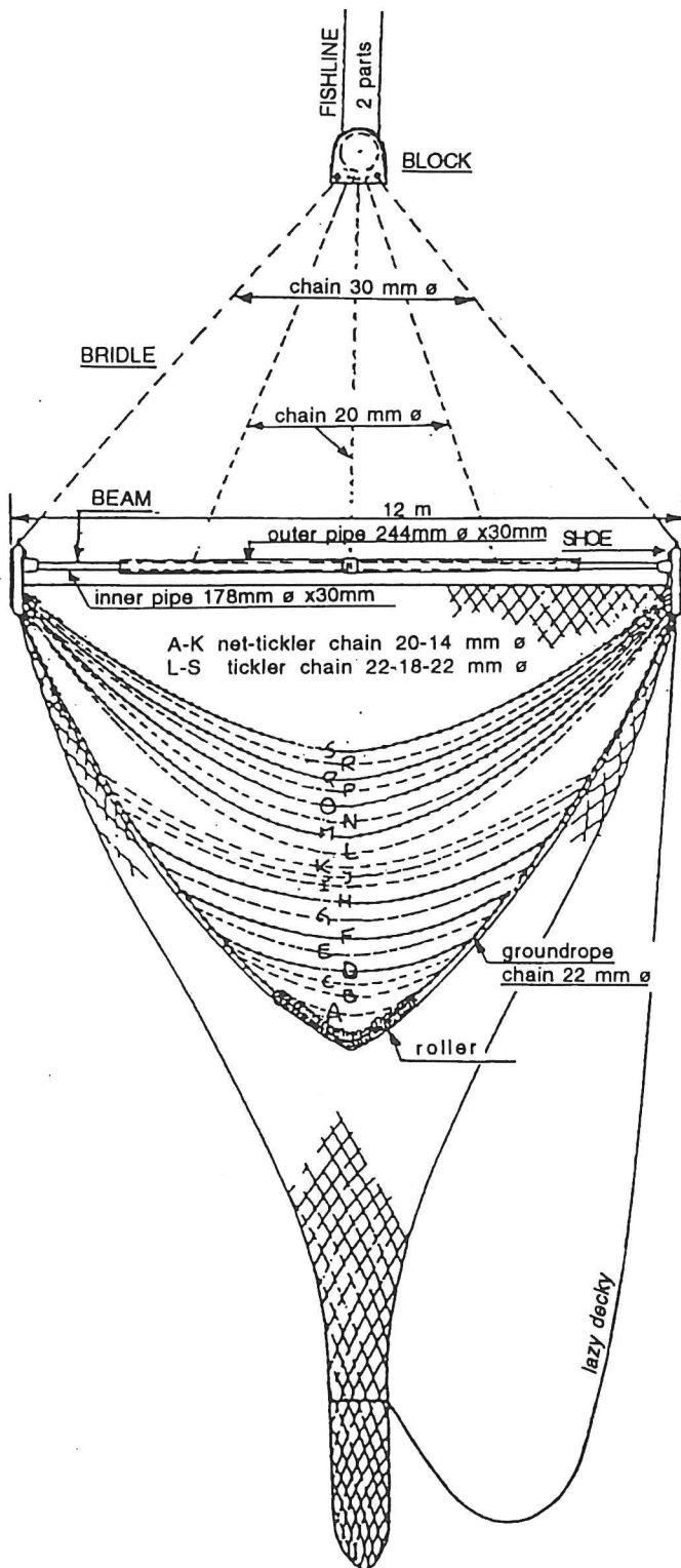
Fig. 3a. Beamtrawl-gear
