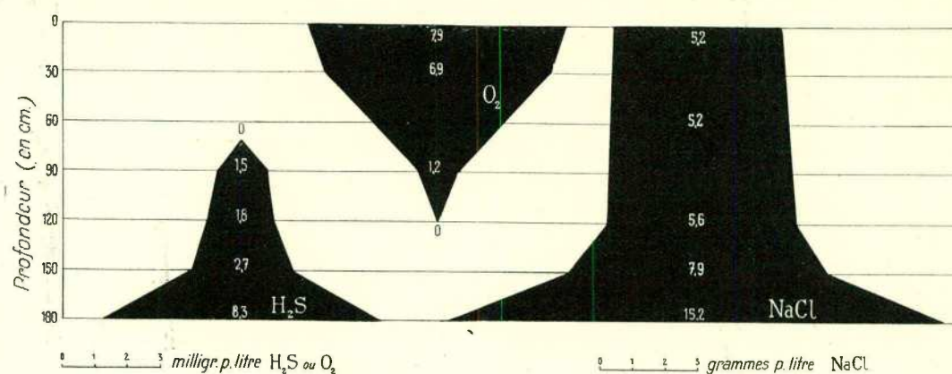
FIG. 14. — Variations verticales de H_2S , O_2 et de la salinité.
