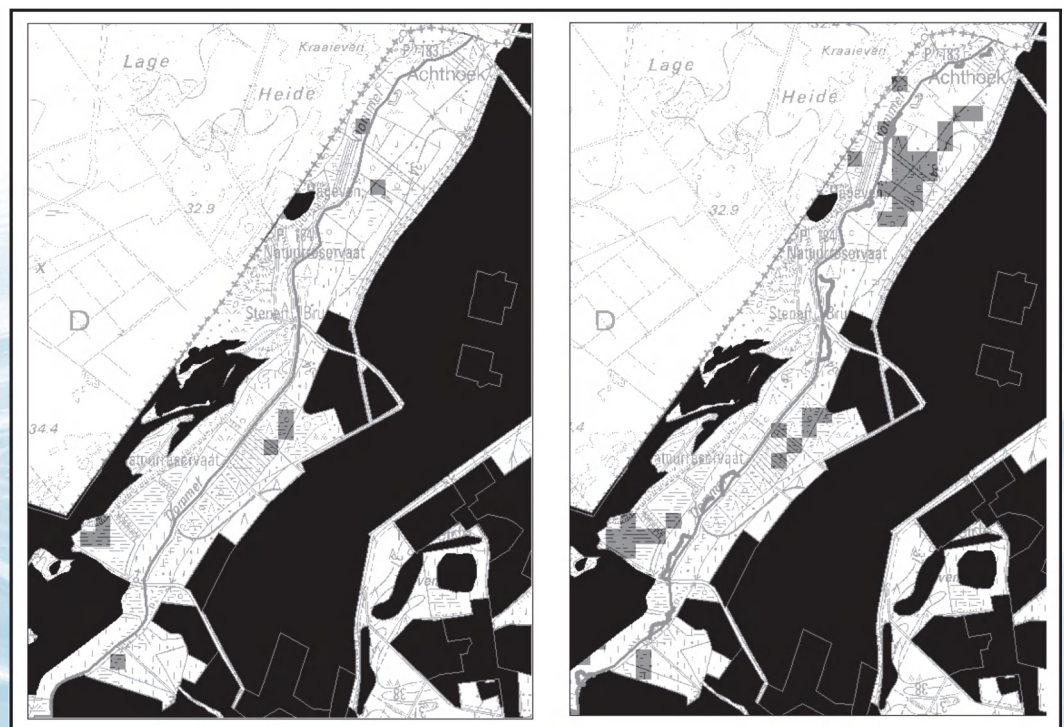
Figuur 2: Potentieel voorkomen van grote zeggenvegetaties met riet in huidige toestand (links) en na herneandering (rechts). De voorspelling zijn weergegeven als donkergrijze blokjes, de zwarte polygonen zijn locaties waarvoor NICHE geen uitspraak doet (zoals landbouwgronden, antropogene gronden, enz.) De Dommel al dan niet met meanders is weergegeven als lichtgrijze polyline.
